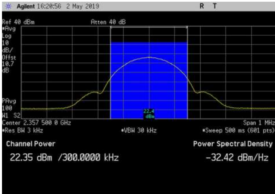
DL_2350-2360_GSM_2357.5MHz_3dB
