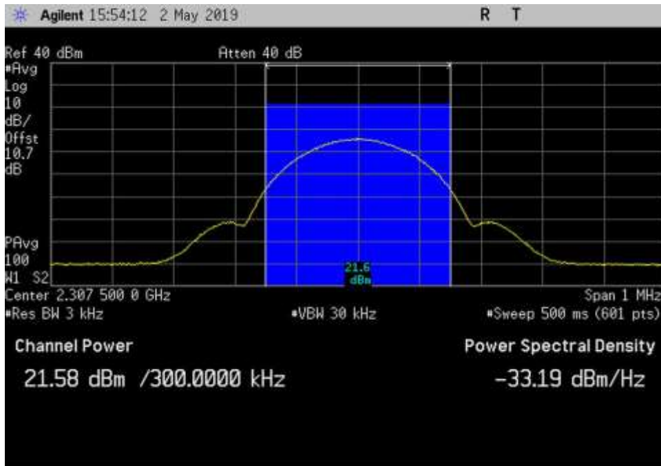
UL_2305-2315_GSM_2307.5MHz_3dB
