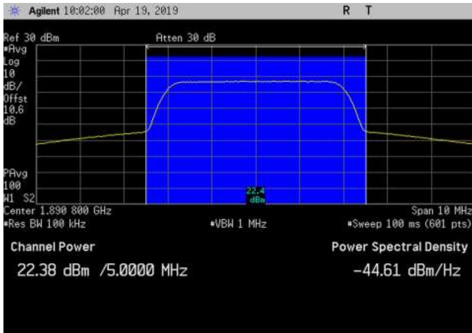
UL_1850-1915_AWGN_1890.8MHz_3dB
