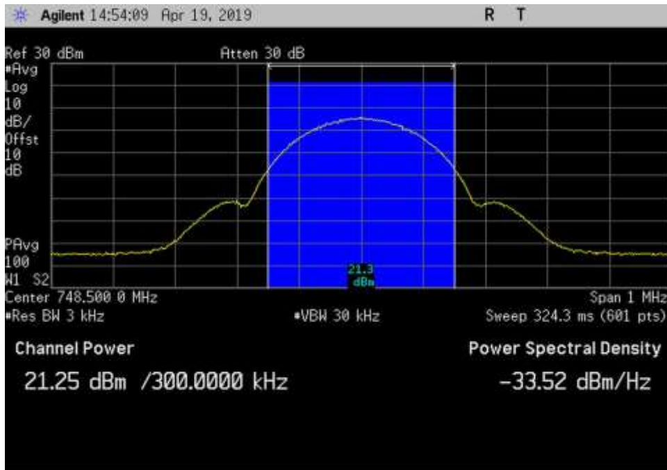
DL_746-757_GSM_748.5MHz_3dB
