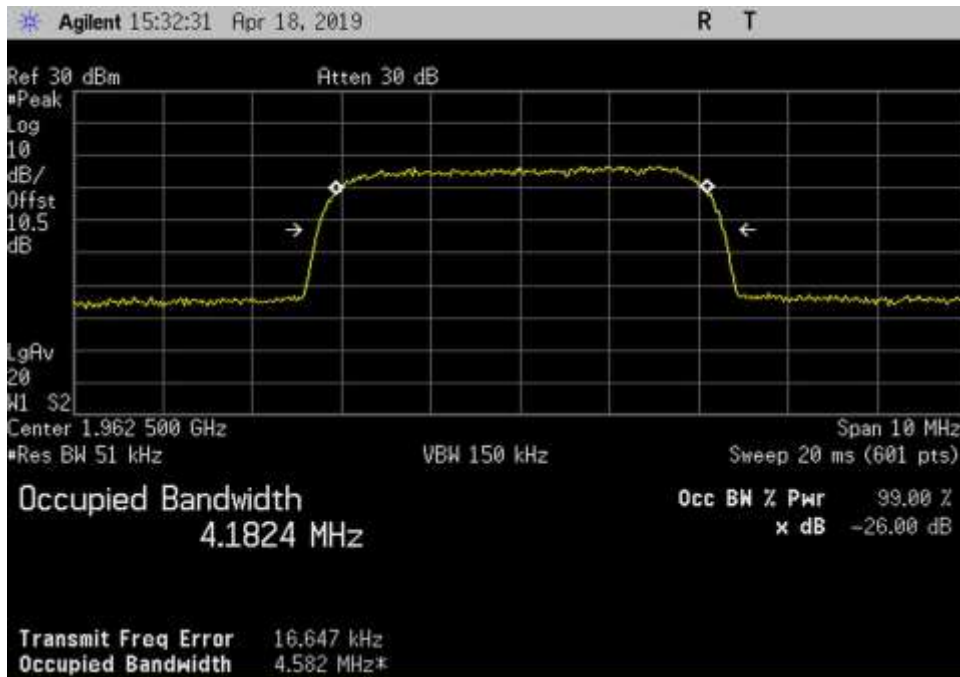
Out_DL_1930-1995_WCDMA_1962.5MHz
