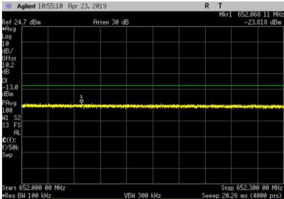
DL_617-652_AWGN_ 652- 652.3MHz_Cm-H+3dB
