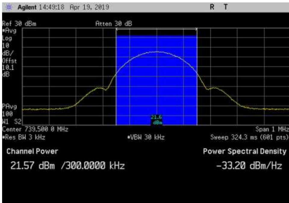
DL_728-746_GSM_739.5MHz_3dB
