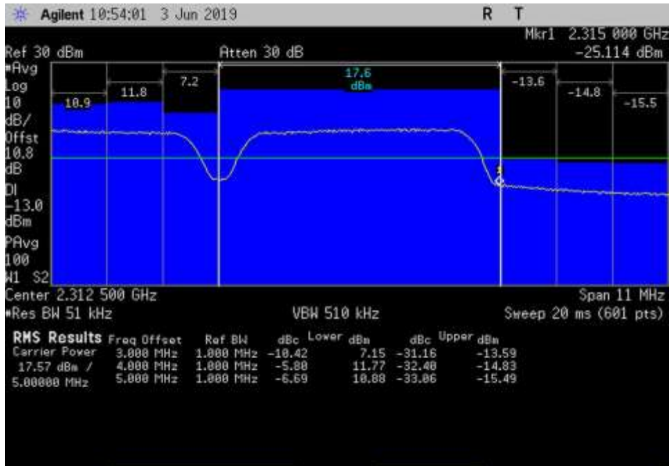
UL_2305-2315_AWGN_ 2315- 2318MHz_Cm-H+3dB
