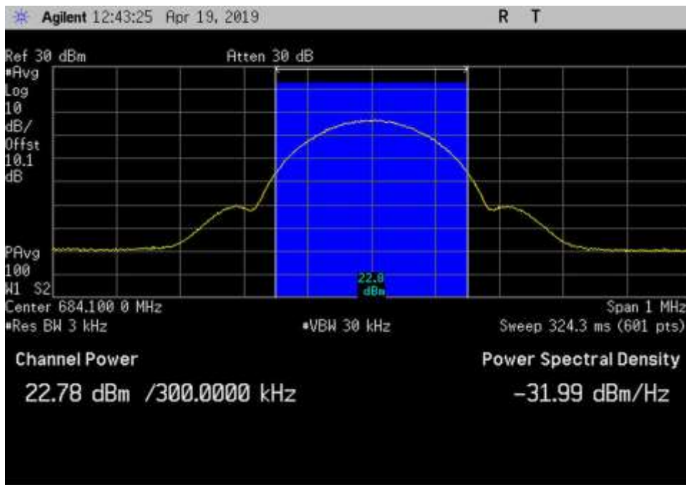
UL_663-698_GSM_684.1MHz_3dB
