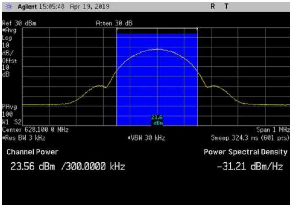
DL_617-652_GSM_628.1MHz_3dB
