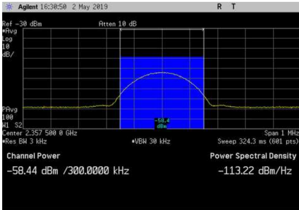
DL_2350-2360_GSM_2357.5MHz_Input
