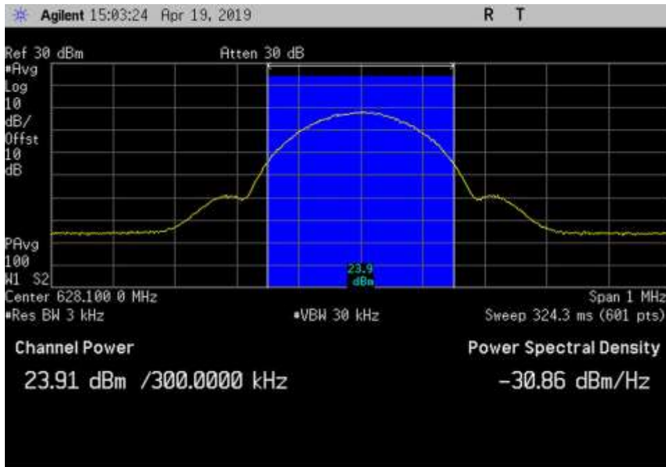
DL_617-652_GSM_628.1MHz
