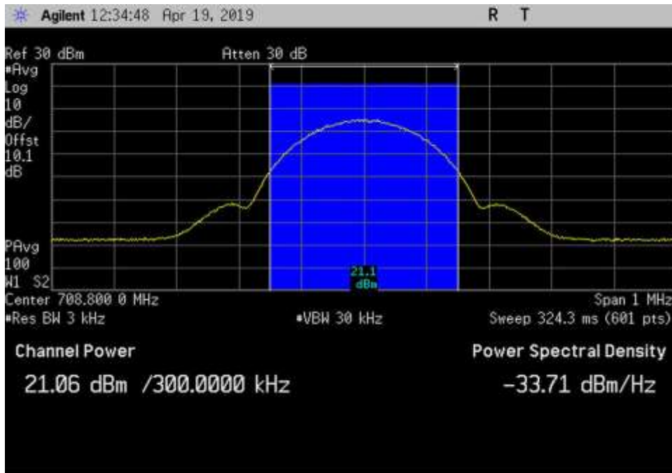
UL_698-716_GSM_708.8MHz
