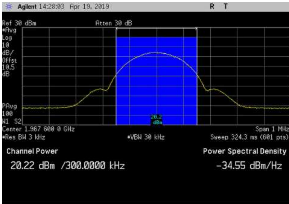
DL_1930-1995_GSM_1967.6MHz_3dB
