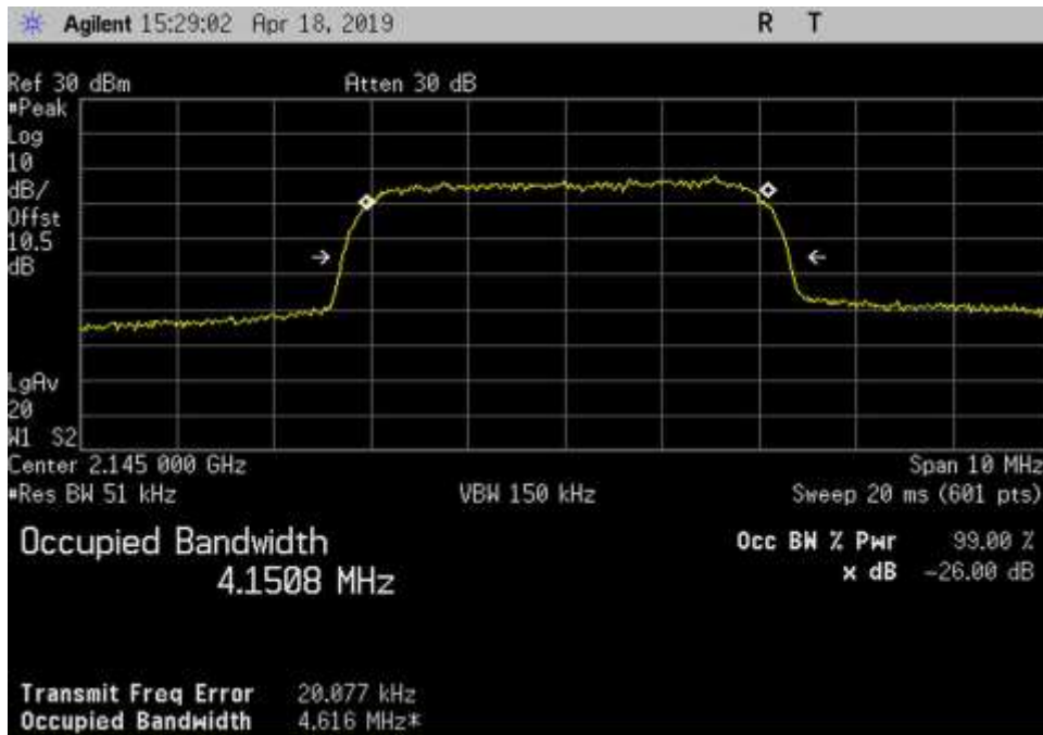
Out_DL_2110-2155_WCDMA_2145MHz
