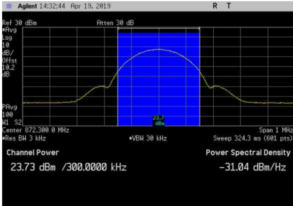
DL_869-894_GSM_ 872.3MHz
