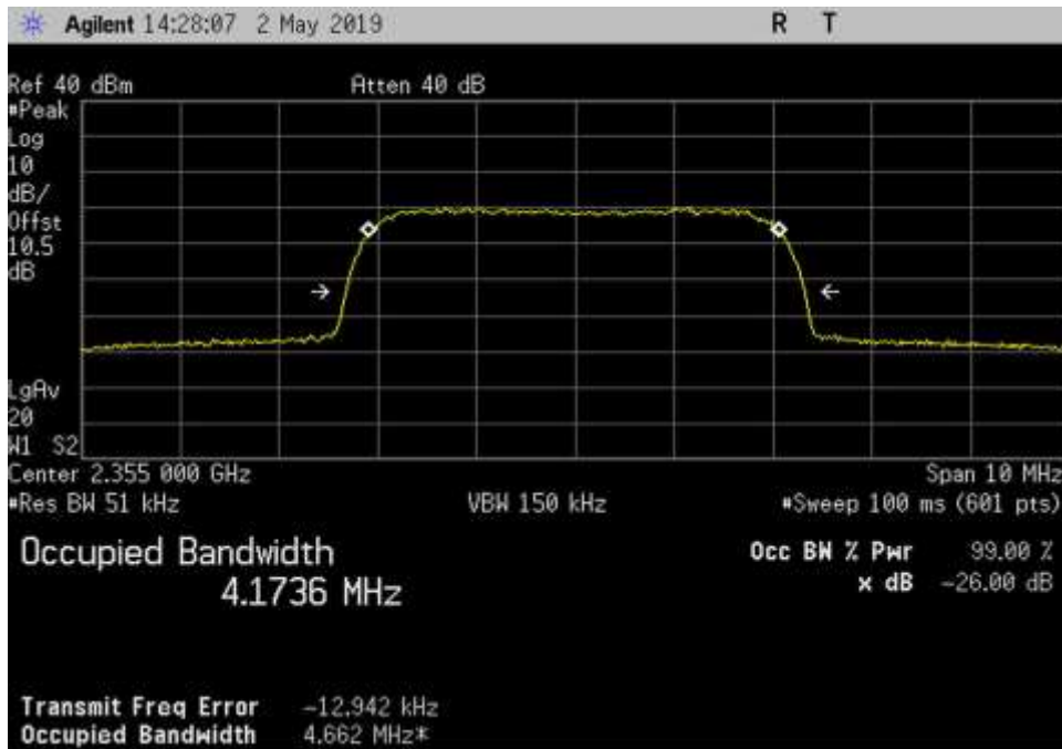
Out_DL_2350-2360_WCDMA_2355MHz
