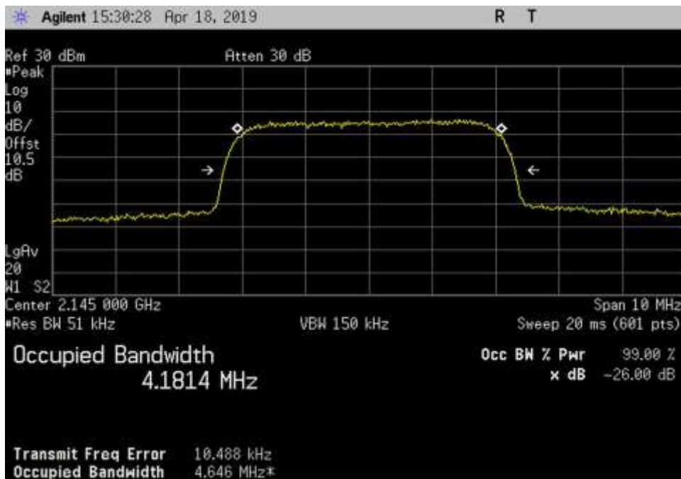
Out_DL_2110-2155_WCDMA_2145MHz_3dB
