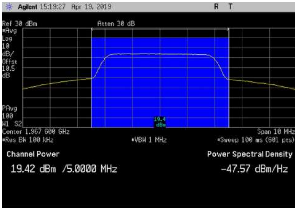
DL_1930-1995_AWGN_1967.6MHz_3dB
