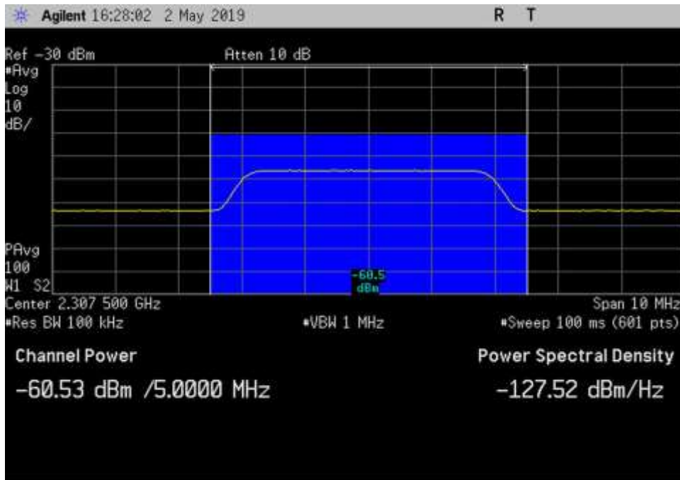
UL_2305-2315_AWGN_2307.5MHz_Input
