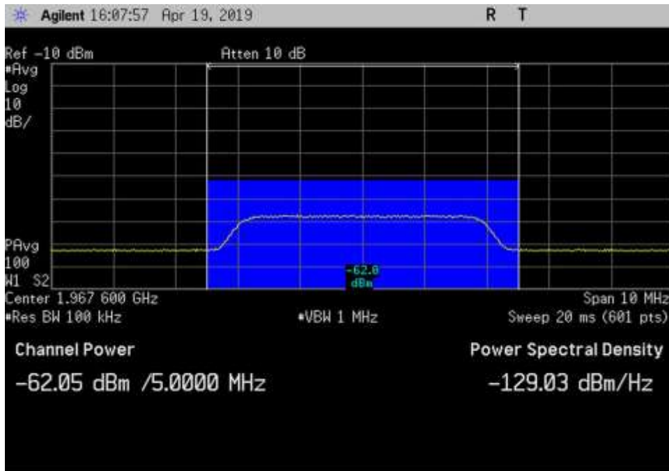
DL_1930-1995_AWGN_1967.6MHz_Input
