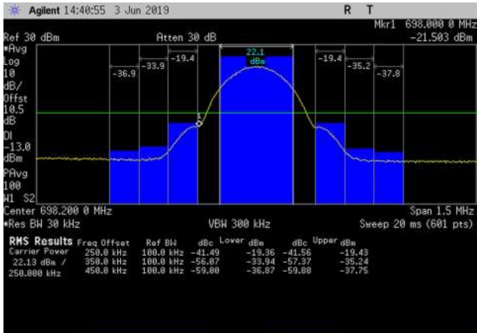
UL_698-716_GSM_697.7- 698MHz_Sn-L+3dB
