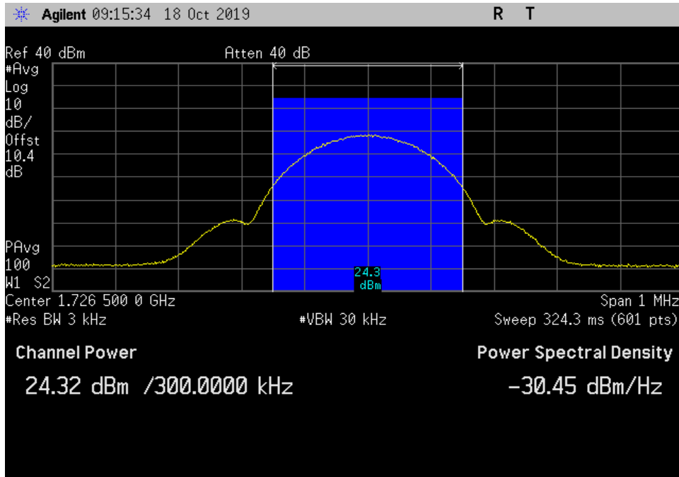
UL_1710-1755_GSM_1726.5MHz
