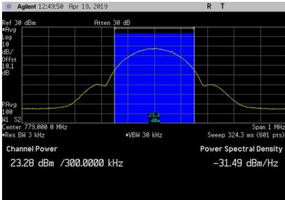
UL_776-787_GSM_779MHz_3dB
