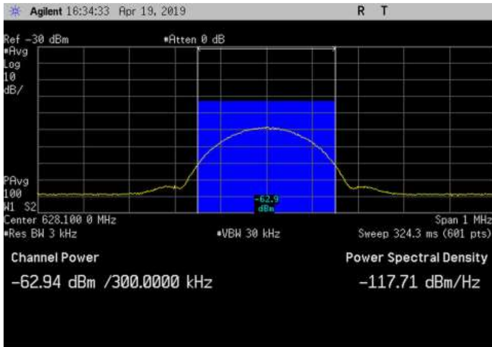
DL_617-652_GSM_628.1MHz_Input
