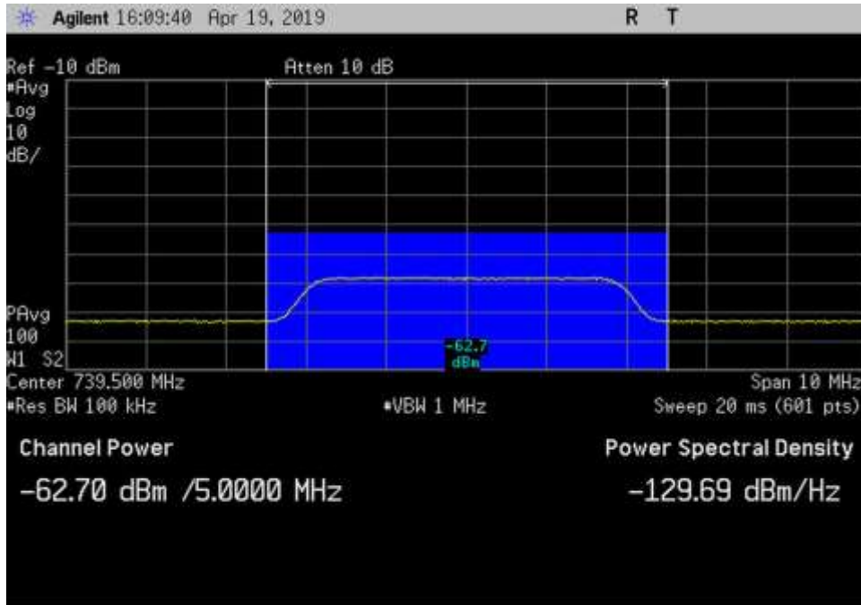
DL_728-746_AWGN_ 739.5MHz_Input
