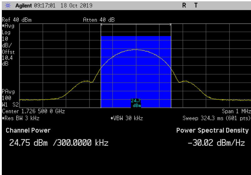
UL_1710-1755_GSM_1726.5MHz_3dB
