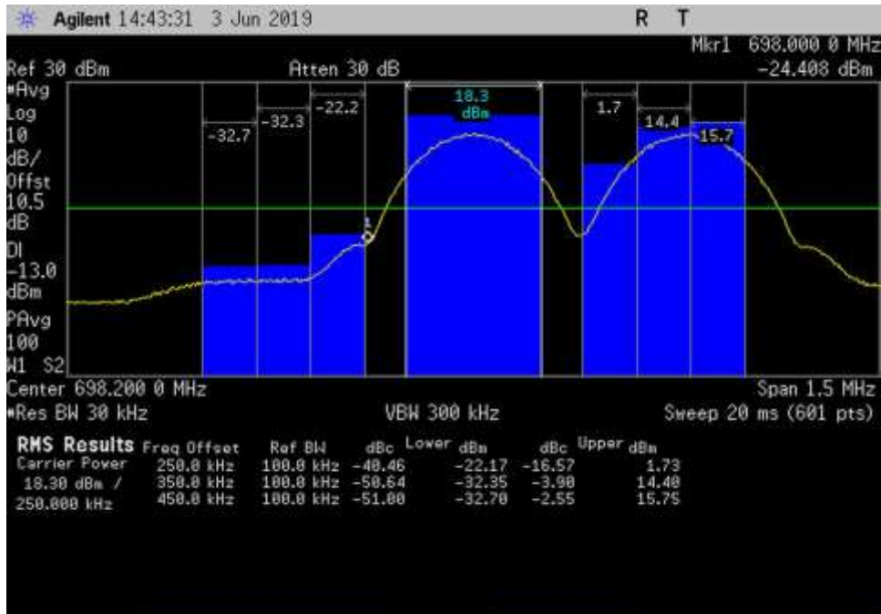
UL_698-716_GSM_697.7-698MHz_Cm-L+3dB
