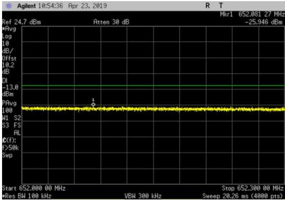
DL_617-652_AWGN_ 652- 652.3MHz_Cm-H
