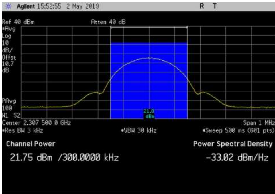
UL_2305-2315_GSM_2307.5MHz
