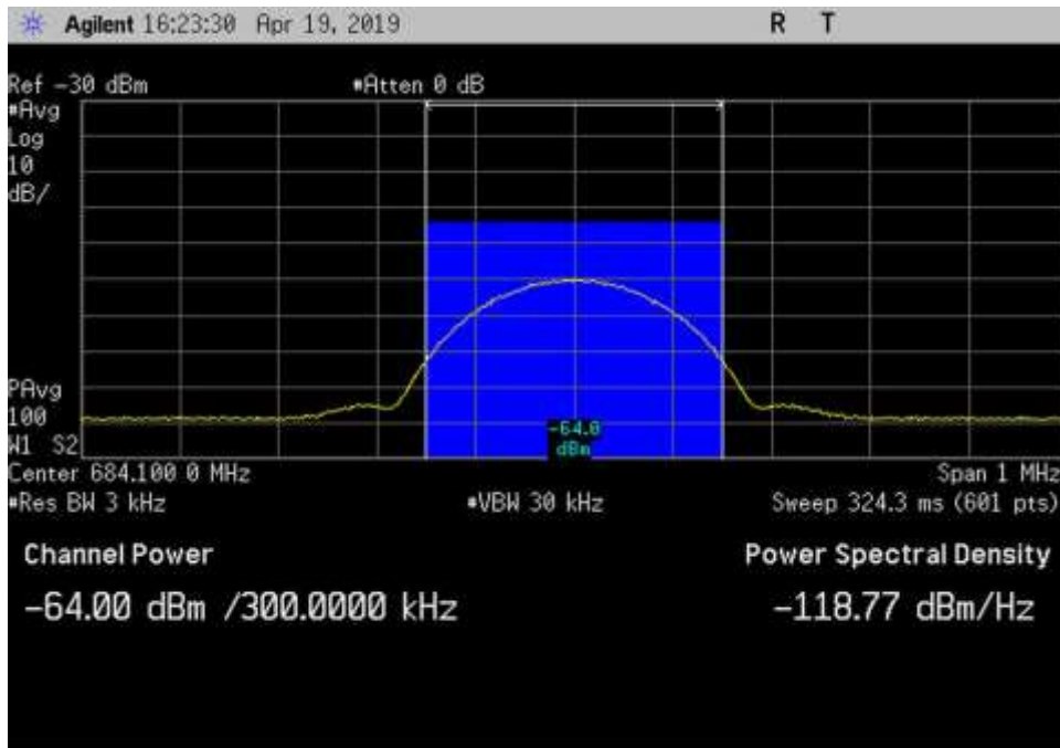
UL_663-698_GSM_684.1MHz_Input
