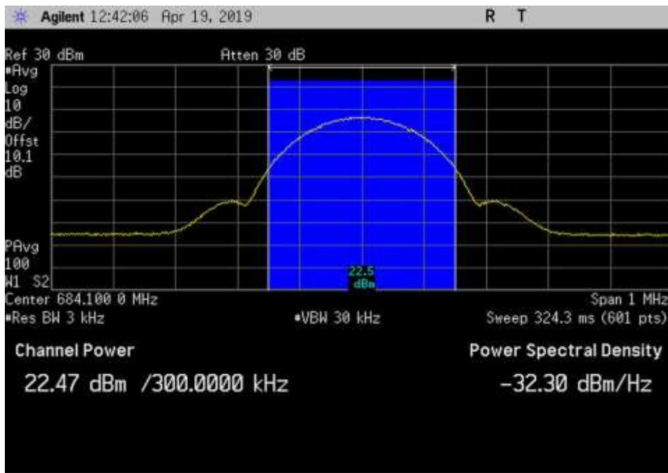
UL_663-698_GSM_684.1MHz
