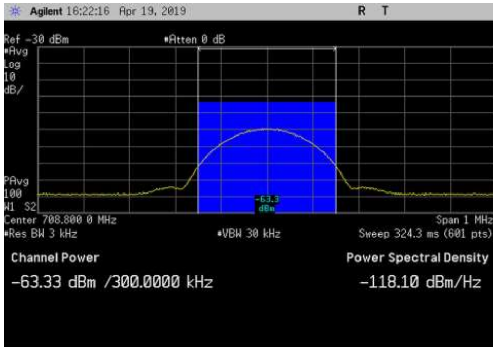
UL_698-716_GSM_708.8MHz_Input
