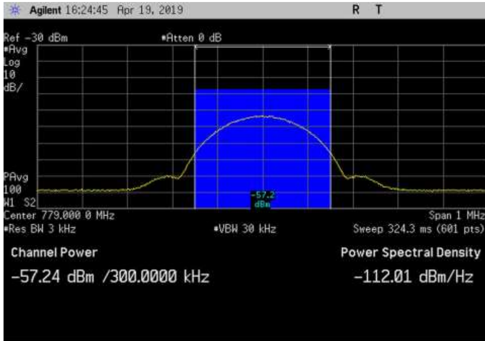
UL_776-787_GSM_779MHz_Input
