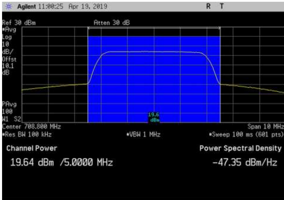
UL_698-716_AWGN_708.8MHz_3dB
