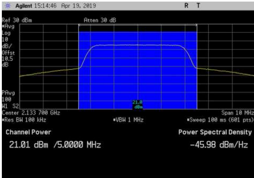
DL_2110-2155_AWGN_2133.7MHz_3dB
