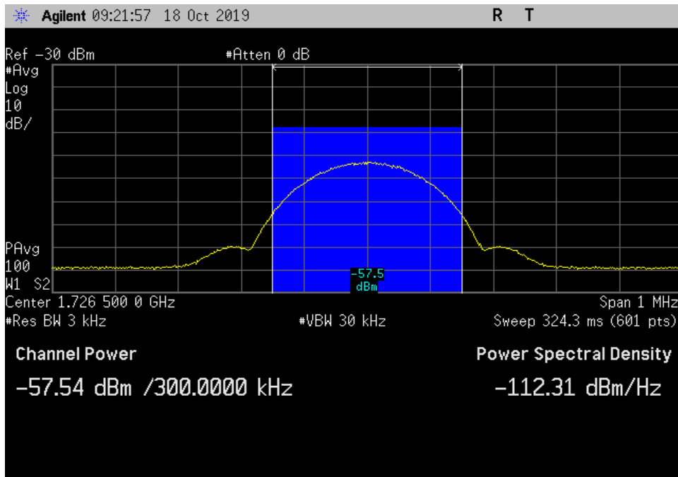
UL_1710-1755_GSM_1726.5MHz_Input
