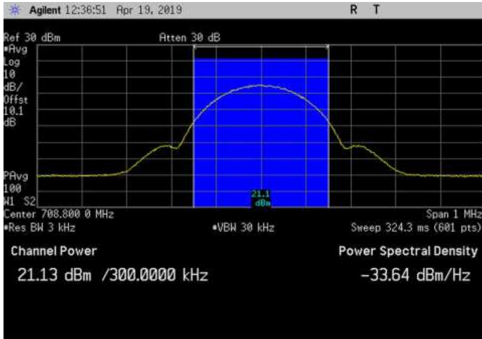
UL_698-716_GSM_708.8MHz_3dB
