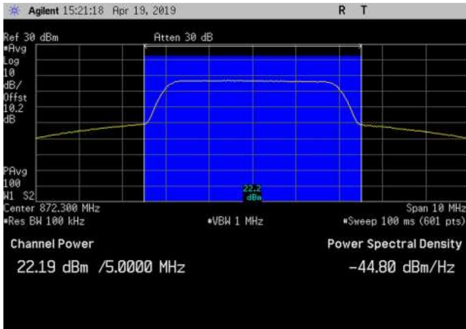
DL_869-894_AWGN_ 872.3MHz.
