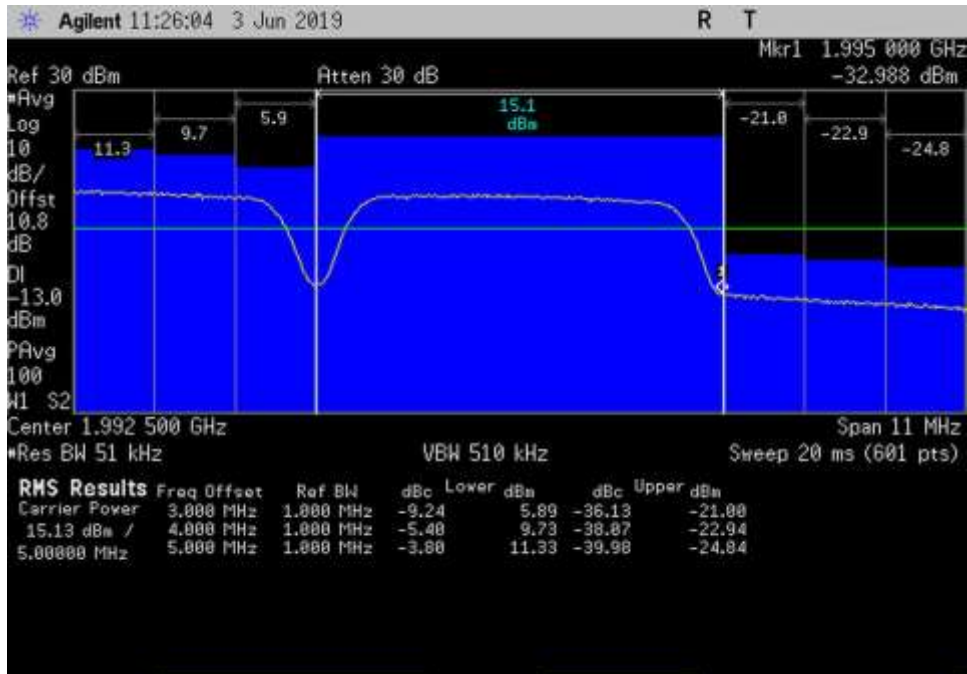
DL_1930-1995_AWGN_1995-1998MHz_Cm-H+3dB
