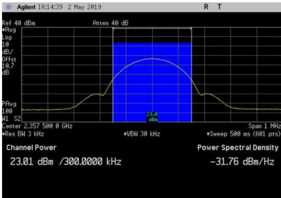
DL_2350-2360_GSM_2357.5MHz
