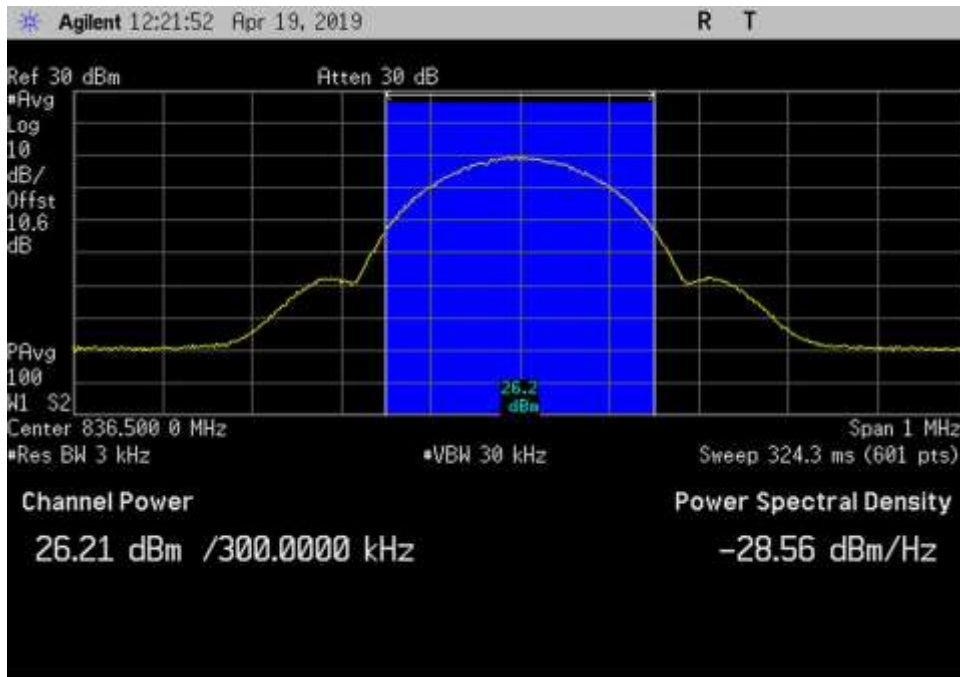
UL_824-849_GSM_836.5MHz_3dB
