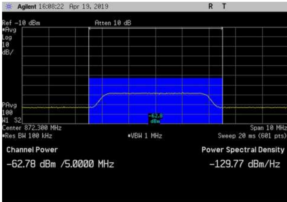
DL_869-894_AWGN_872.3MHz_Input
