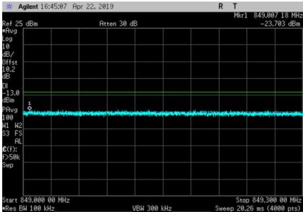
UL_824-849_AWGN_849-849.3MHz_Cm-H+3dB
