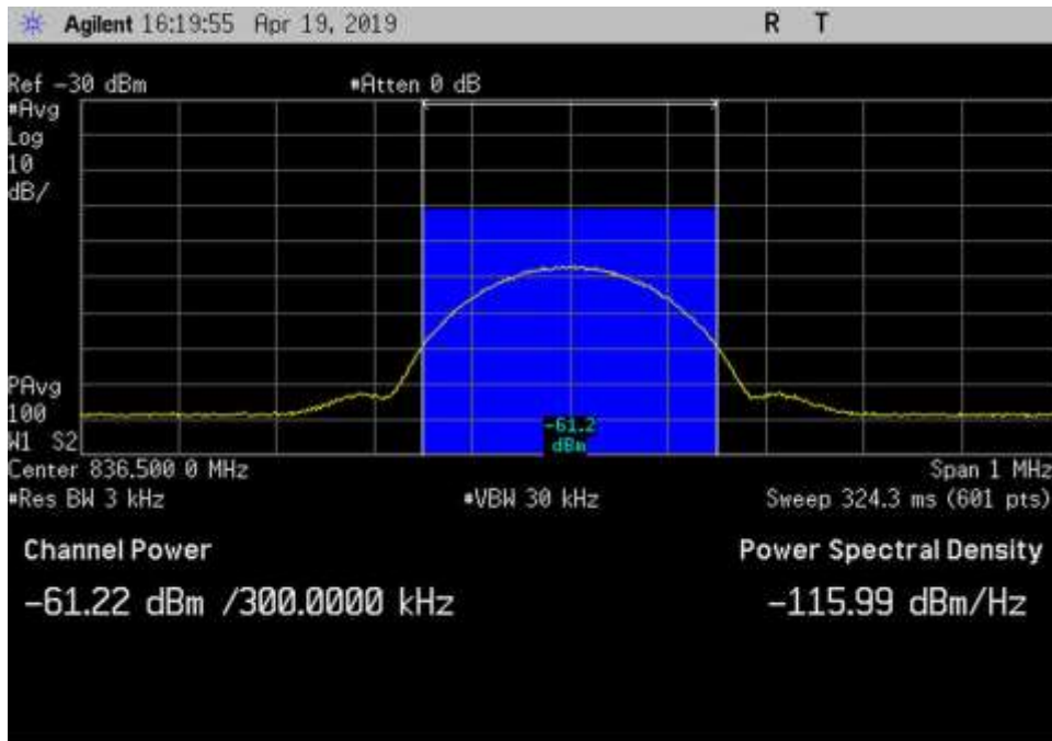
UL_824-849_GSM_836.5MHz_Input
