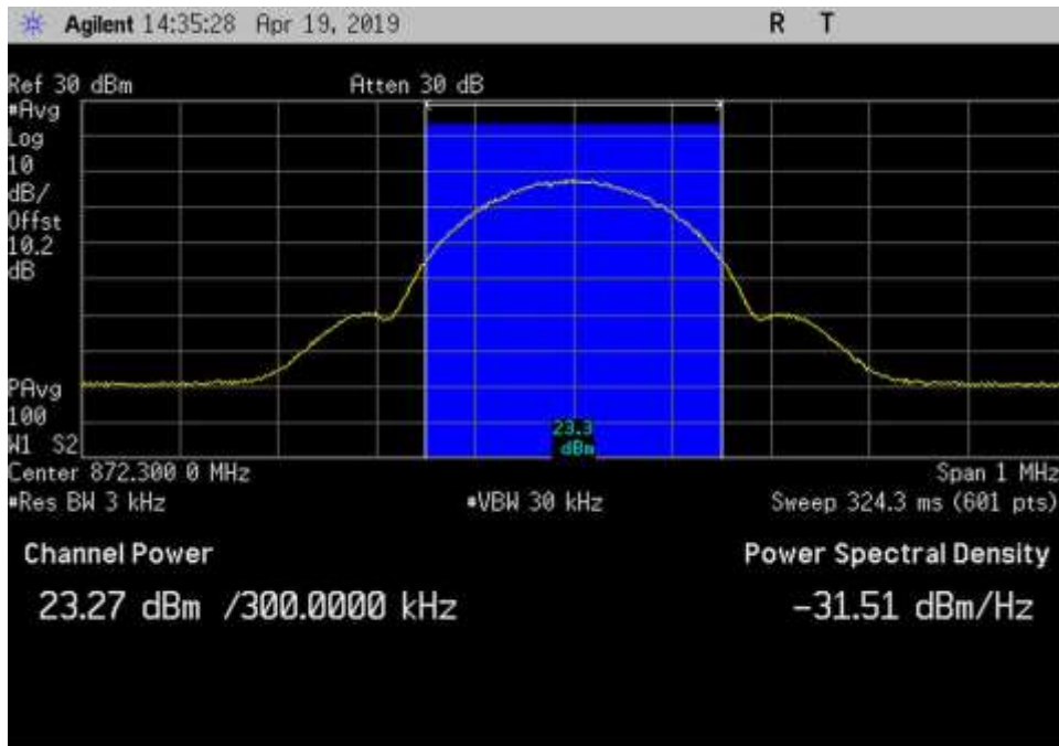
DL_869-894_GSM_ 872.3MHz_3dB
