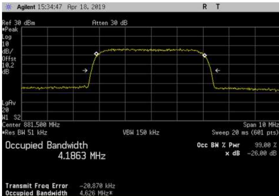
Out_DL_869-894_WCDMA_881.5MHz_3dB
