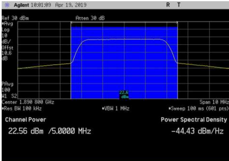
UL_1850-1915_AWGN_1890.8MHz
