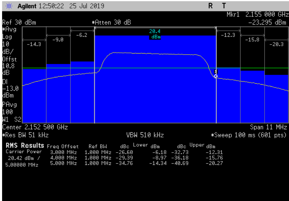
DL_2110-2155_AWGN_2147-2158MHz_Sn_H
