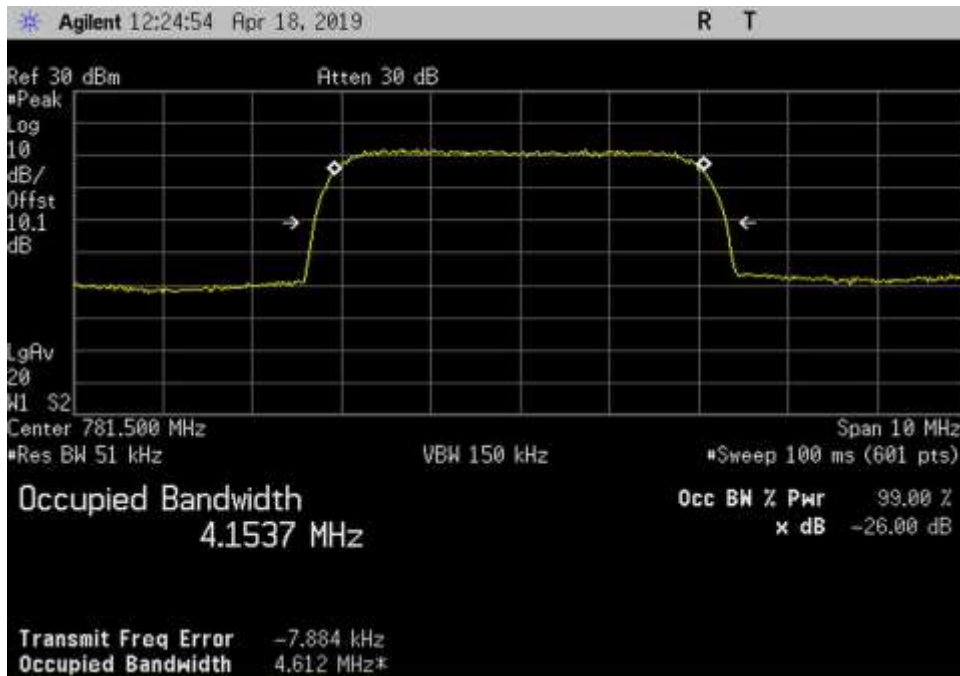
Out_UL_776-787_WCDMA_781.5MHz_3dB
