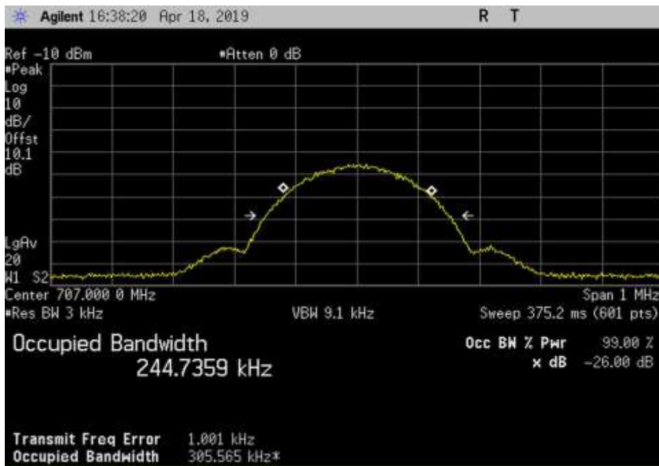
In_UL_698-716_GSM_707MHz
