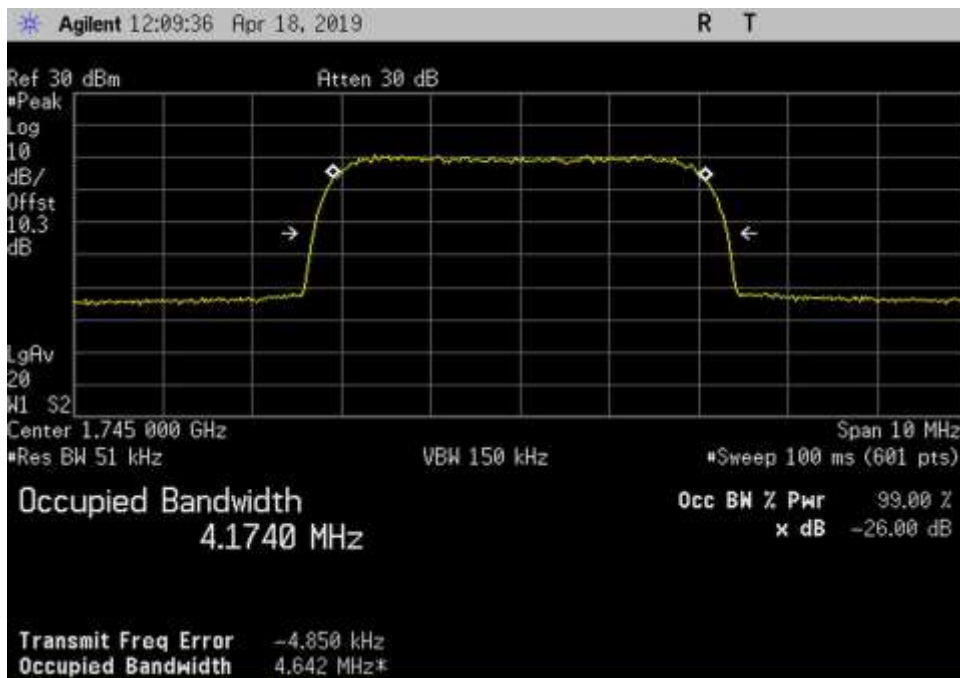
Out_UL_1710-1755_WCDMA_1745MHz_3dB
