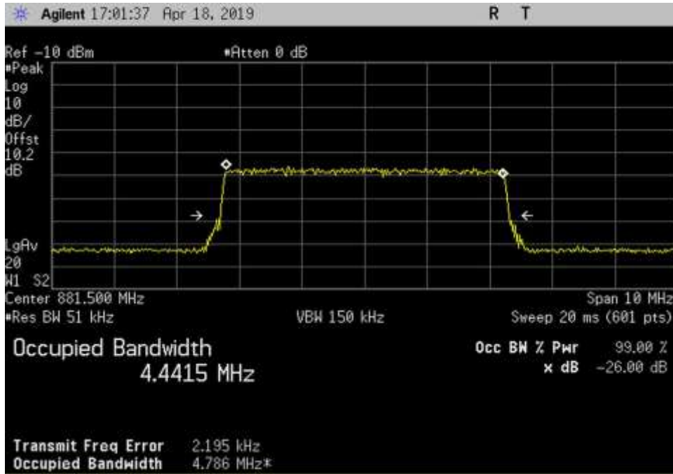
In_DL_869-894_LTE_881.5MHz
