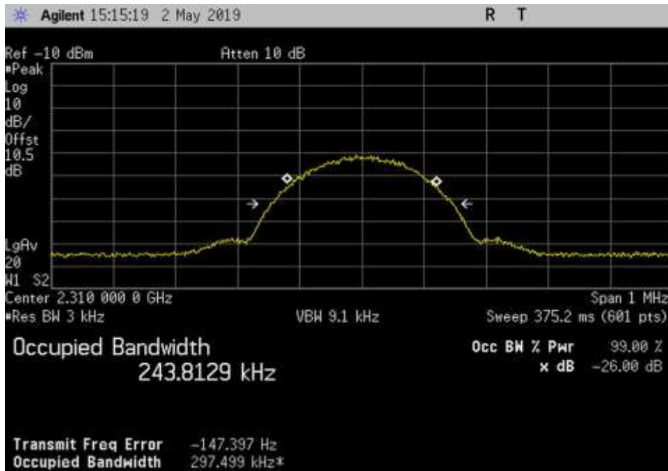
In_UL_2305-2315_GSM_2310MHz
