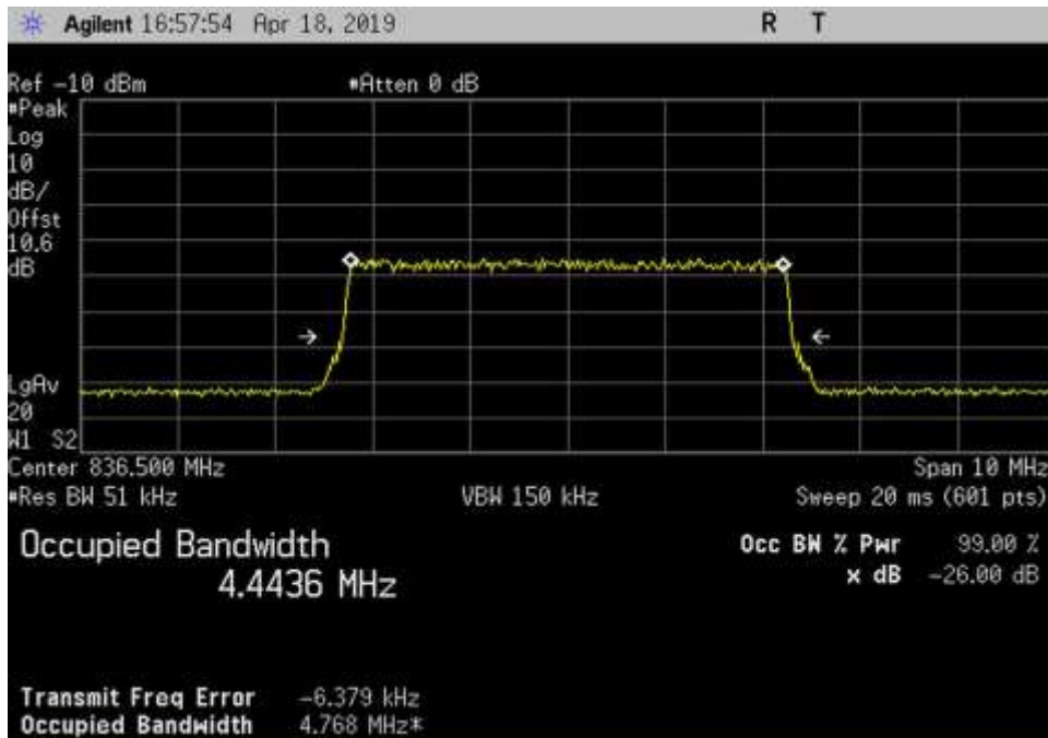
In_UL_824-849_LTE_836.5MHz
