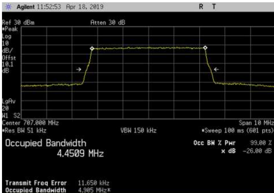
Out_UL_698-716_LTE_707MHz_3dB
