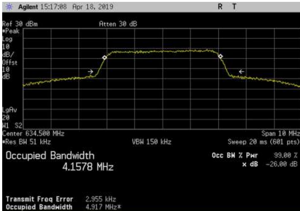
Out_DL_617-652_AWGN_634.5MHz_3dB
