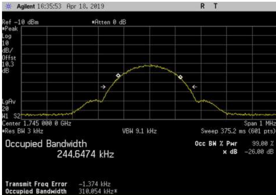
In_UL_1710-1755_GSM_1745MHz
