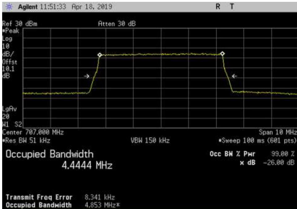
Out_UL_698-716_LTE_707MHz
