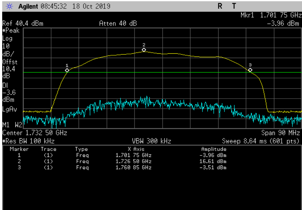
UL_1710-1755
