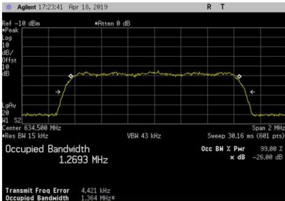
In_DL_617-652_CDMA_634.5MHz
