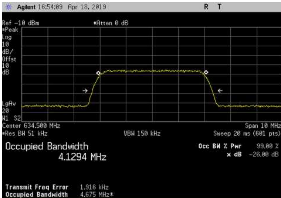
In_DL_617-652_AWGN_ 634.5MHz
