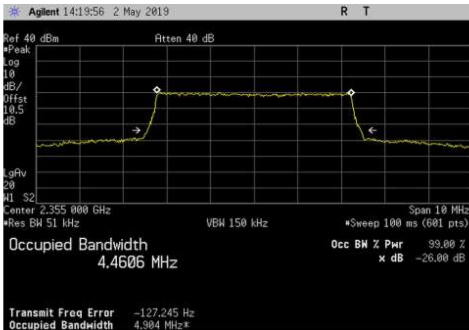
Out_DL_2350-2360_LTE_2355MHz_3dB
