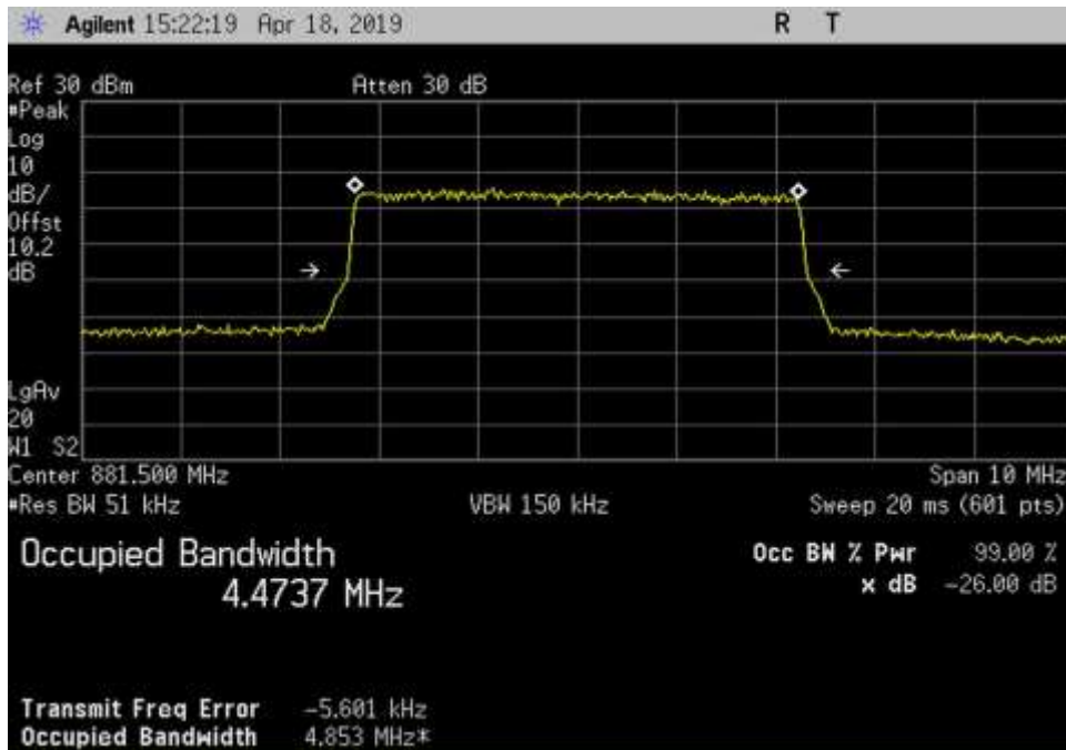
Out_DL_869-894_LTE_881.5MHz_3dB
