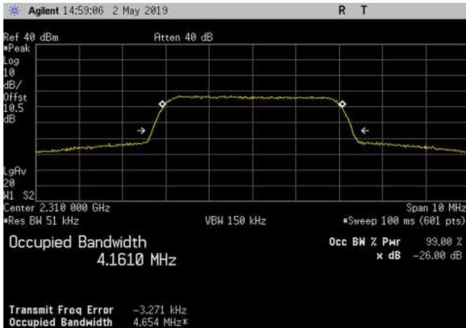
Out_UL_2305-2315_AWGN_2310MHz
