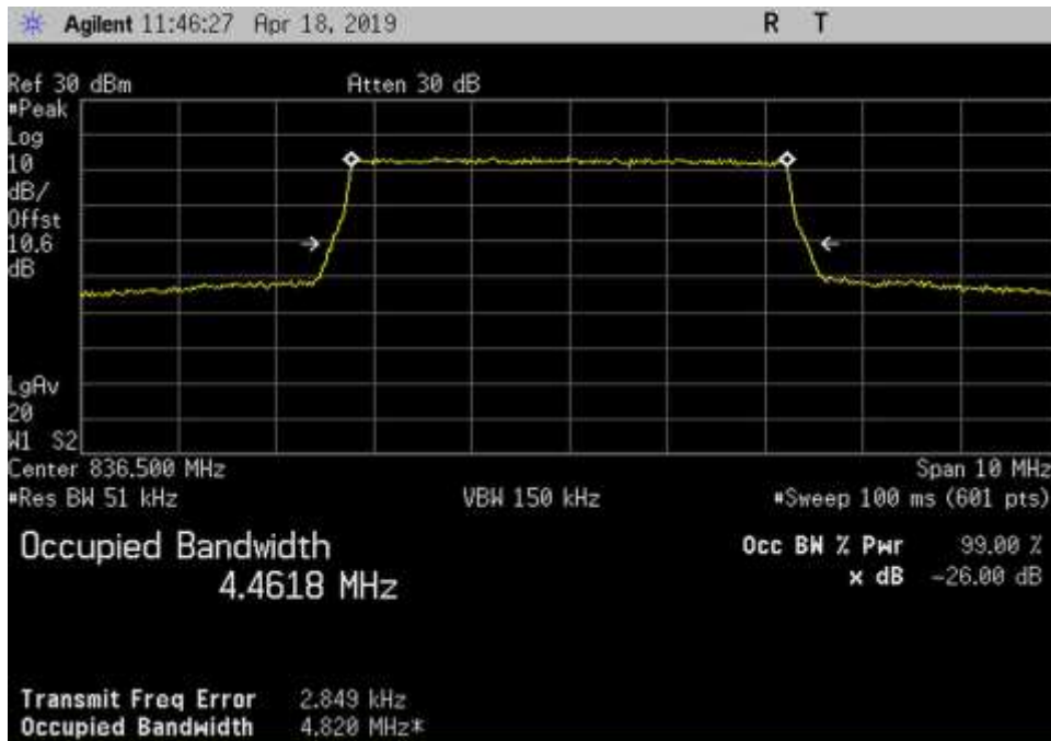
Out_UL_824-849_LTE_836.5MHz
