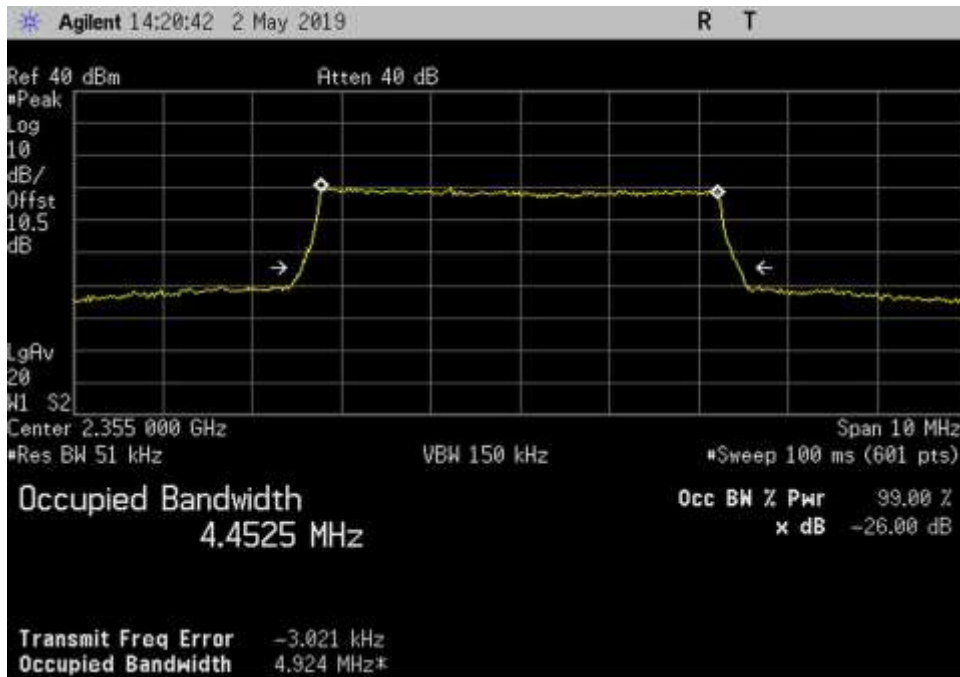
Out_DL_2350-2360_LTE_2355MHz
