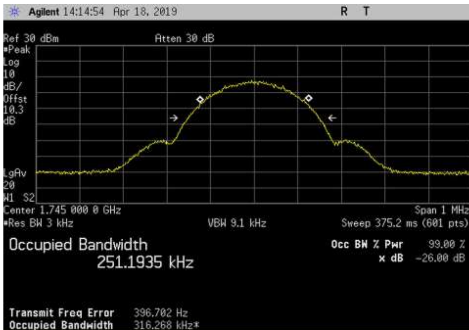
Out_UL_1710-1755_GSM_1745MHz.
