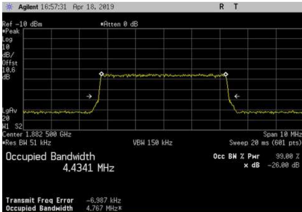
In_UL_1850-1915_LTE_1882.5MHz
