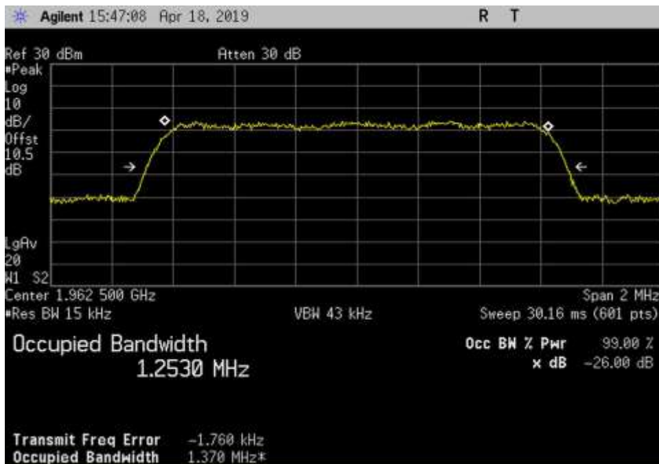
Out_DL_1930-1995_CDMA_1962.5MHz_3dB
