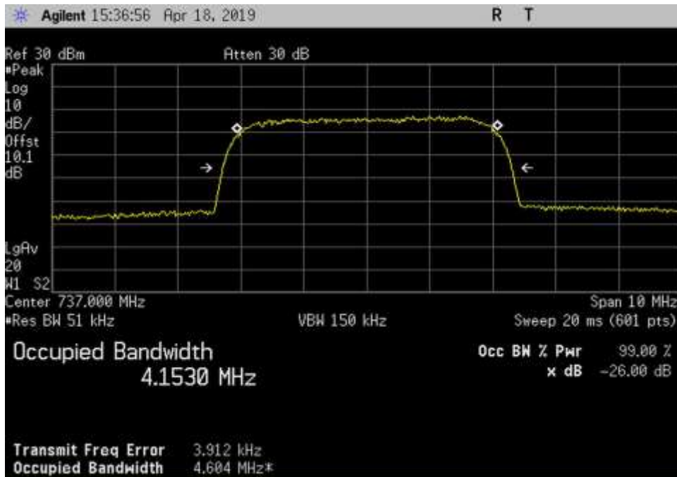
Out_DL_728-746_WCDMA_737MHz
