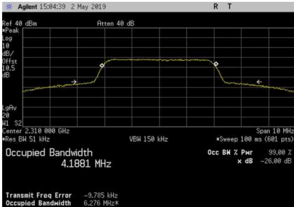
Out_UL_2305-2315_AWGN_2310MHz_3dB
