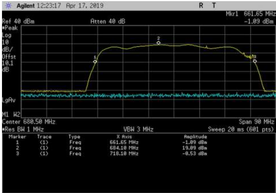
UL_663-698
