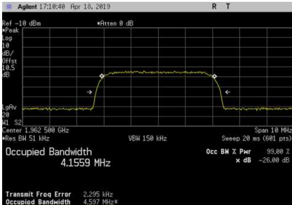
In_DL_1930-1995_WCDMA_1962.5MHz
