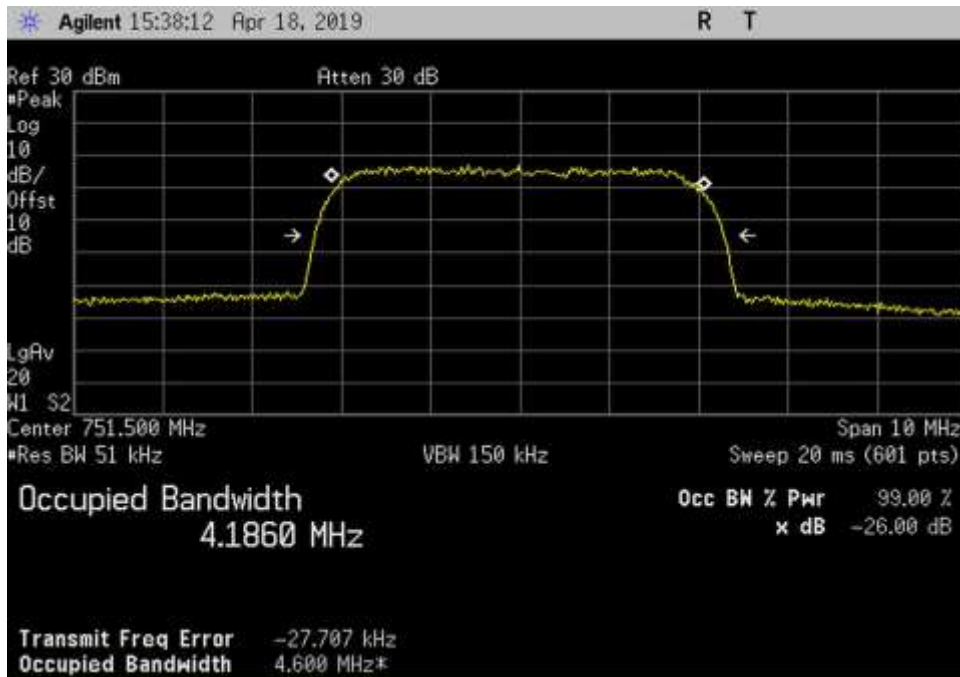
Out_DL_746-757_WCDMA_751.5MHz
