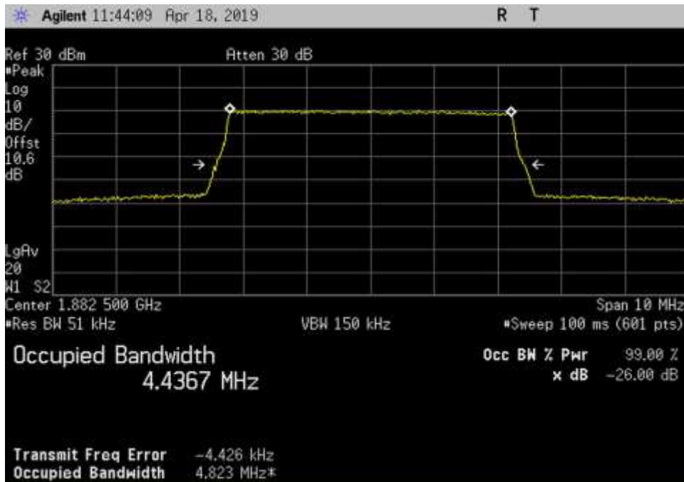
Out_UL_1850-1915_LTE_1882.5MHz
