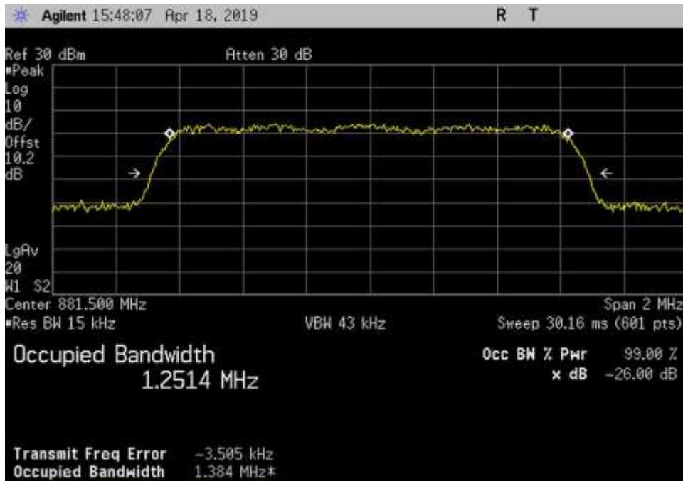
Out_DL_869-894_CDMA_ 881.5MHz
