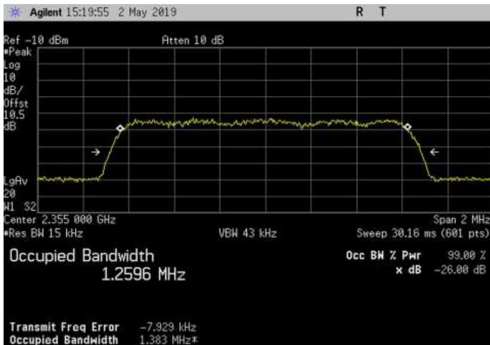
In_DL_2350-2360_CDMA_2355MHz
