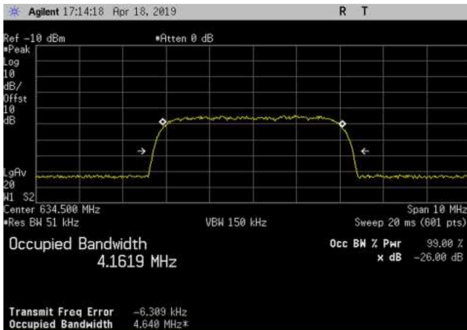
In_DL_617-652_WCDMA_634.5MHz
