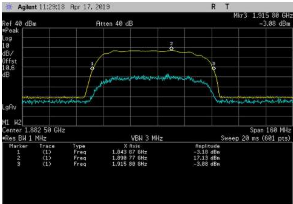
UL_1850-1915
