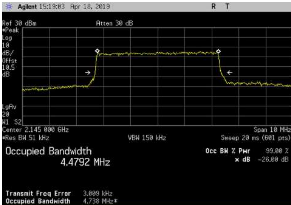
Out_DL_2110-2155_LTE_2145MHz
