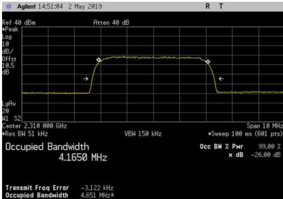
Out_UL_2305-2315_WCDMA_2310MHz
