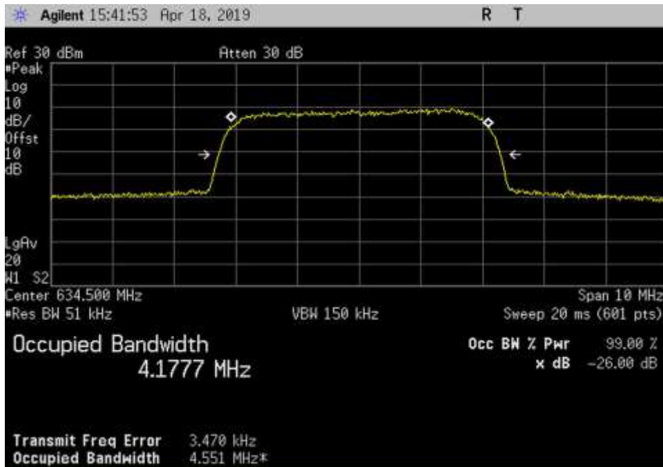
Out_DL_617-652_WCDMA_634.5MHz
