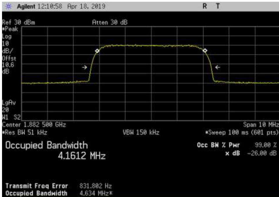
Out_UL_1850-1915_WCDMA_1882.5MHz
