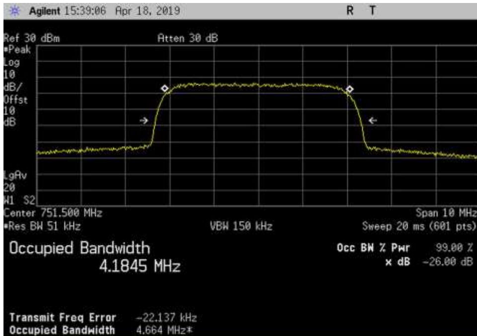
Out_DL_746-757_WCDMA_751.5MHz_3dB
