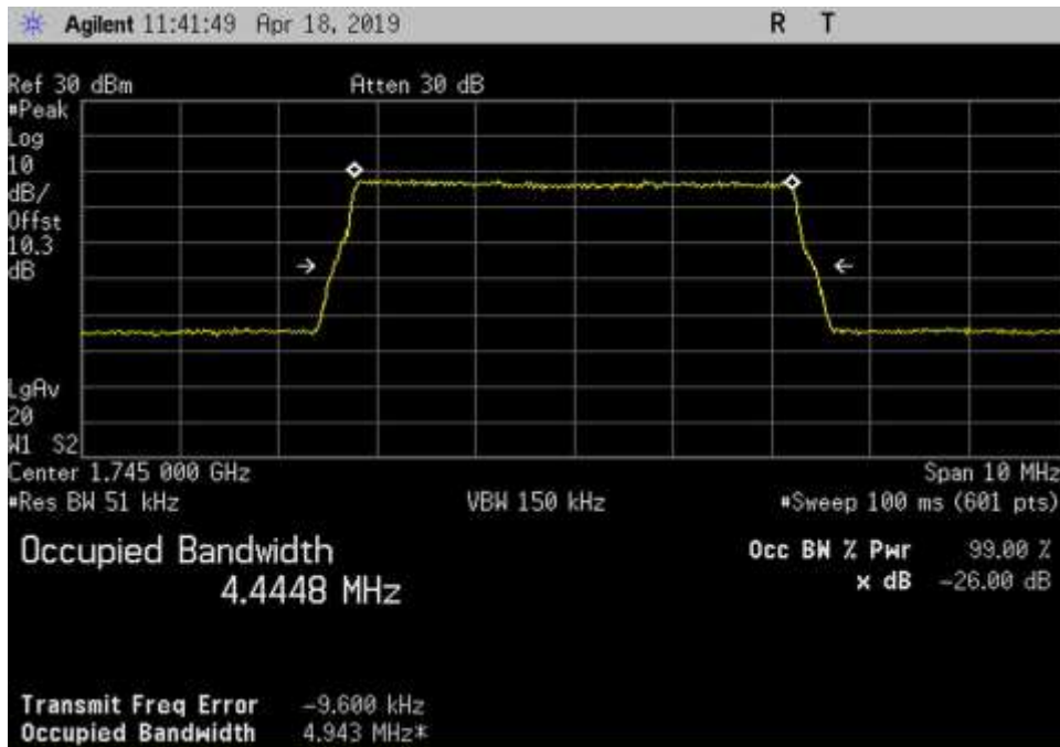
Out_UL_1710-1755_LTE_1745MHz
