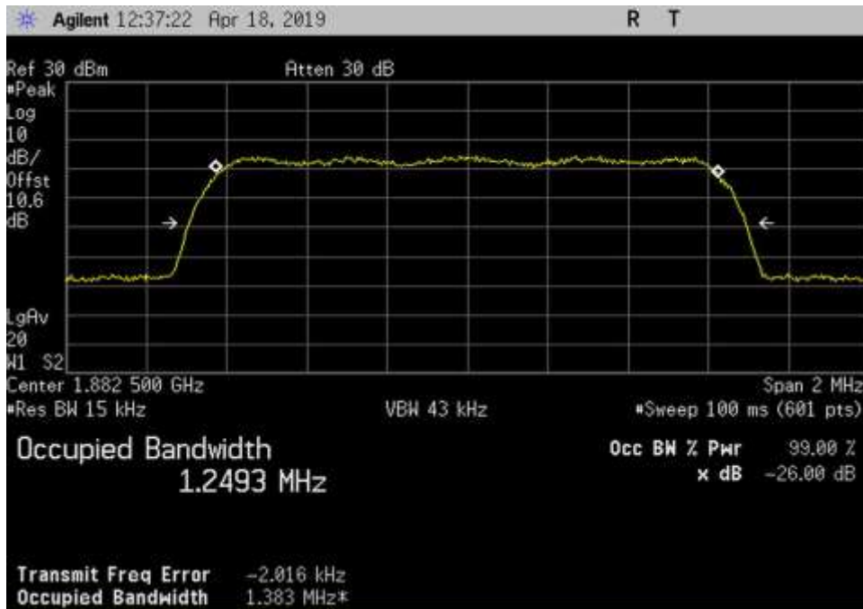
Out_UL_1850-1915_CDMA_1882.5MHz
