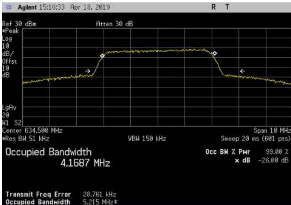
Out_DL_617-652_AWGN_634.5MHz
