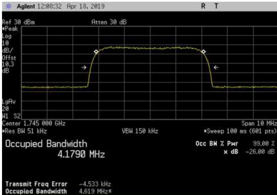
Out_UL_1710-1755_WCDMA_1745MHz
