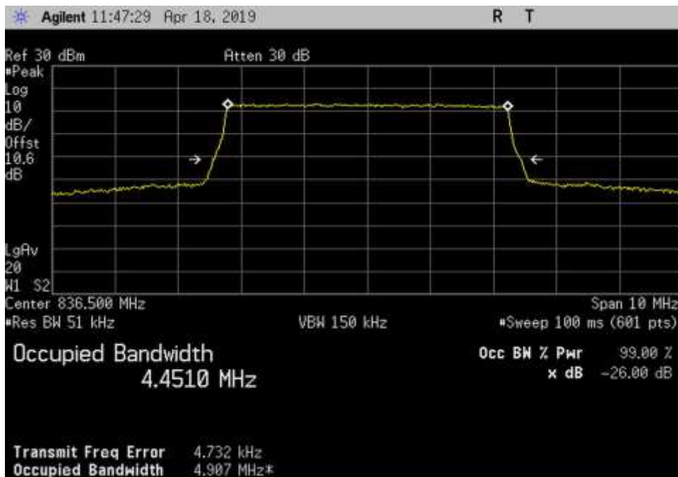
Out_UL_824-849_LTE_836.5MHz_3dB
