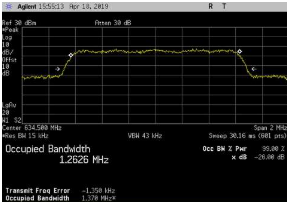
Out_DL_617-652_CDMA_ 634.5MHz
