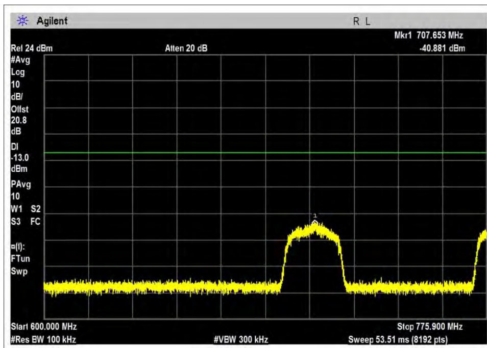
UL-776-787L-AWGN-H
