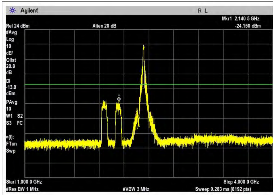
DL-746-757-AWGN-L
