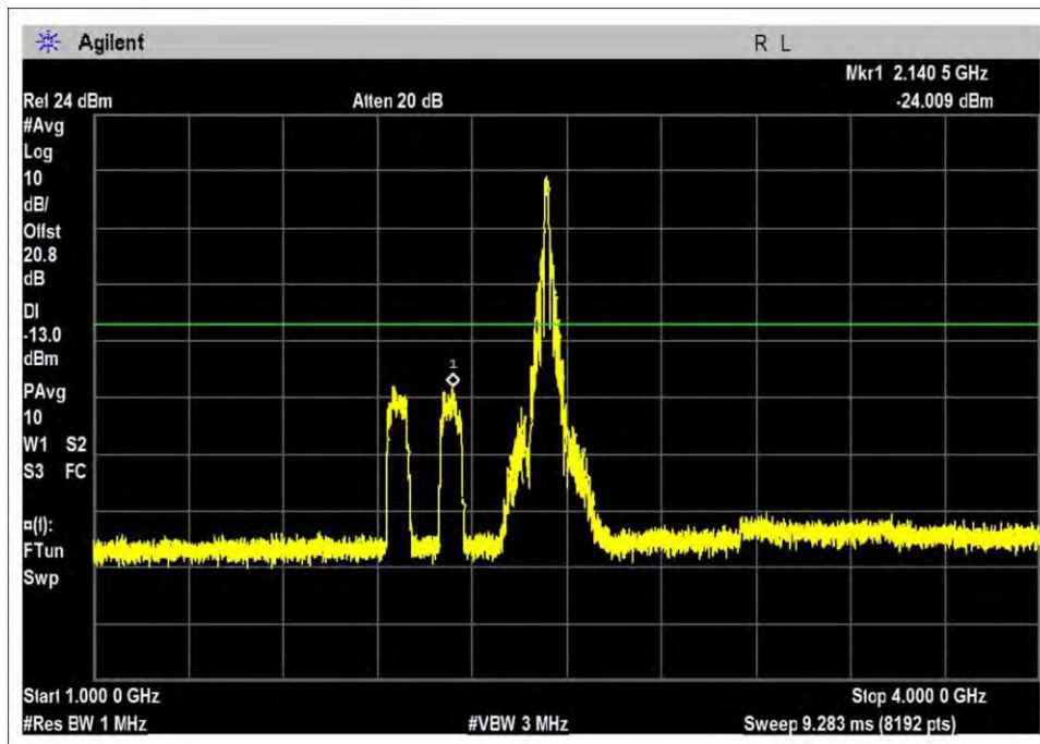
DL-746-757-AWGN-M
