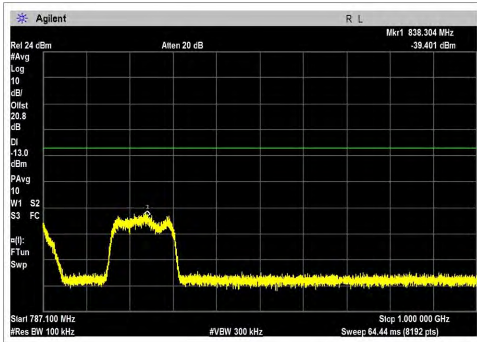
UL-776-787R-AWGN-L
