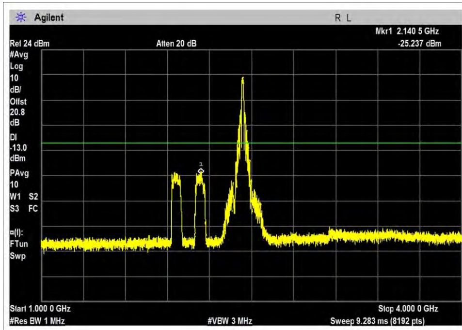
DL-746-757-GSM-M
