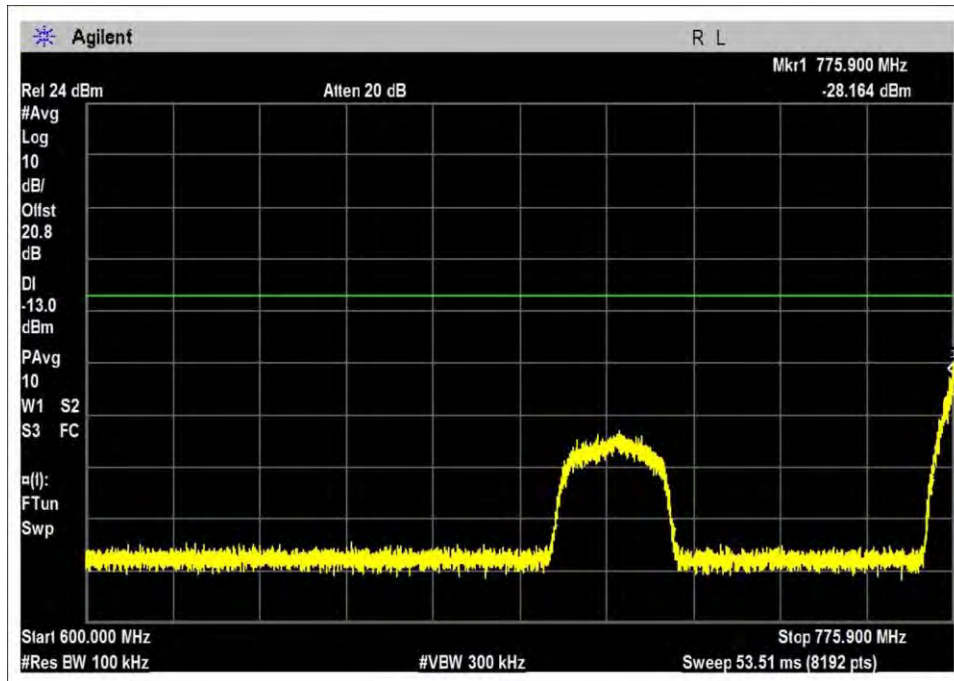
UL-776-787L-AWGN-L
