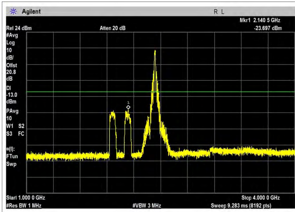
DL-746-757-GSM-L
