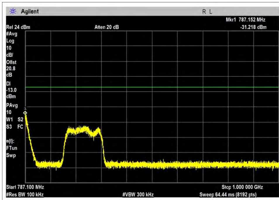
UL-776-787R-AWGN-H
