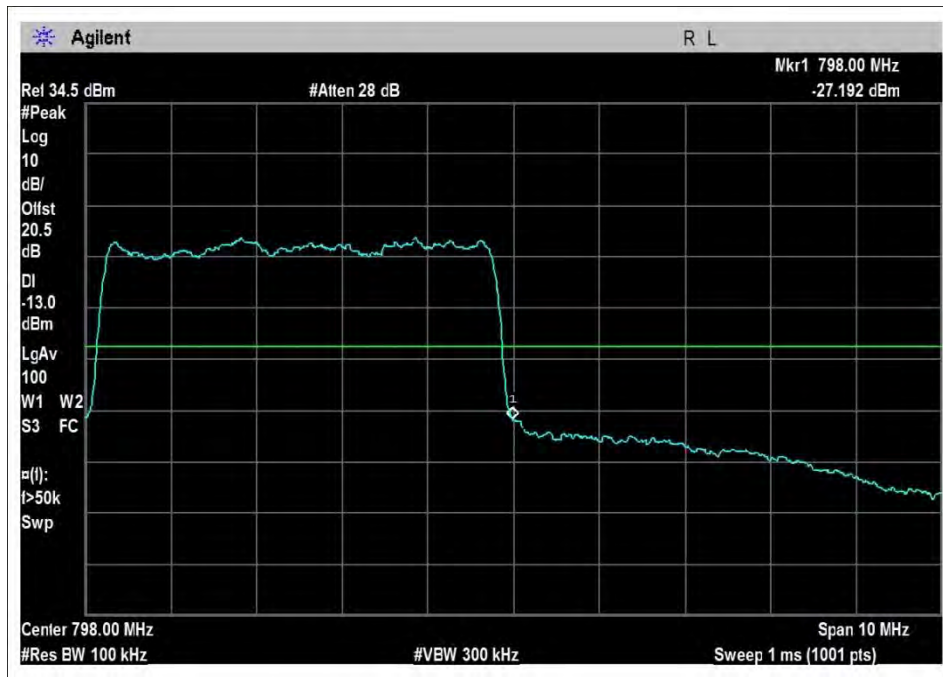
LTE-UL-788-798H-AGC+10dB
