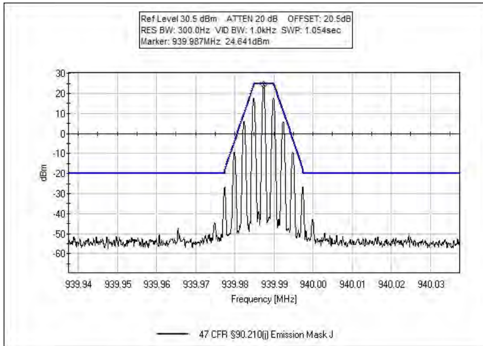
900M_FM_DL-940H-MaskJ
