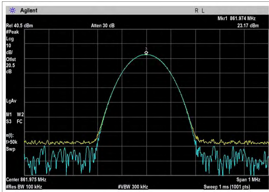
DL-851-862H-Unmod-25.2
