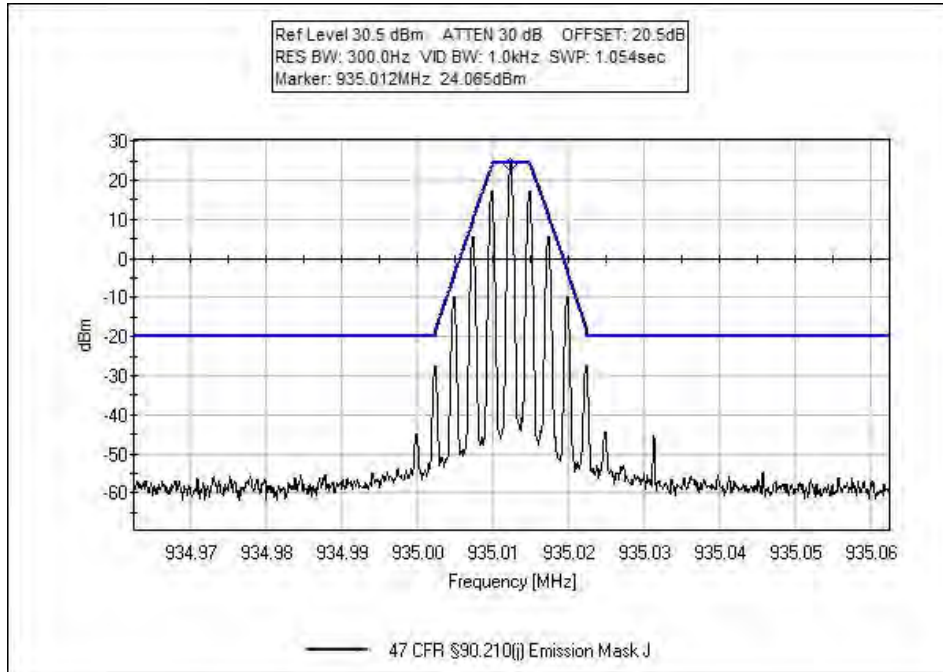
900M_FM_DL-935L-MskJ
