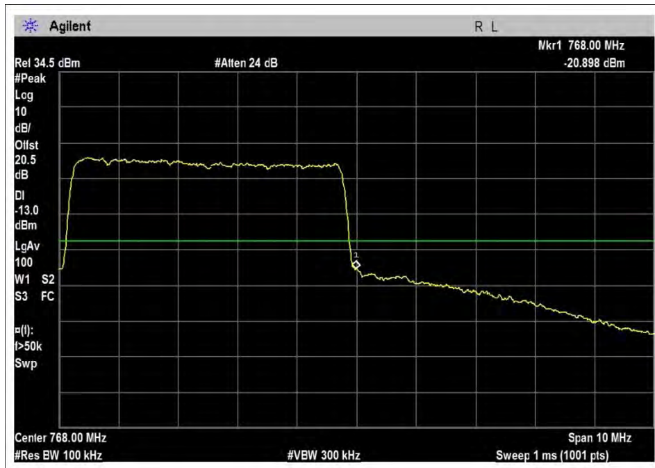
LTE-DL-758-768H-AGC
