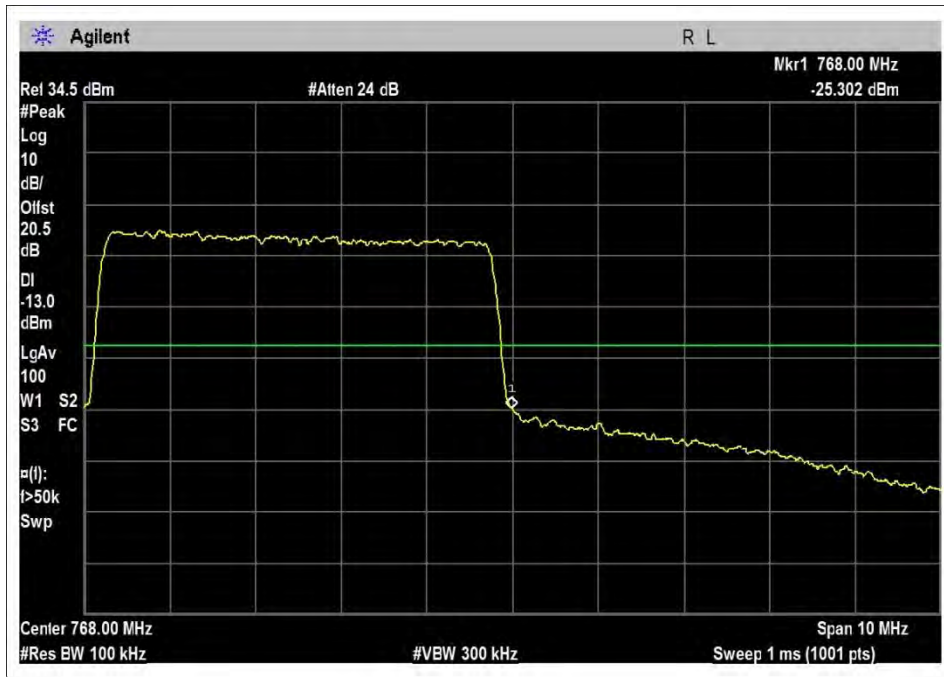
LTE-DL-758-768H-33
