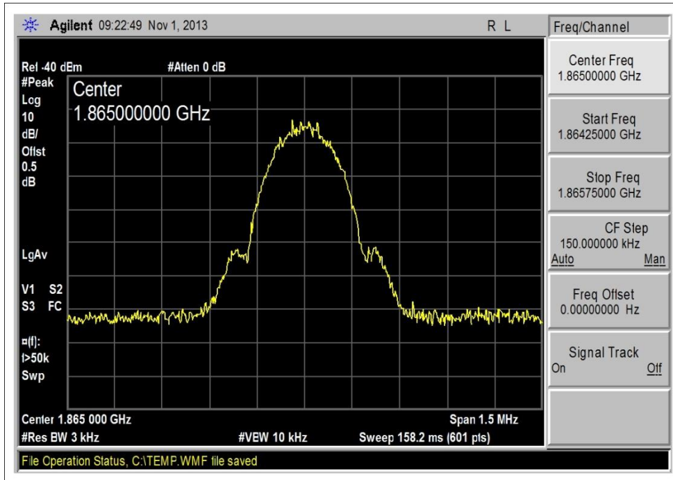
1850-1910MHz UL_GSM_Input
