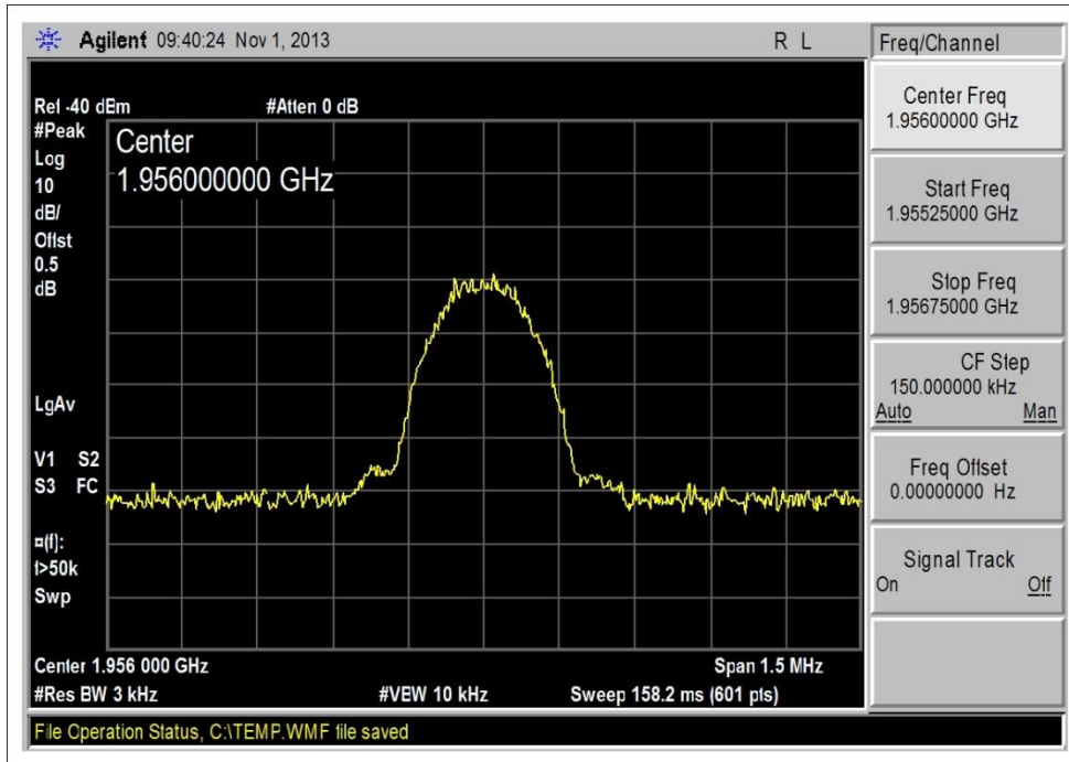
1930-1990MHz DL_GSM_Input
