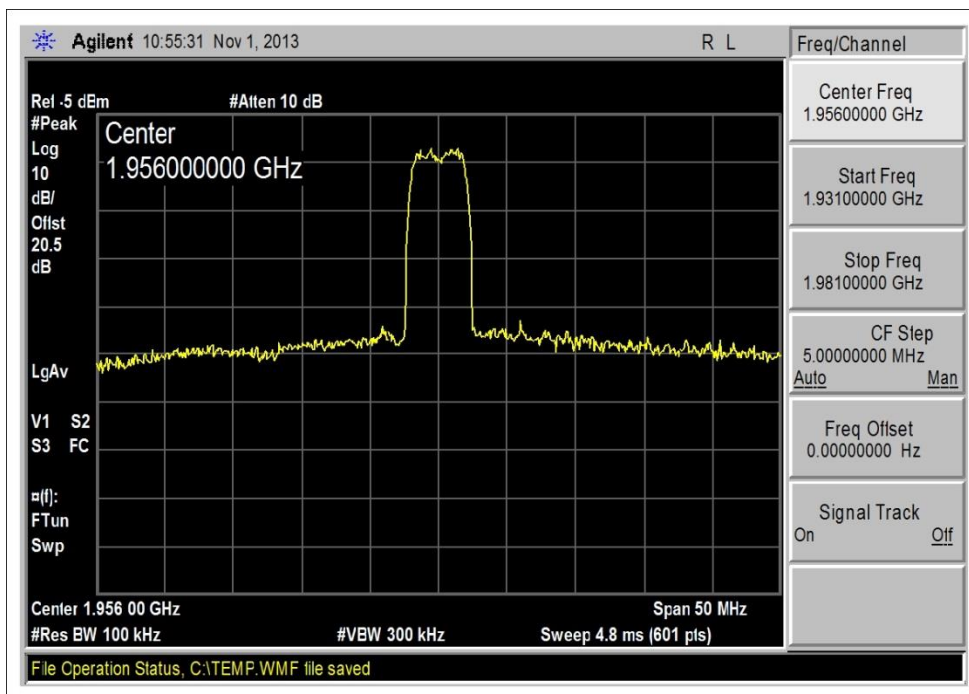
1930-1990MHz DL_WCDMA_Output
