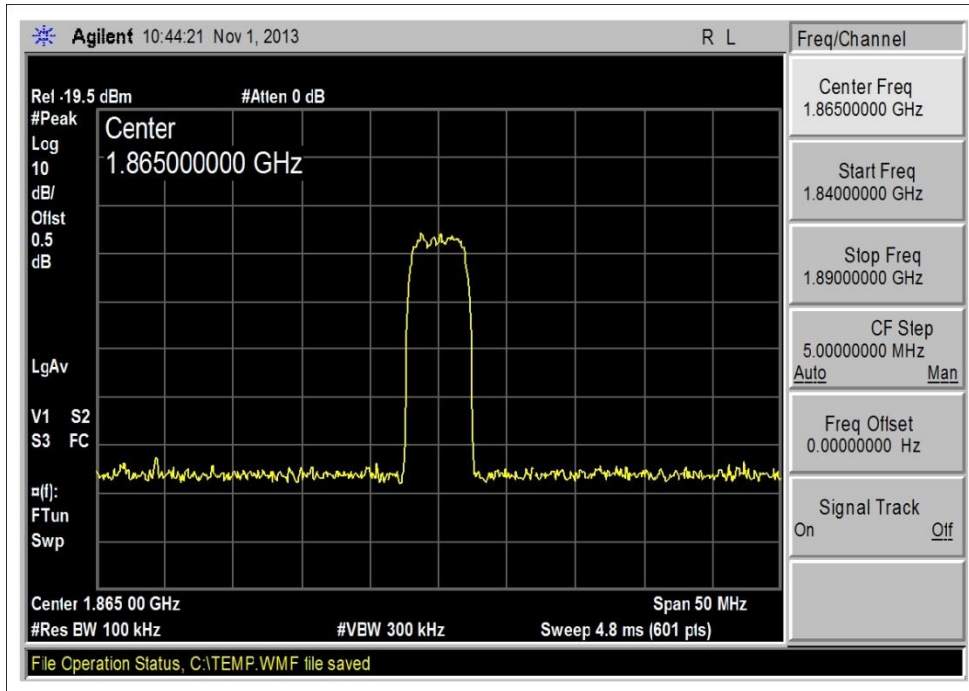
1850-1910MHz UL_WCDMA_Input
