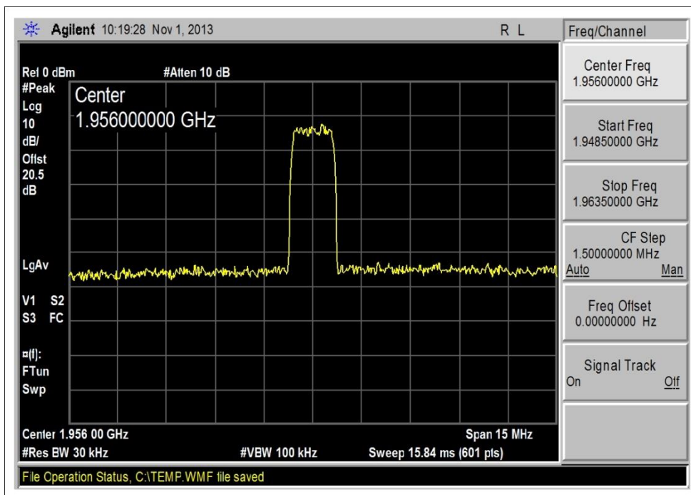
1930-1990MHz DL_CDMA_Output
