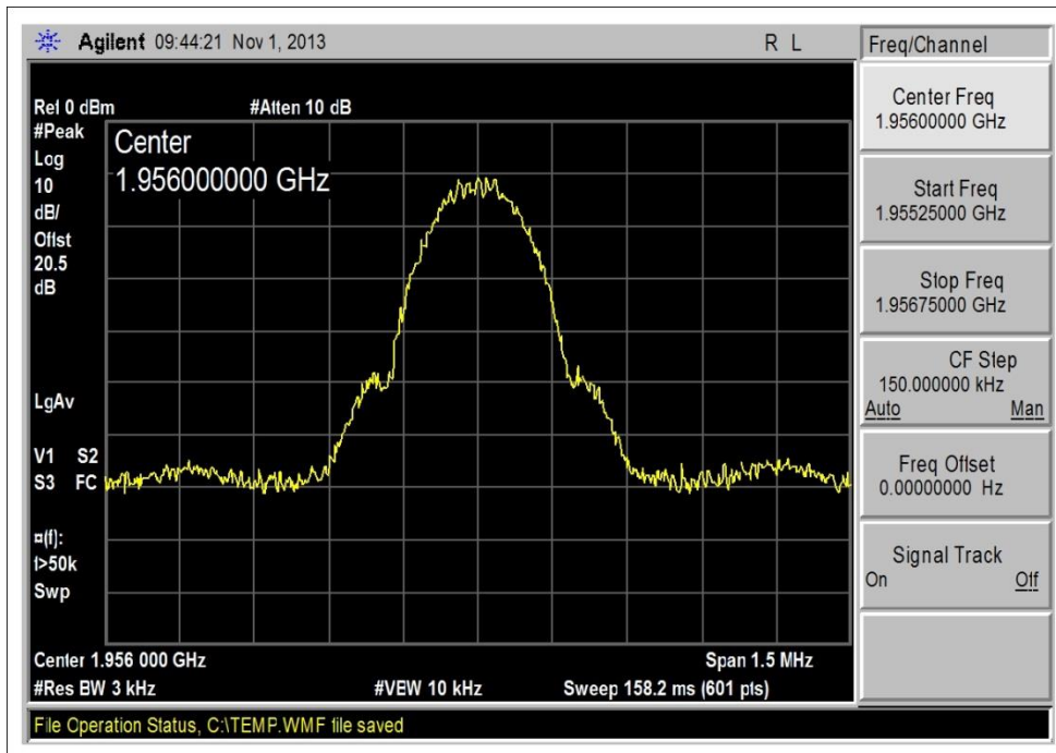
1930-1990MHz DL_GSM_Output
