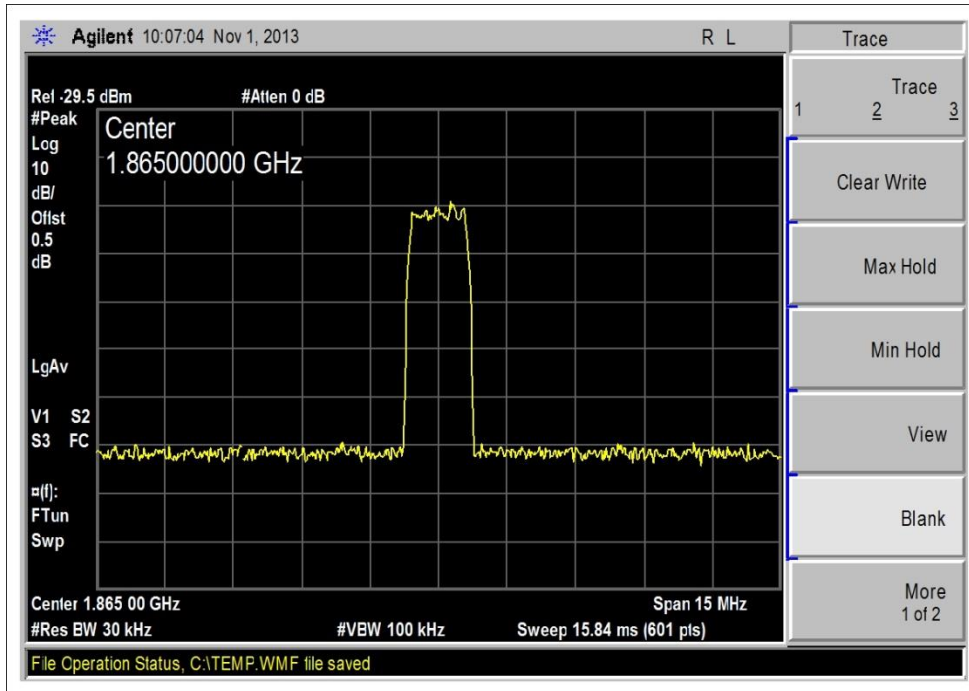
1850-1910MHz UL_CDMA_Input
