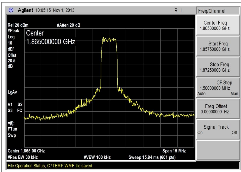
1850-1910MHz UL_CDMA_Output
