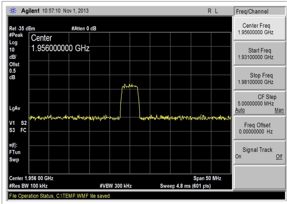
1930-1990MHz DL_WCDMA_Input
