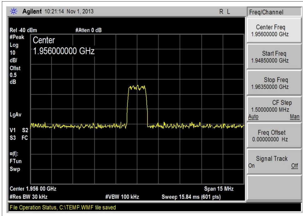
1930-1990MHz DL_CDMA_Input
