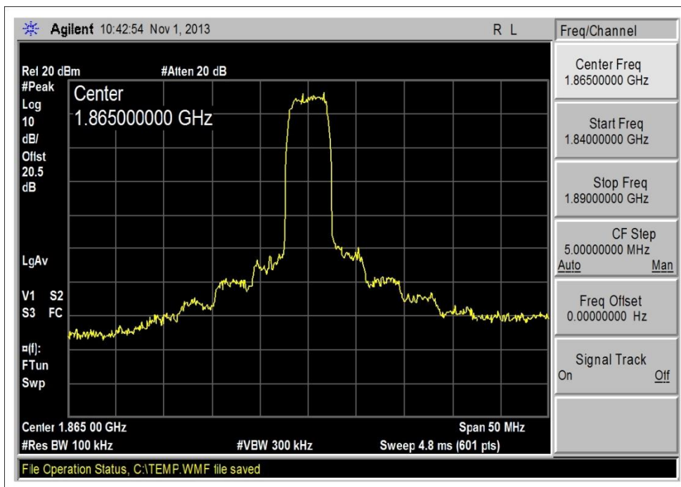
1850-1910MHz UL_WCDMA_Output
