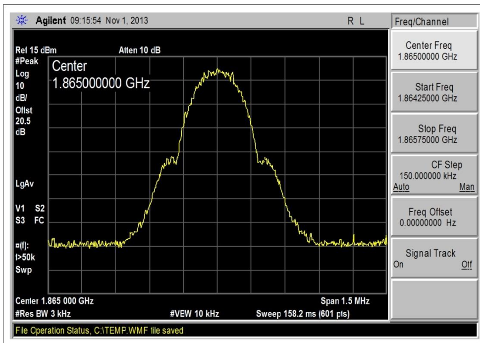
1850-1910MHz UL_GSM_Output
