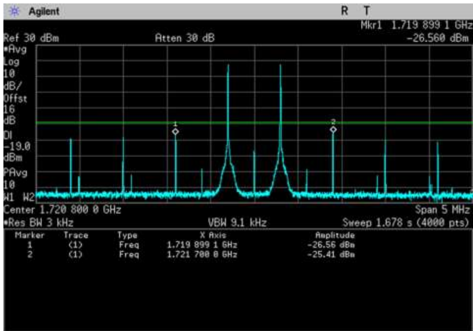
UL_1710-1755_1720.8MHz
