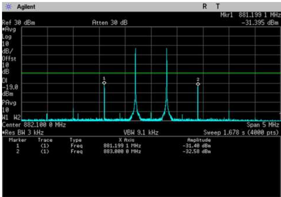
DL_869-894_ 882.1MHz
