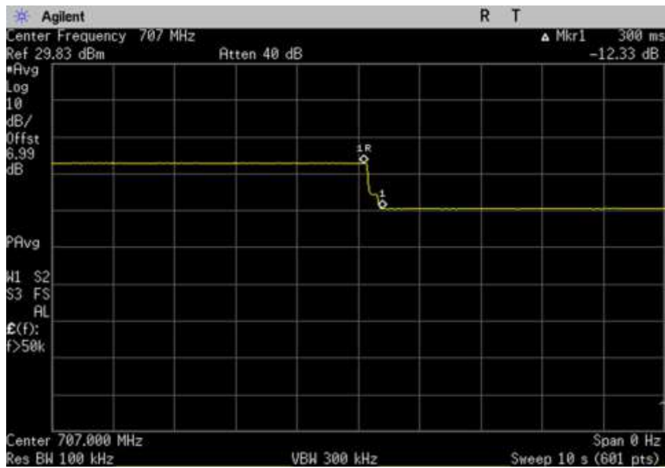
UL_698-716_707MHz_VAR
