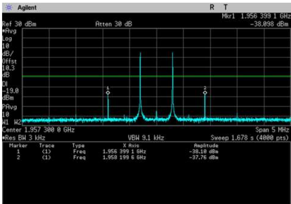
DL_1930-1995_ 1957.3MHz
