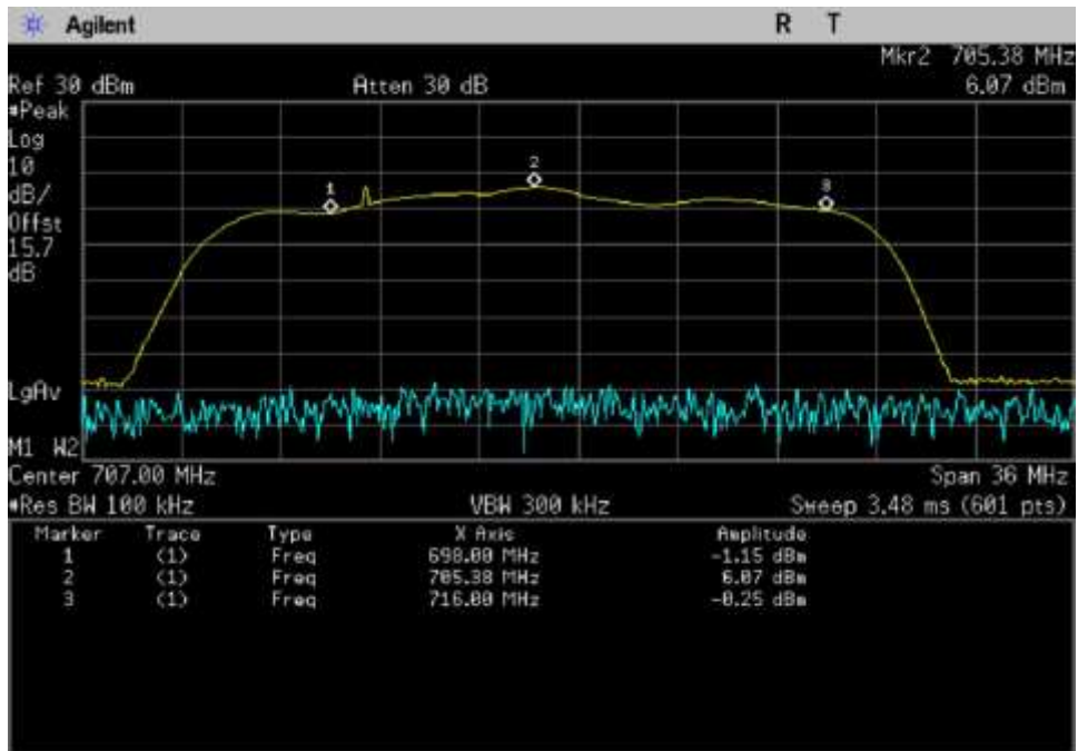
UL_698-716_698-705.38MHz
