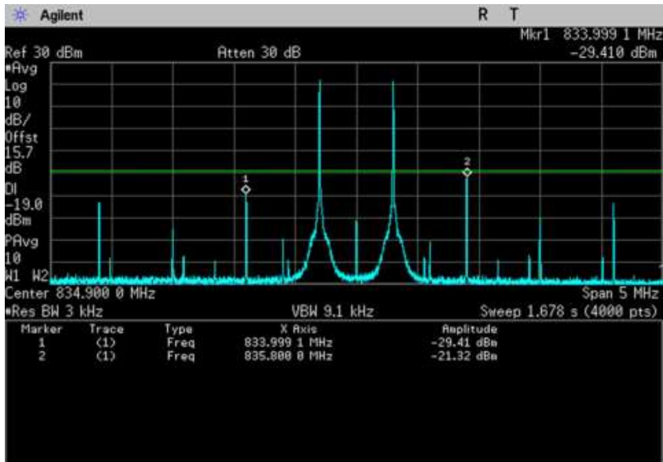
UL_824-849_ 834.9MHz
