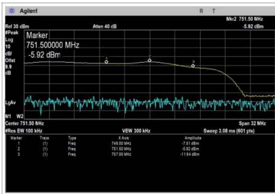
DL_746-757_746- 751.5MHz
