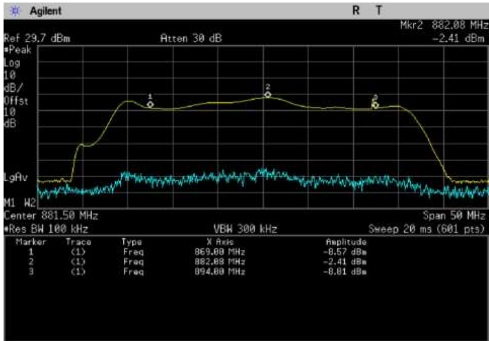
DL_869-894_ 869- 882.08MHz
