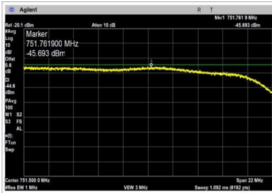
DL_746-757_ 751.5MHz
