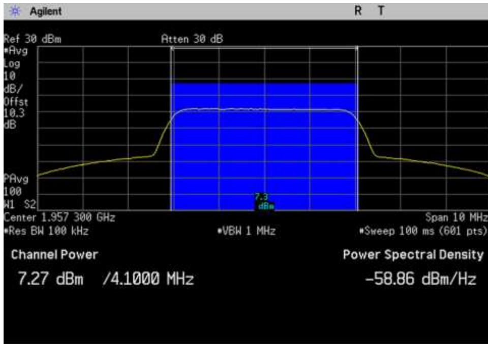
DL_1930-1995_AWGN_Max_1957.3MHz
