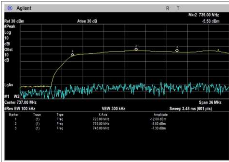
DL_728-746_728- 739.0MHz
