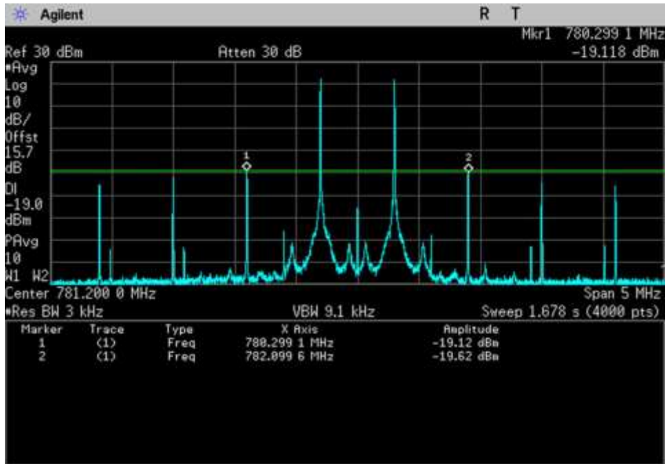
UL_776-787_ 781.2MHz
