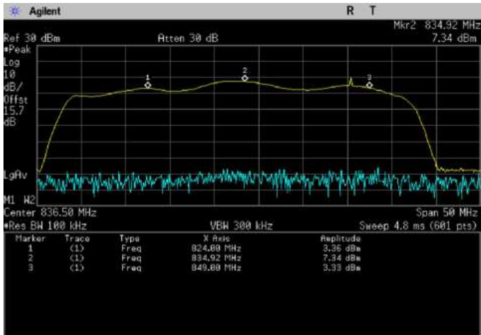
UL_824-849_ 824- 834.92MHz
