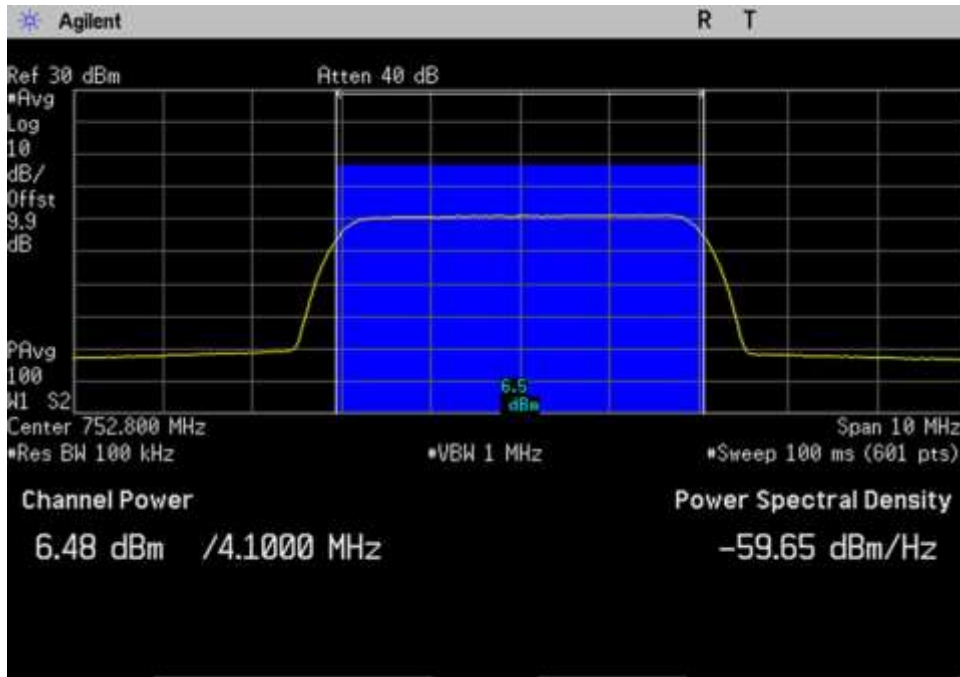
DL_746-757_AWGN_752.8MHz
