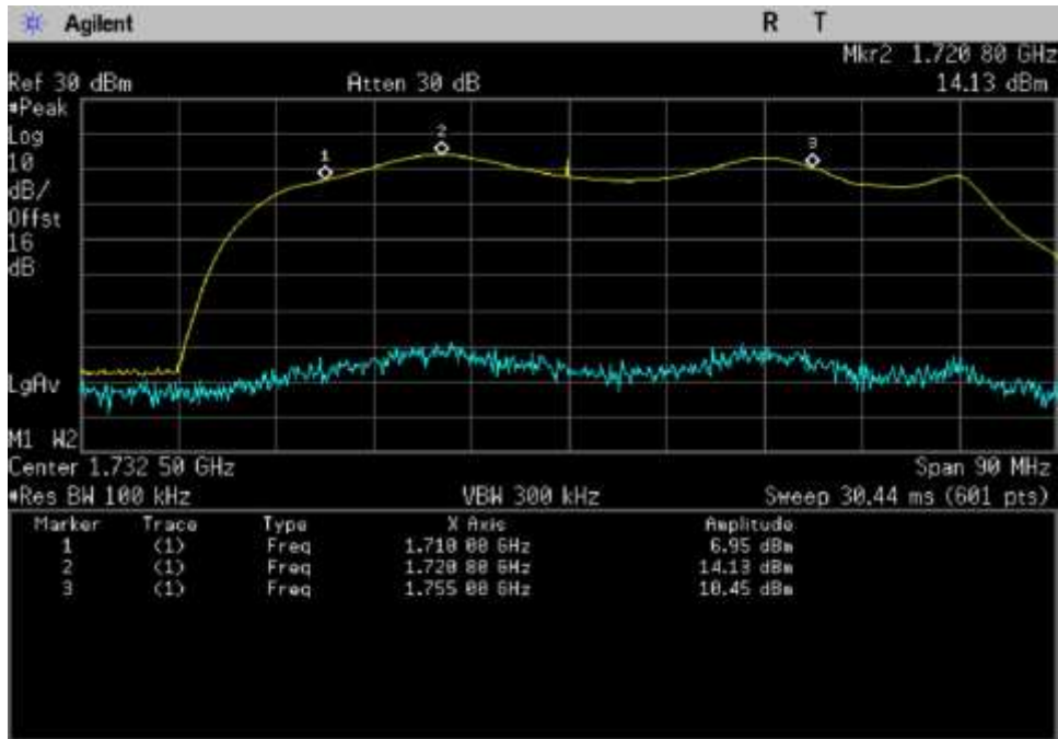
UL_1710-1755_1710-1720.8MHz
