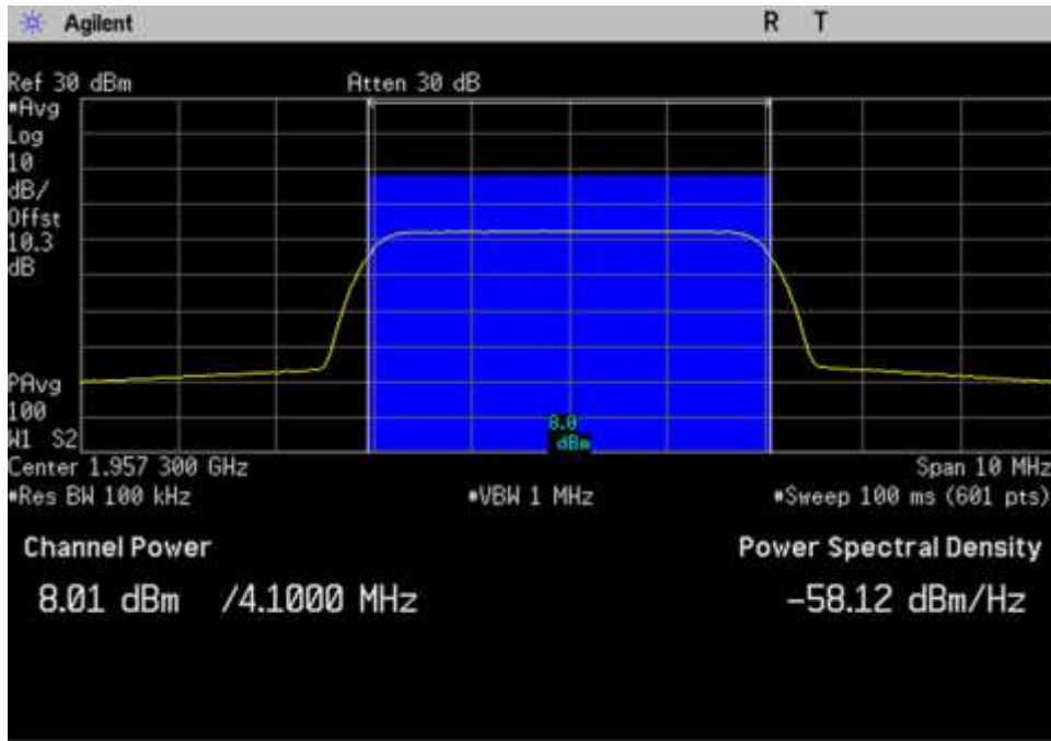
DL_1930-1995_AWGN_1957.3MHz
