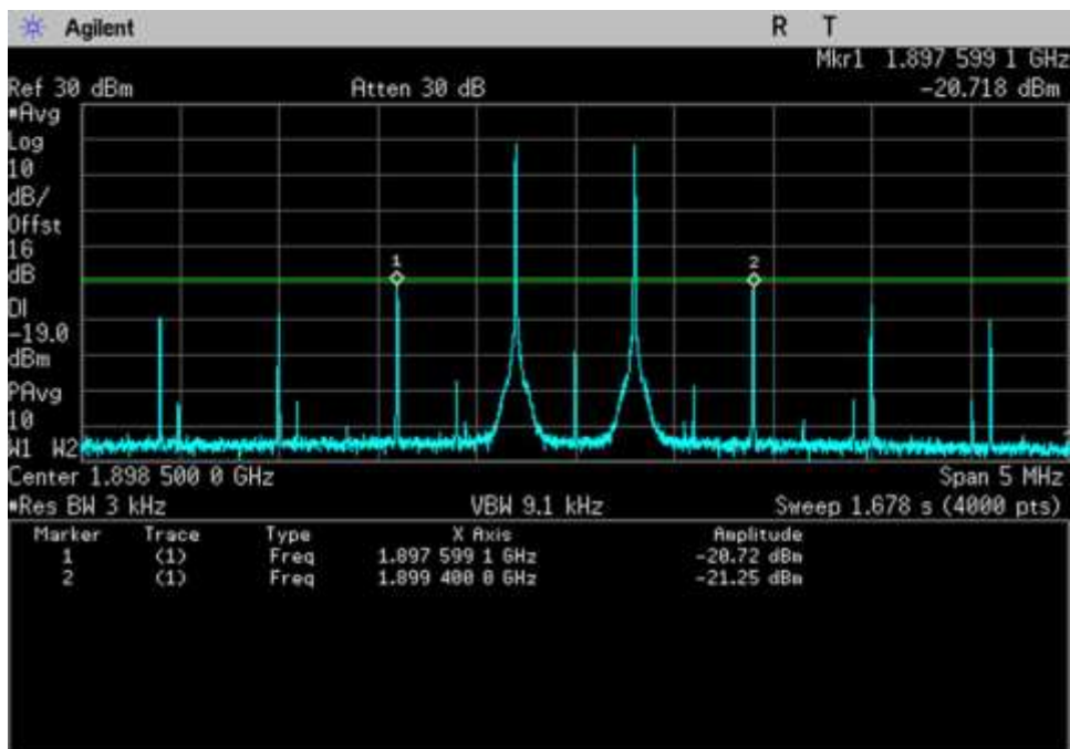
UL_1850-1915_1898.5MHz
