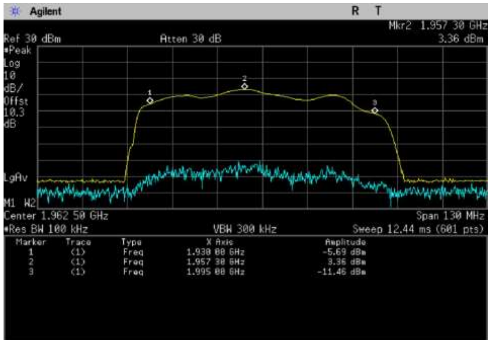
DL_1930-1995_ 1930- 1957.3MHz
