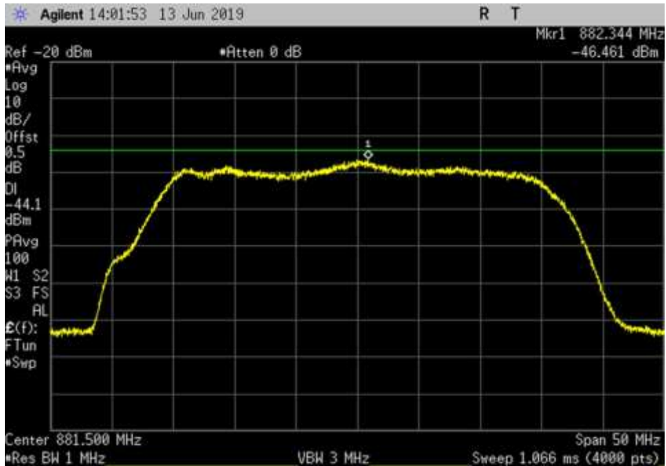
DL_869-894_881.5MHz_165ft Cable
