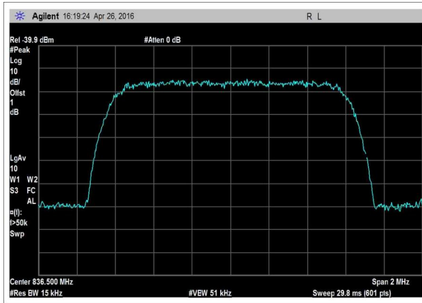
OBW_UL_824-849MHz_CDMA
