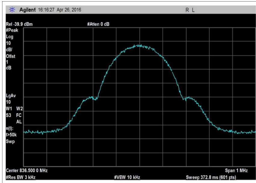
OBW_UL_824-849MHz_GSM
