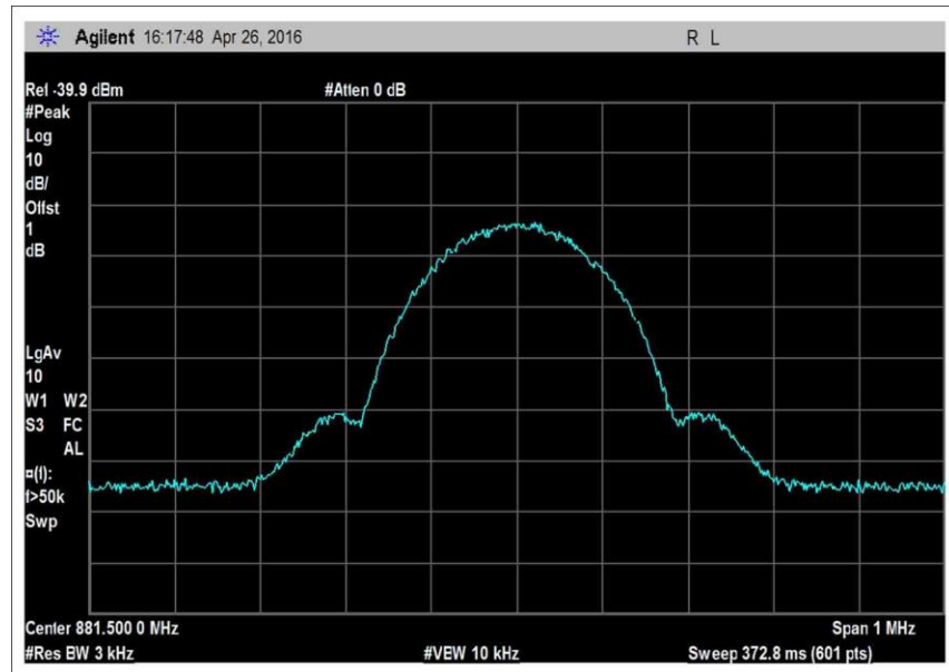
OBW_DL_869-894MHz_GSM
