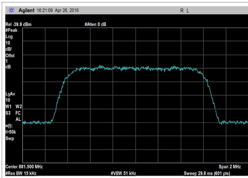
OBW_DL_869-894MHz_CDMA
