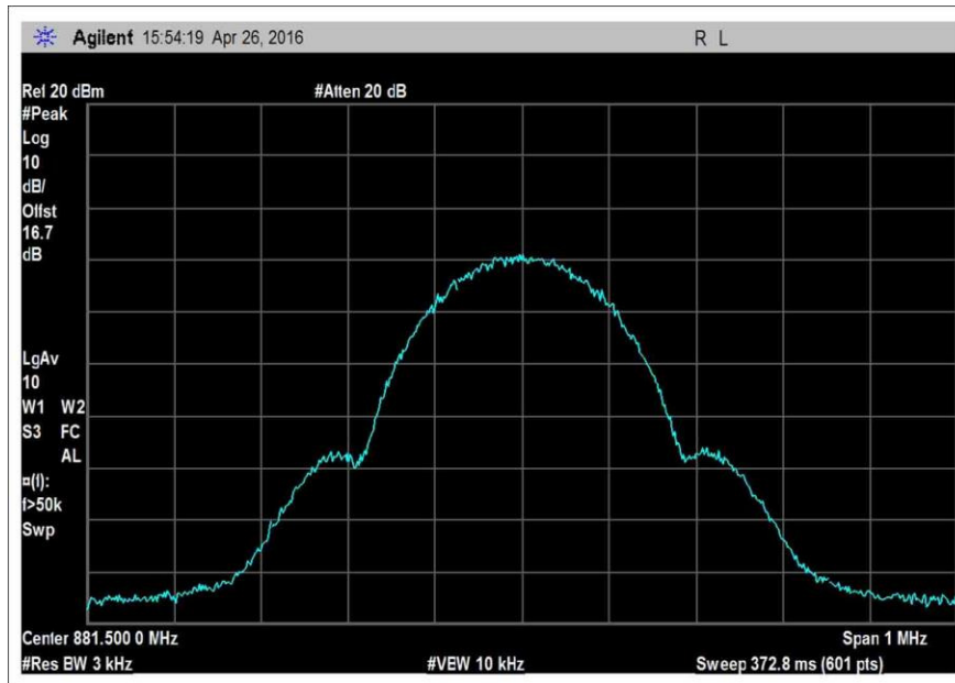
OBW_DL_869-894MHz_GSM
