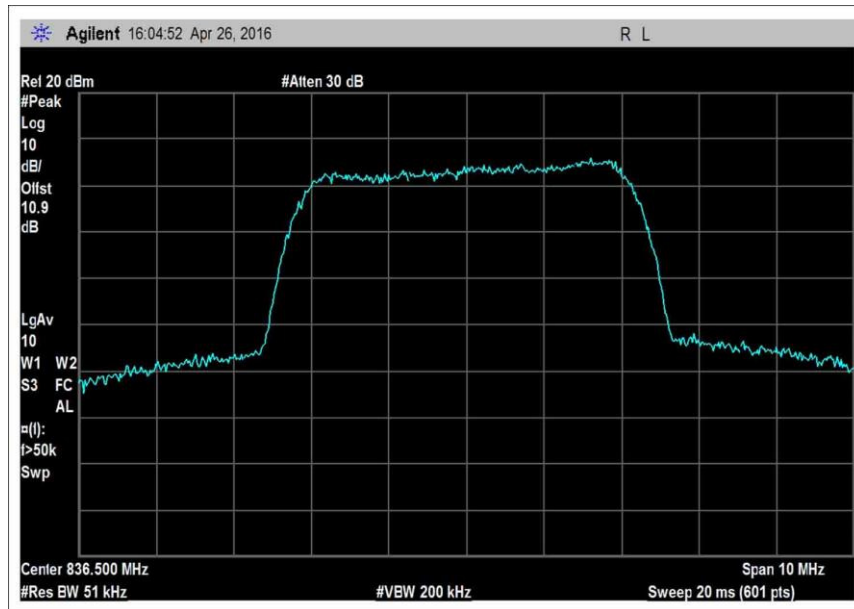
OBW_UL_824-849MHz_WCDMA
