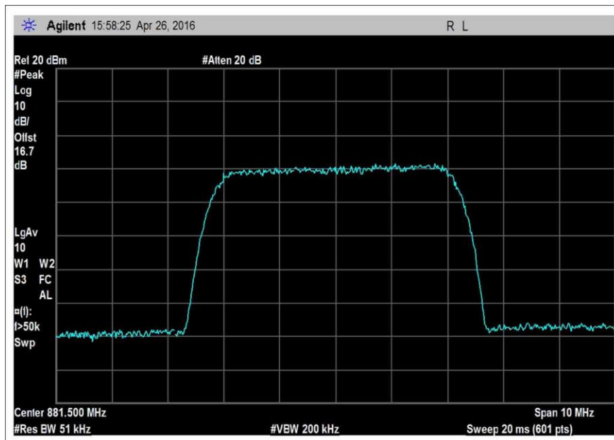
OBW_DL_869-894MHz_WCDMA
