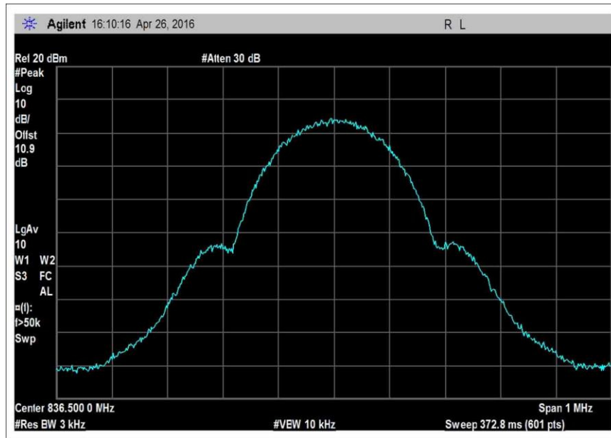
OBW_UL_824-849MHz_GSM
