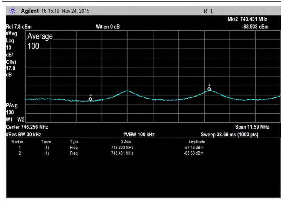
DL-746-757-AWGNR+4
