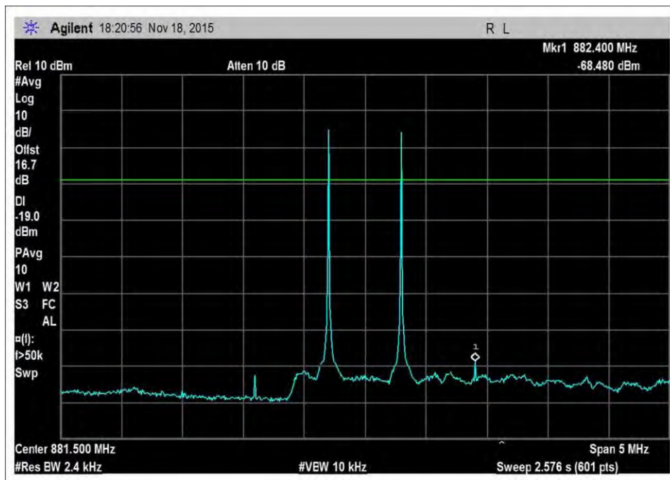
7.4_Intermod_DL_869-894MHz+10dB
