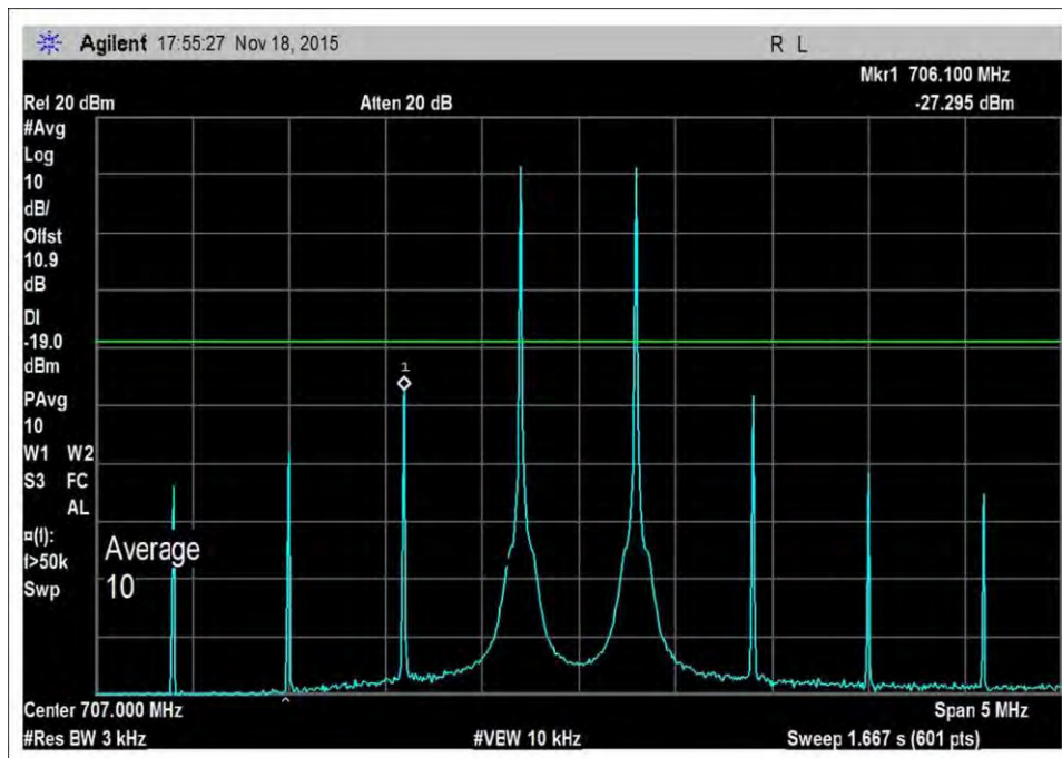
7.4_Intermod_UL_698-716MHz+10dB
