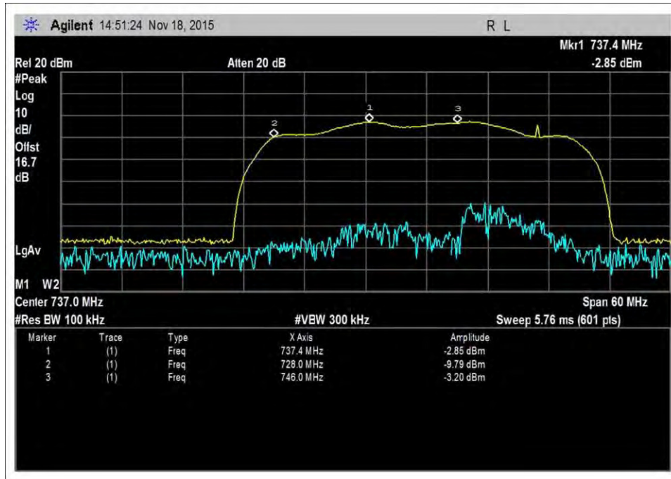
7.1_band verify_DL_728-746MHz_Zoom 2
