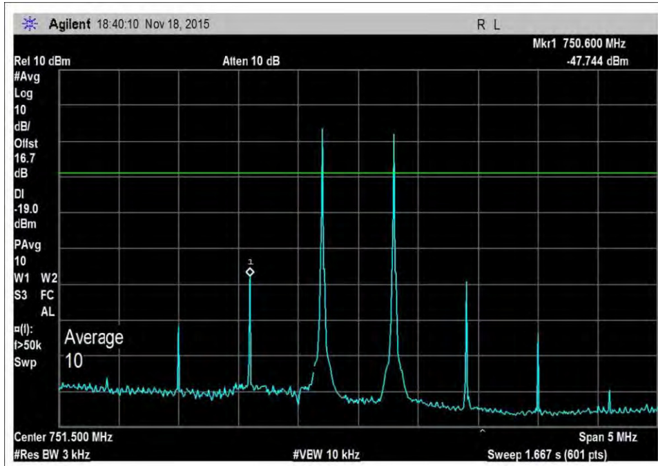
7.4_Intermod_DL_746-757MHz+10dB
