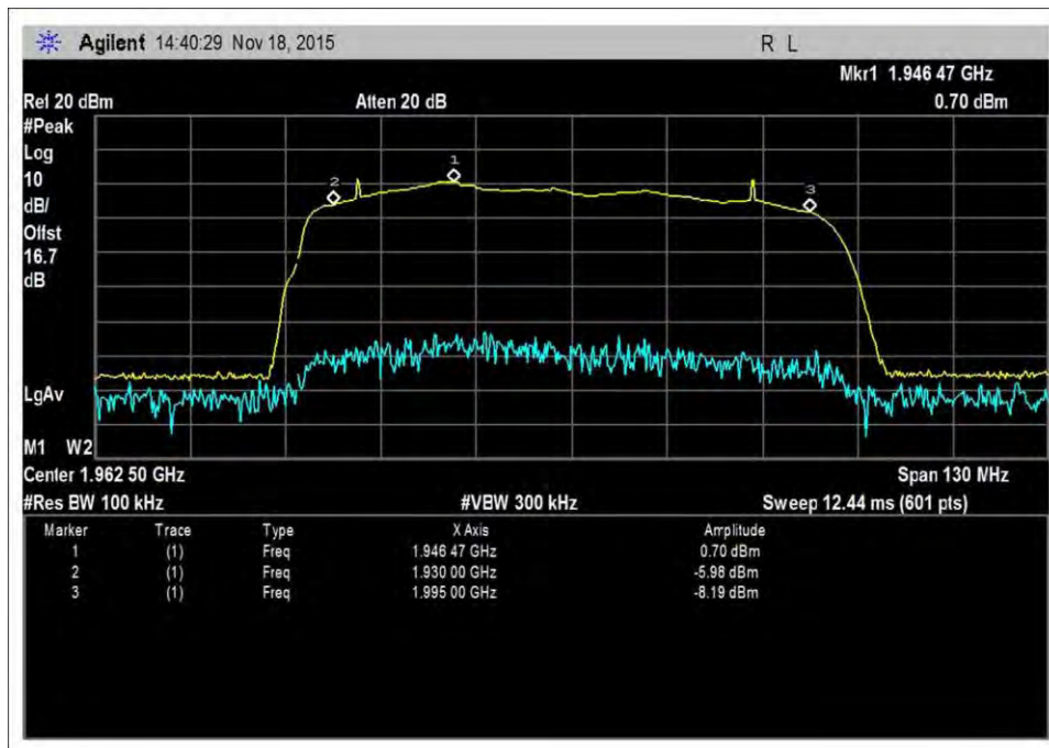
7.1_band verify_DL_1930-1995MHz_3
