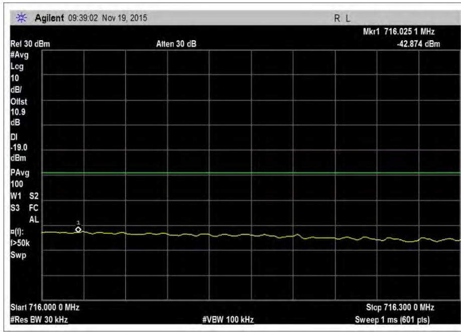
7.5_OBE_UL_698-716MHz_H_Max
