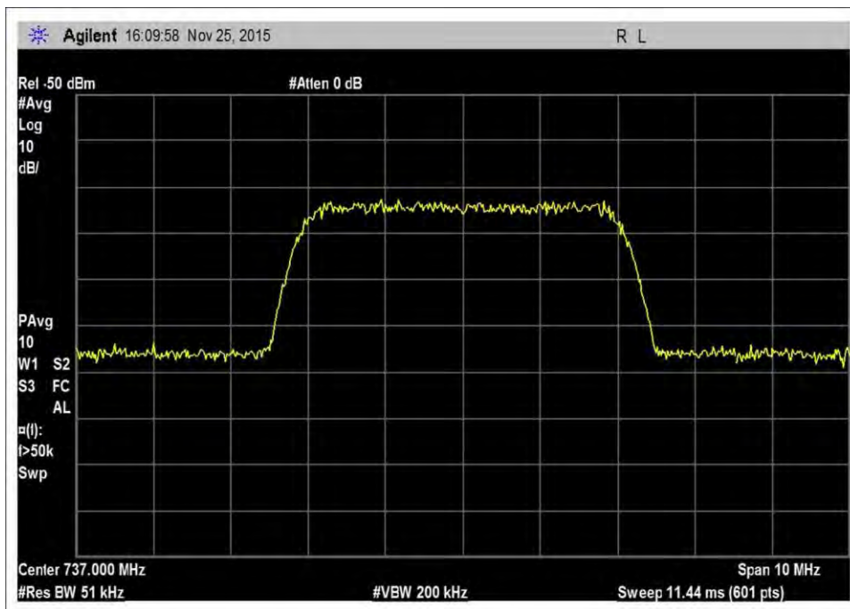
7.10_OBW_DL_728-746MHz_WCDMA
