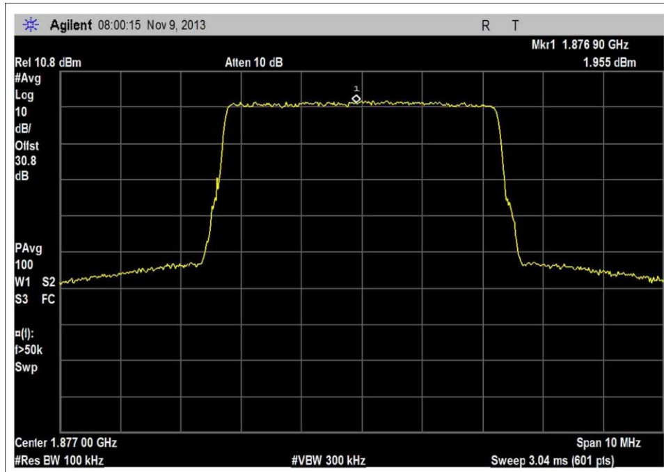
UL 1850-1915MHz, LTE Output
