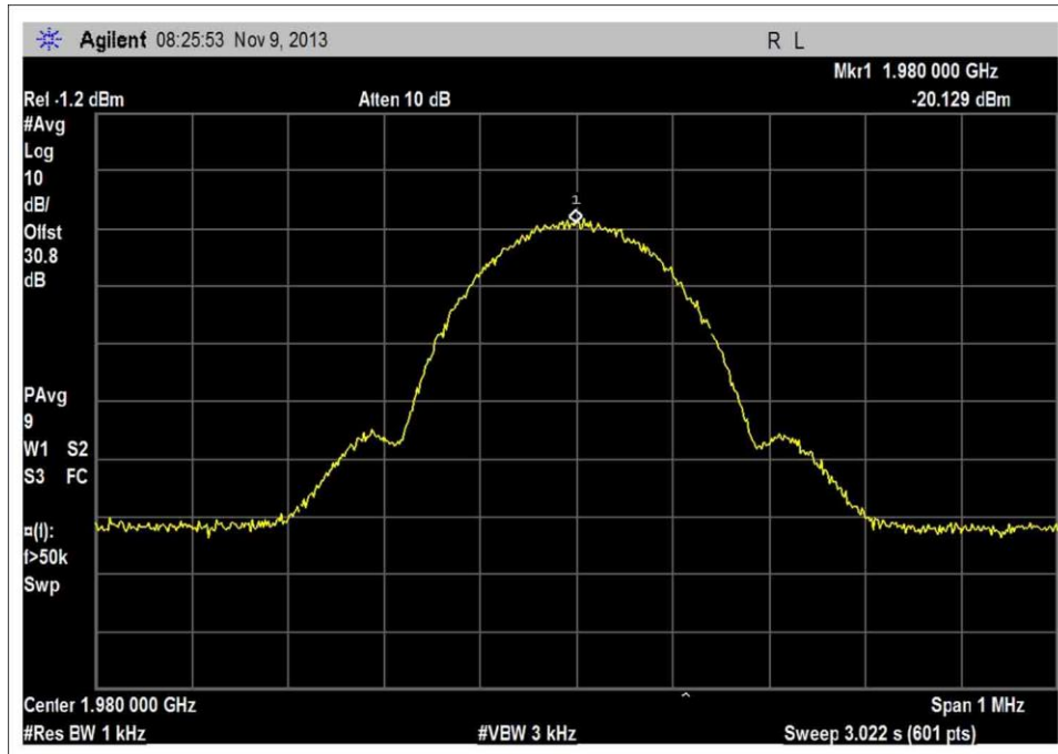
DL 1930-1995MHz, GSM Output
