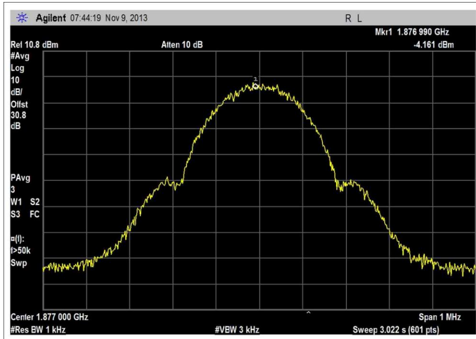
UL 1850-1915MHz, GSM Output
