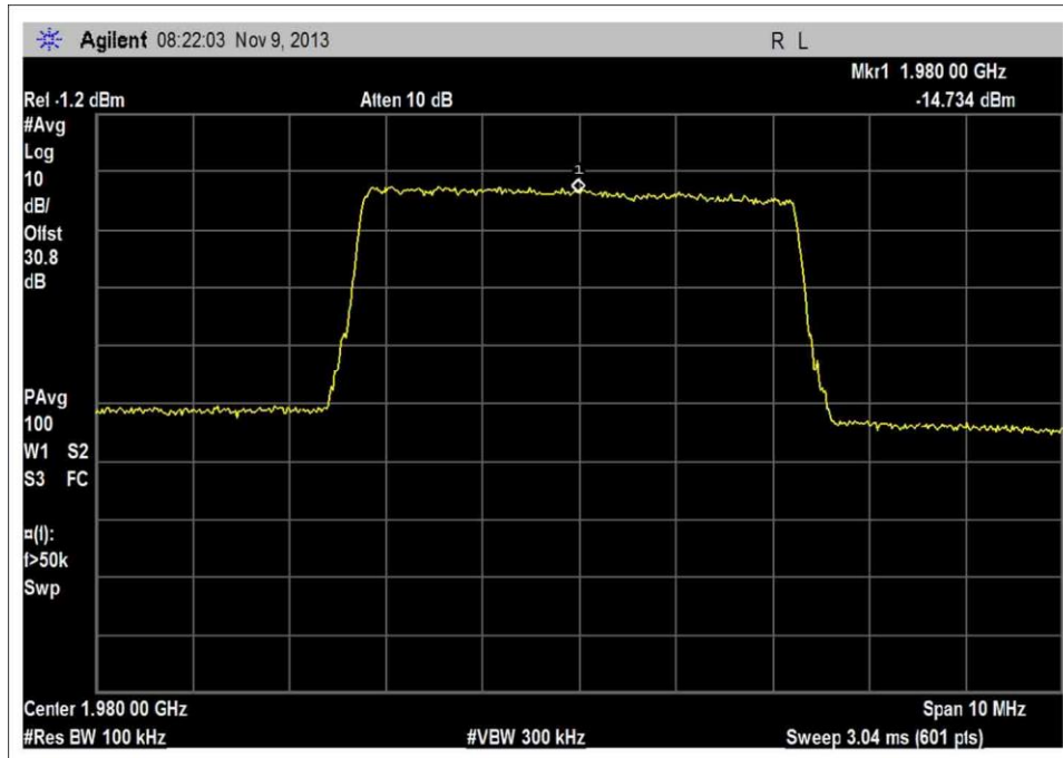
DL 1930-1995MHz, LTE Output
