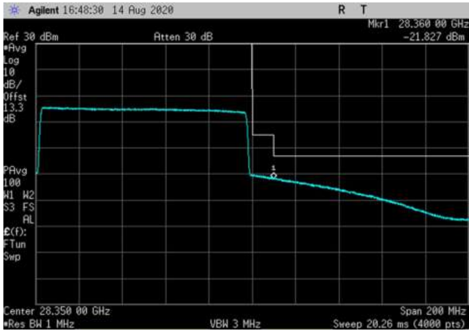
DL_27500-28350_256QAM-100MHz-H-AGC+3-CP OFDM_HC
