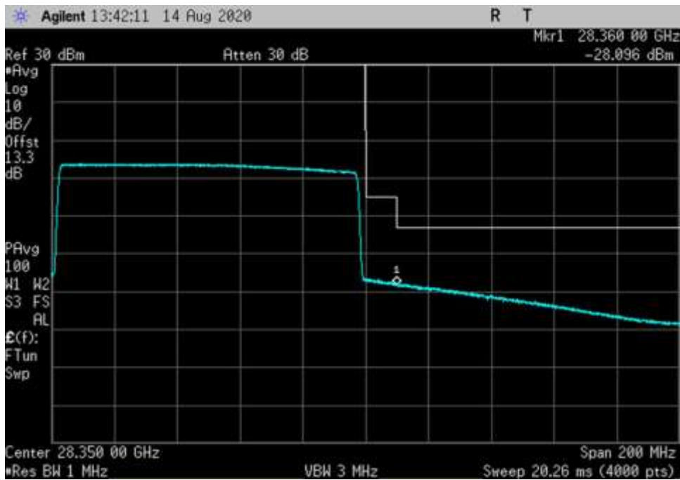
UL_27500-28350-QPSK-100MHz-H-AGC+3-CP OFDM_HC
