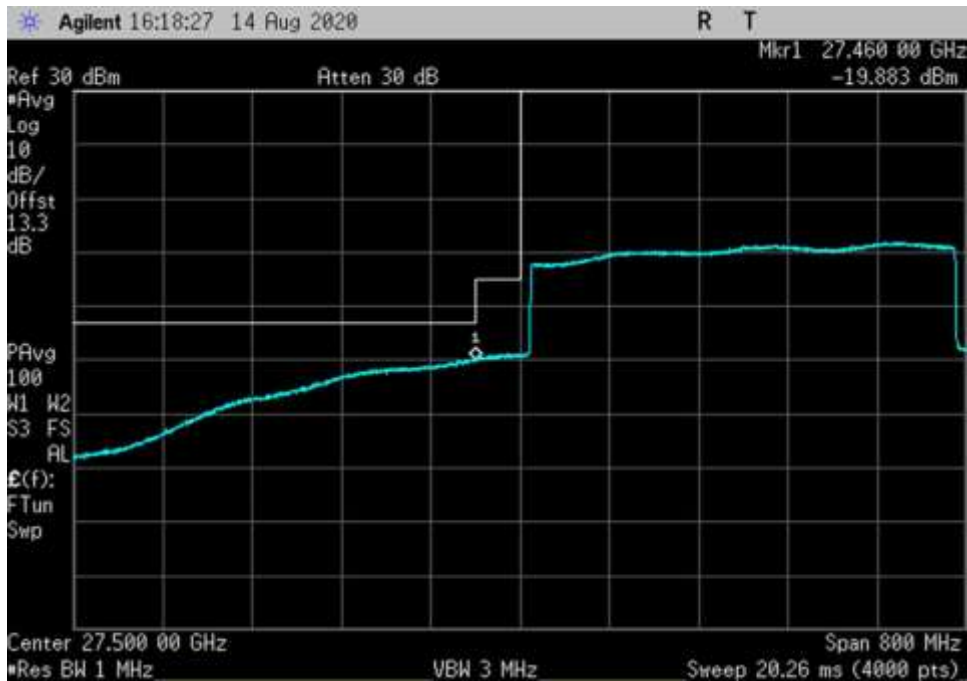
DL_27500-28350_64QAM-400MHz-H-AGC+3-CP OFDM_LC
