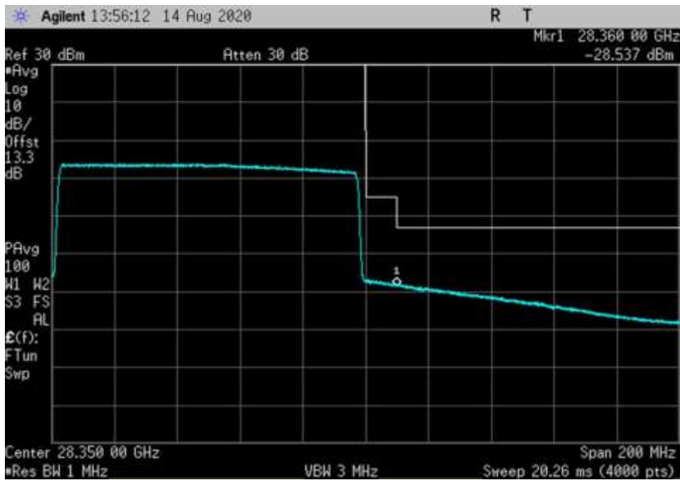
UL_27500-28350-256QAM-100MHz-H-AGC+3-CP OFDM_HC
