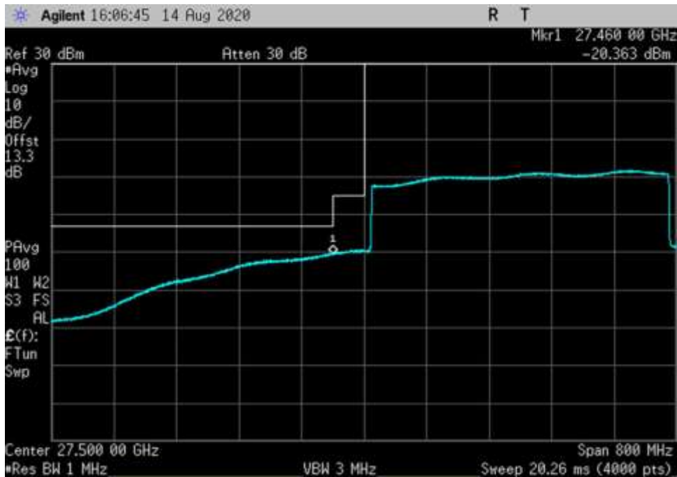
DL_27500-28350_QPSK-400MHz-H-CP OFDM_LC
