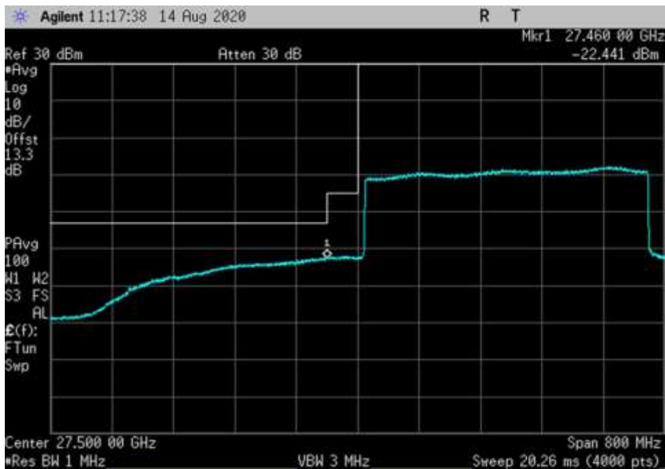
UL_27500-28350-256QAM-400MHz-V-AGC+3-DFT OFDM_LC
