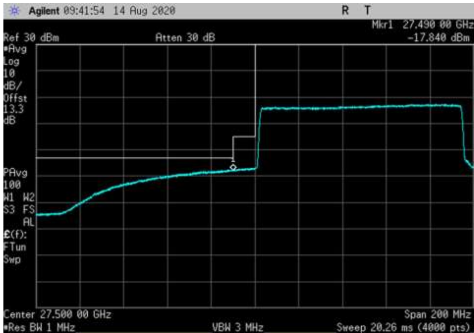
UL_27500-28350-256QAM-100MHz-V- DFT OFDM_LC
