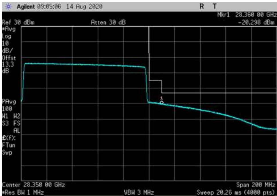
UL_27500-28350-16QAM-100MHz-V-CP OFDM_HC
