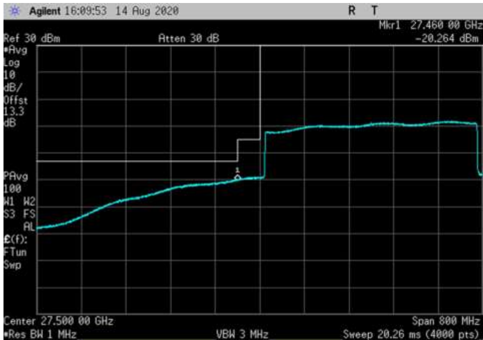
DL_27500-28350_16QAM-400MHz-H-CP OFDM_LC
