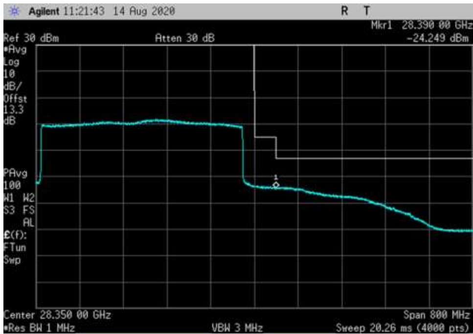
UL_27500-28350-256QAM-400MHz-V-AGC+3-DFT OFDM_HC
