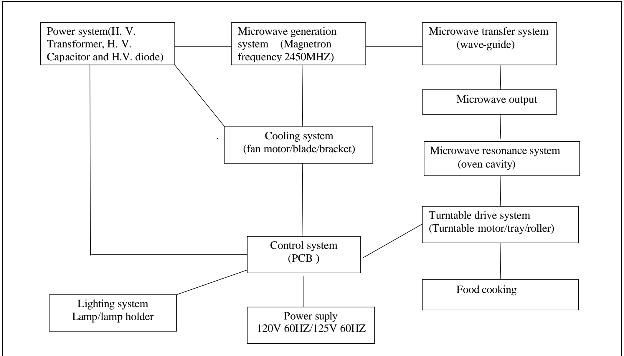
E9025X-Y 产品方框图
