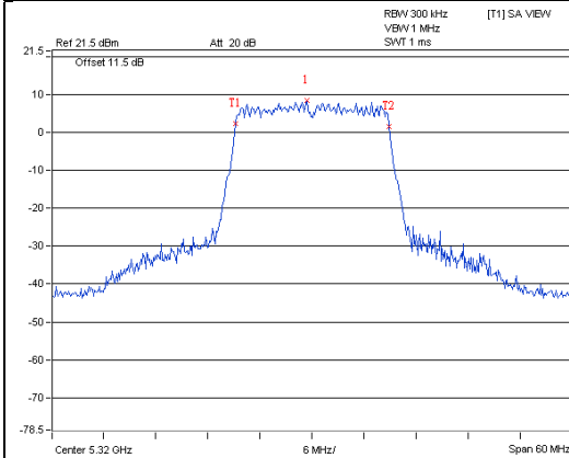
11ac (20MHz) 2S3T TxBF CH64 Chain3
