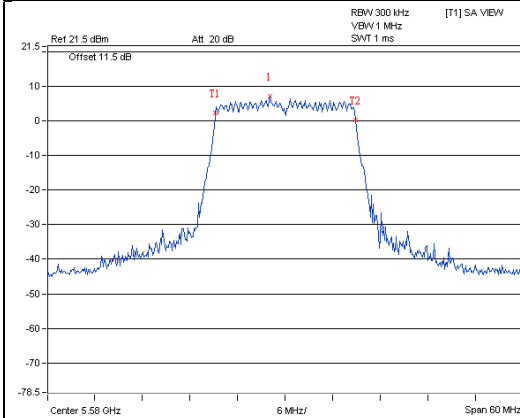
11ac (20MHz) 2S3T TxBF CH116 Chain3
