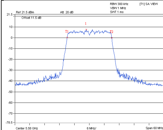
11ac (20MHz) 2S3T TxBF CH116 Chain3
