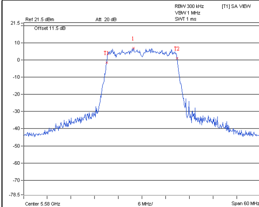
11ac (20MHz) 2S3T TxBF CH116 Chain2
