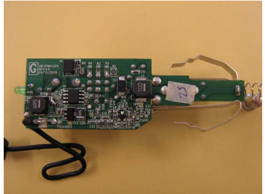
PCBA Bottom
