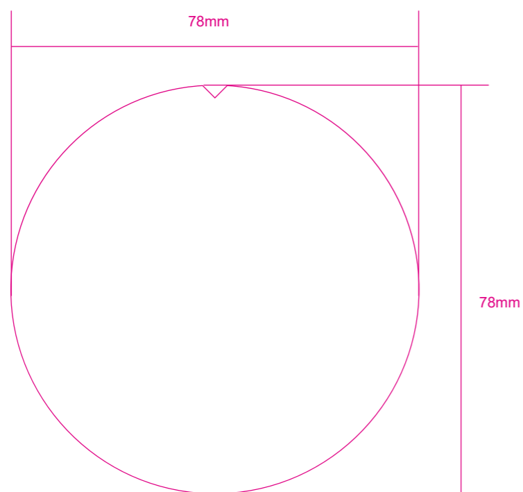
尺寸圖 outline dimension
