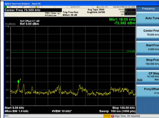
9 KHz – 150 KHz
