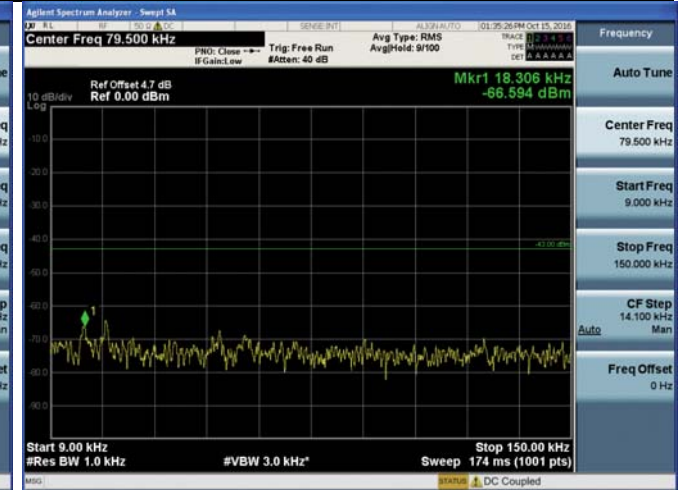
9 KHz – 150 KHz
