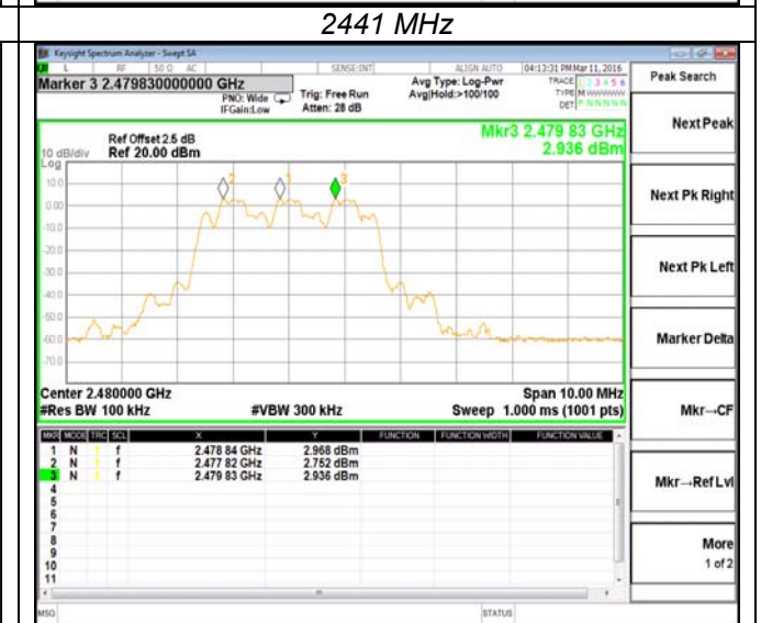
2480 MHz
