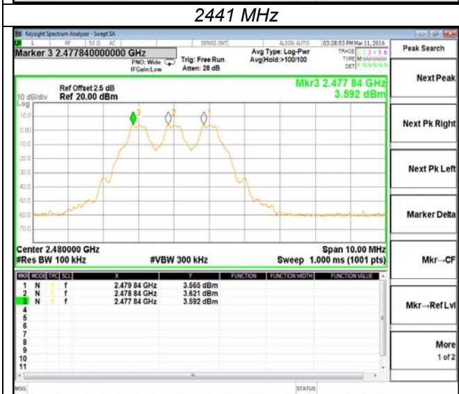
2480 MHz
