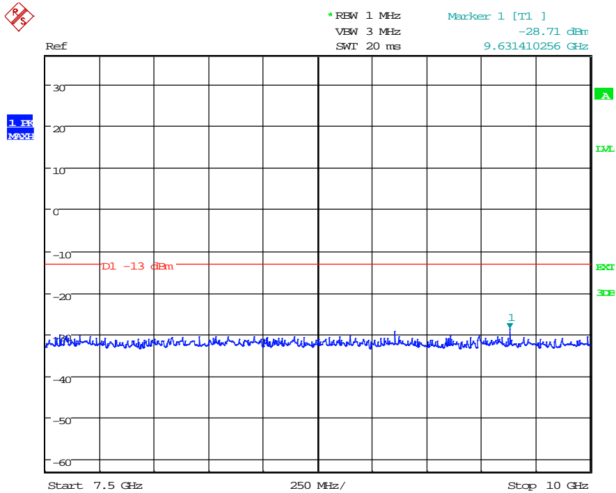
(Plot 4.6.1 D5: Idle WCDMA Band II)
