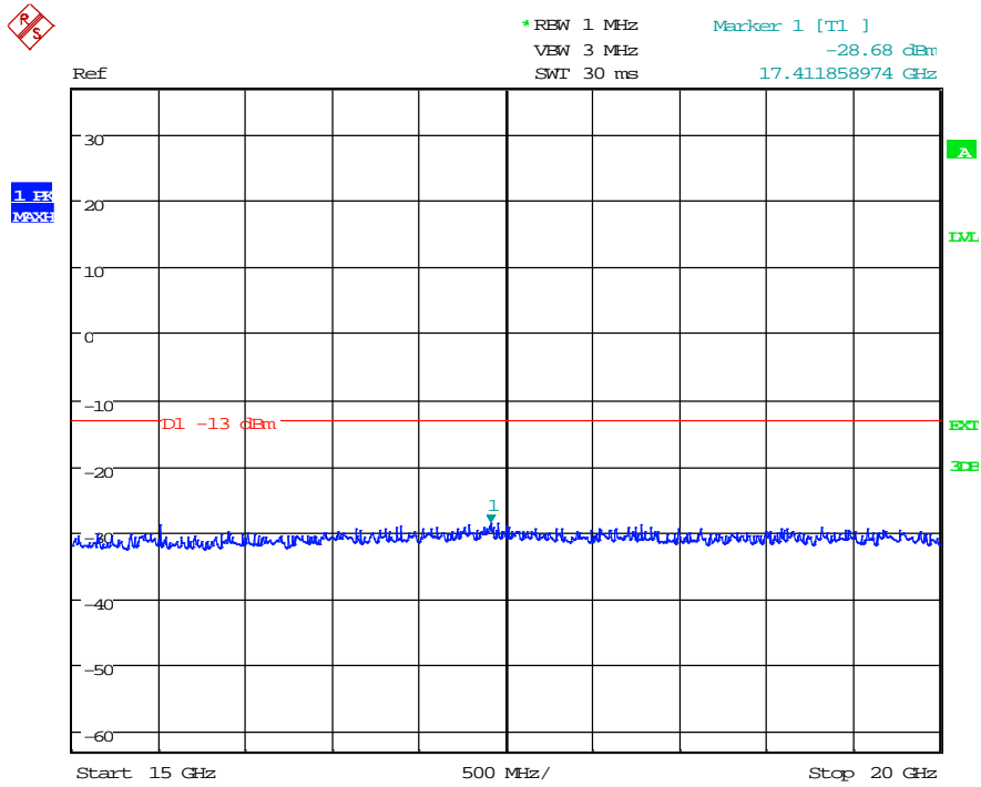
(Plot 4.6.1 D7: Idle WCDMA Band II)
