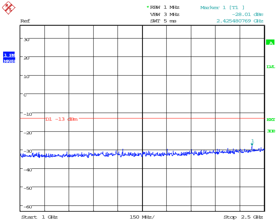
(Plot 4.6.1 D3: Idle WCDMA Band II)
