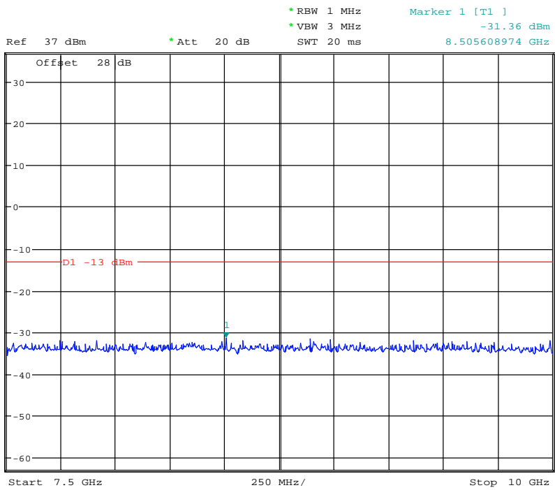
(Plot 4.6.1 D5: Idle WCDMA Band II)
