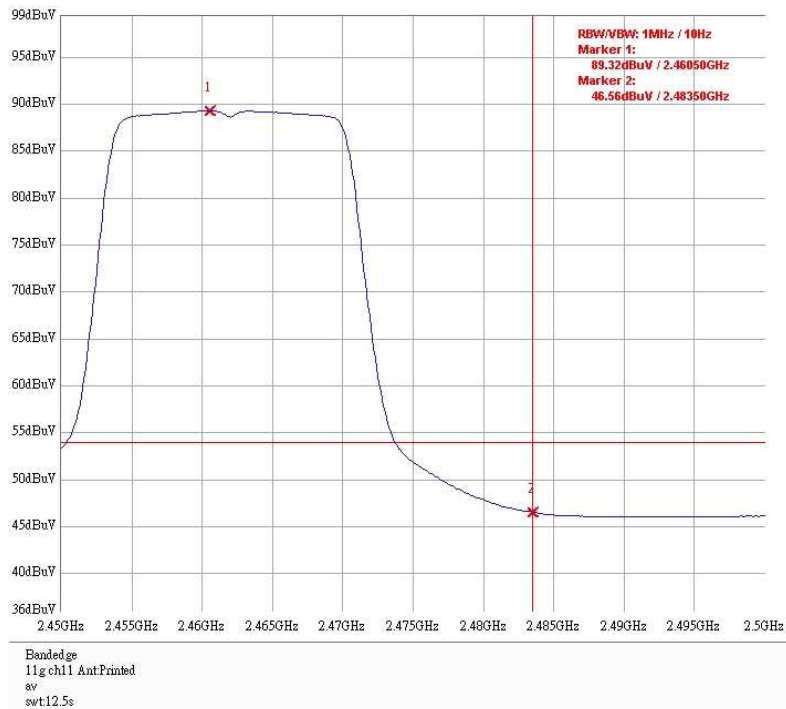
Band edge @ 802.11g mode channel 11 AV
