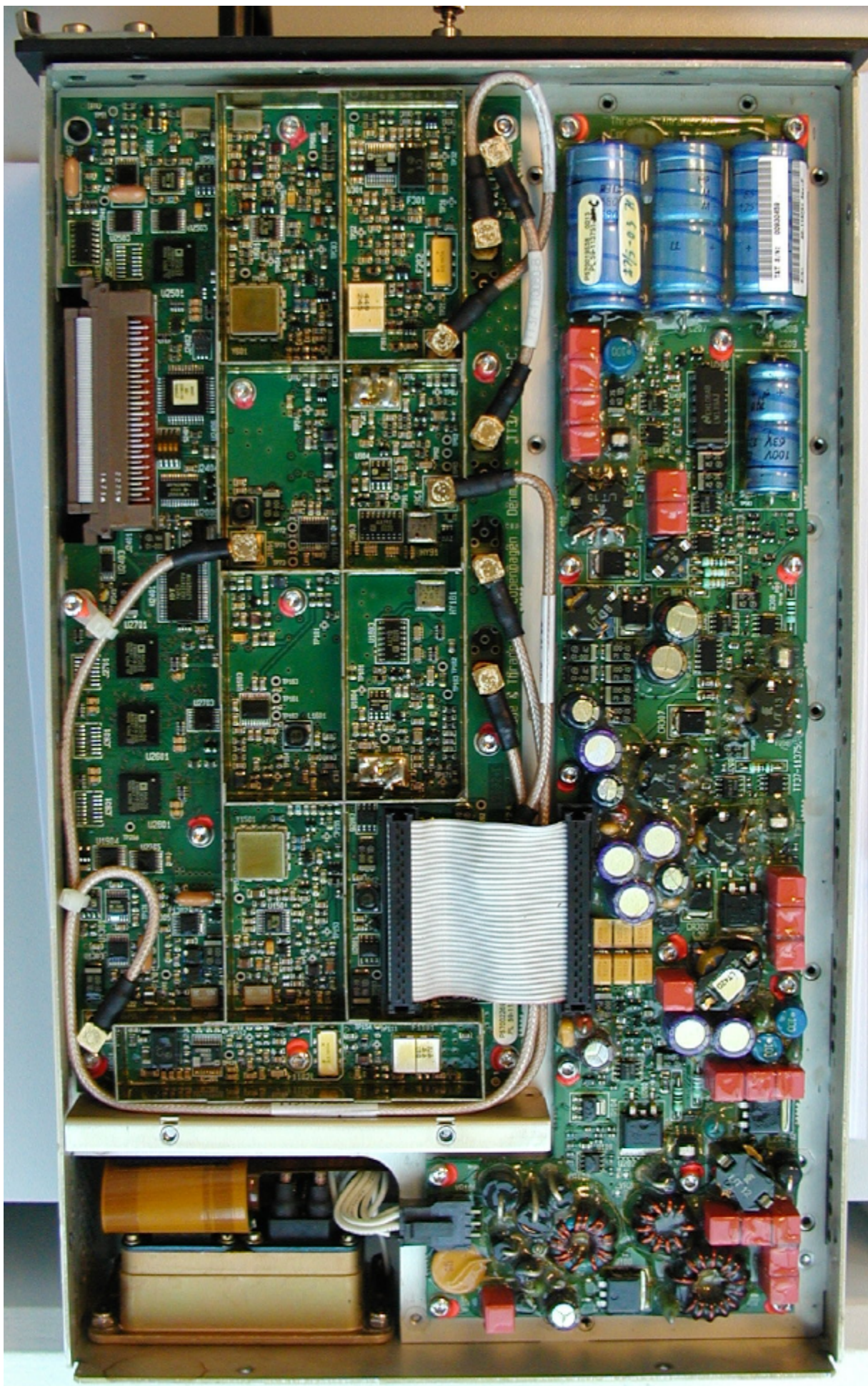
TT-5035A SDU Right: TT93-113892 Left: TT93-113751
