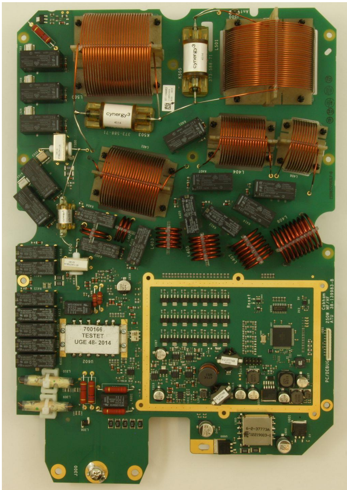
ATU module front side
