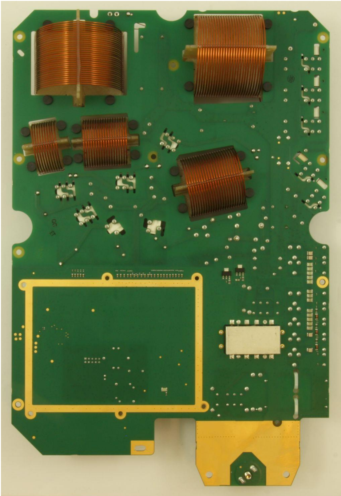
ATU module back side
