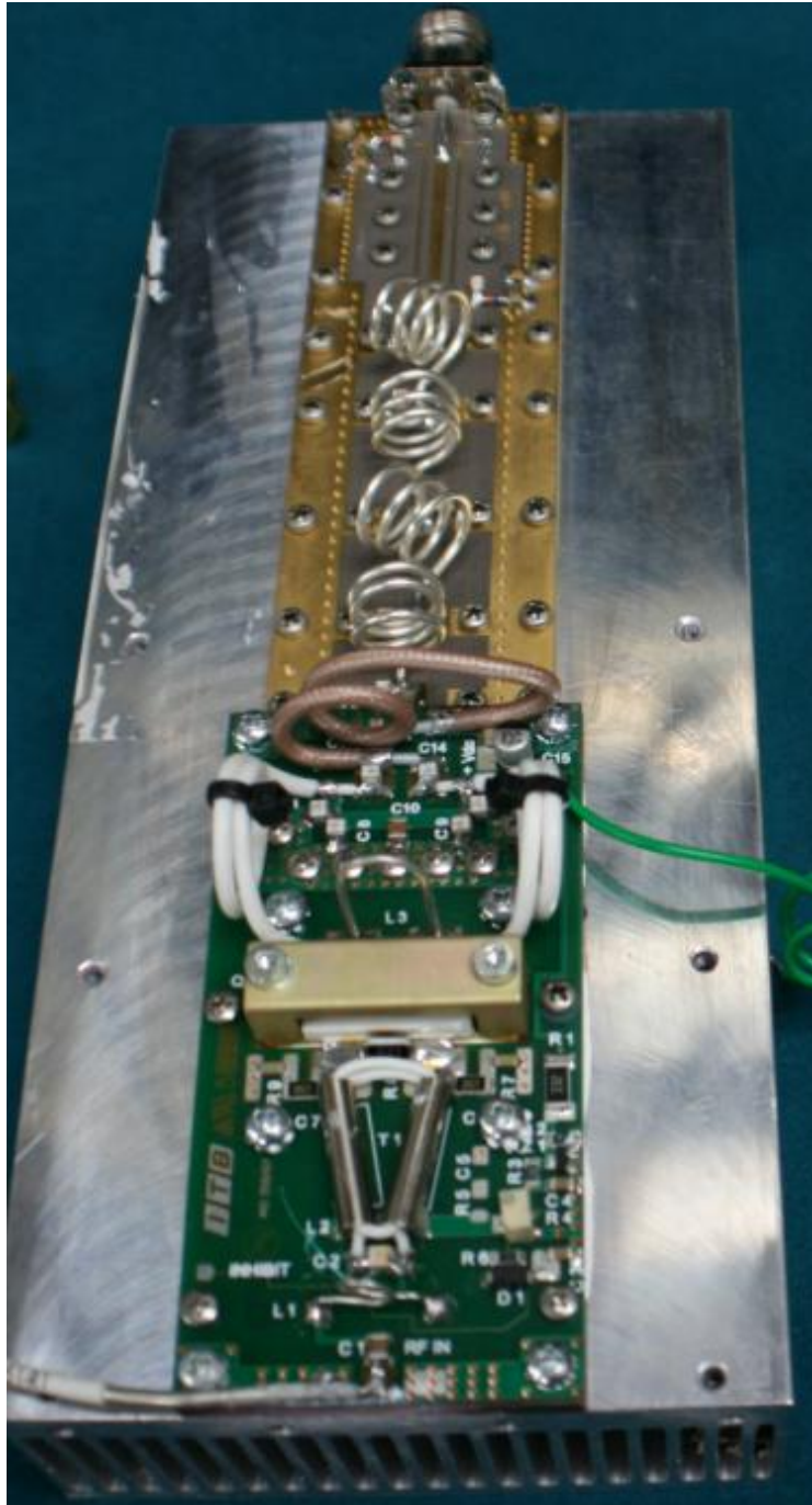
RF MODULE
