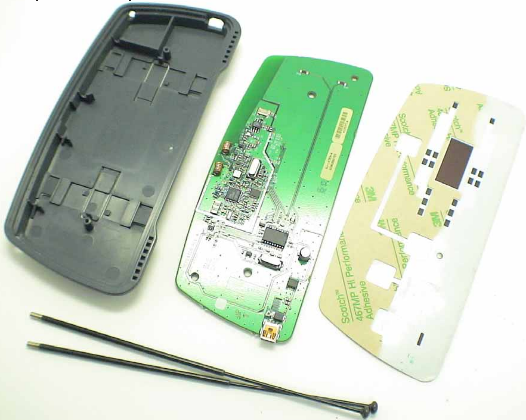
DUT apart (top)
