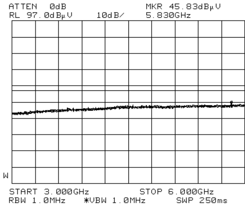
Channel 6 @ 802.11g (Turbo) 108Mbps (3GHz-6GHz)
