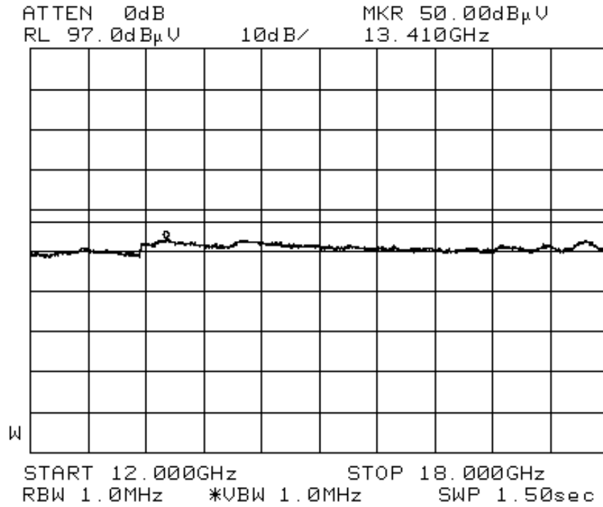
Channel 6 @ 802.11g (Turbo) 108Mbps (12GHz-18GHz)
