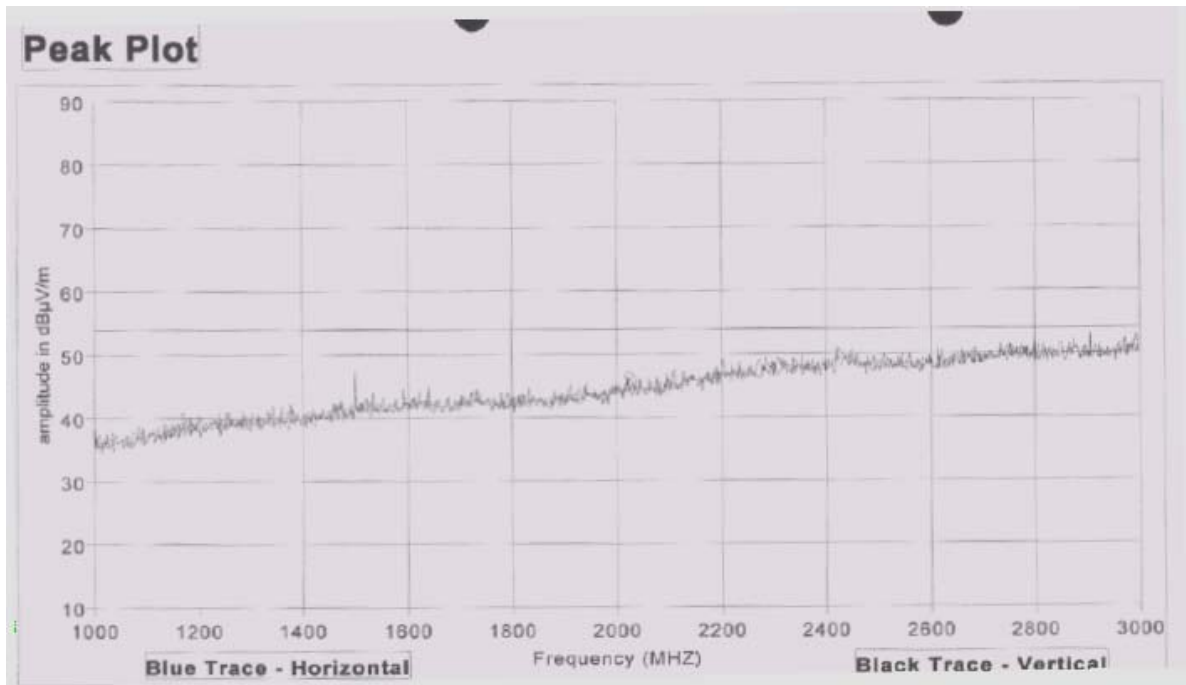
Channel 6 @ 802.11g (Turbo) 108Mbps (1GHz-3GHz)
