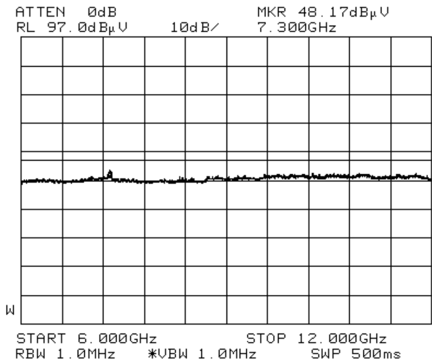
Channel 6 @ 802.11g (Turbo) 108Mbps (6GHz-12GHz)
