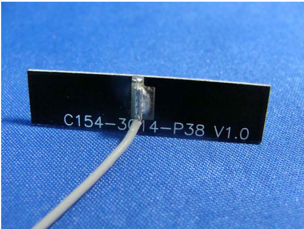
(6) EUT Photo (REF-02-P118-70B-150)
