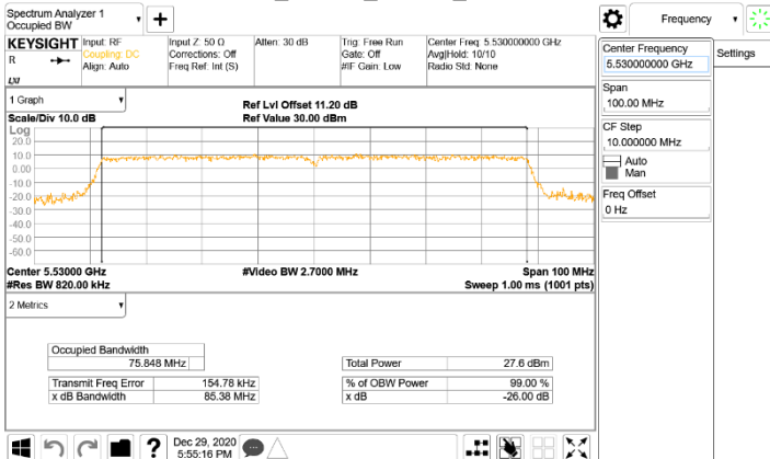
802.11ac_80MHz_Chain2_5530MHz
