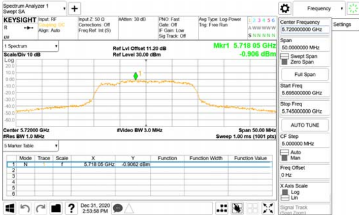
802.11n_20MHz_Chain2_5720MHz_UNII 3
