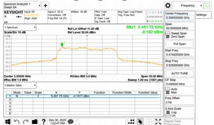
802.11n_20MHz_Chain3_5500MHz
