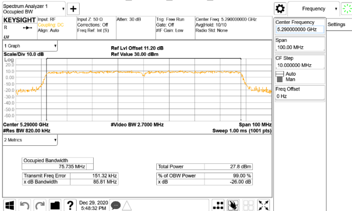
802.11ac_80MHz_Chain2_5290MHz
