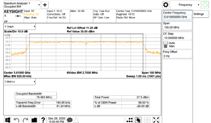
802.11ac_80MHz_Chain2_5610MHz
