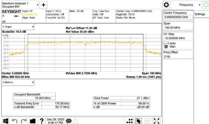
802.11ac_80MHz_Chain1_5690MHz
