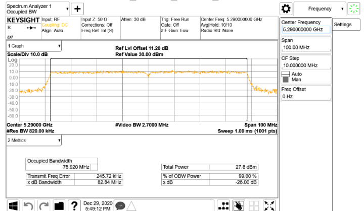
802.11ac_80MHz_Chain3_5290MHz
