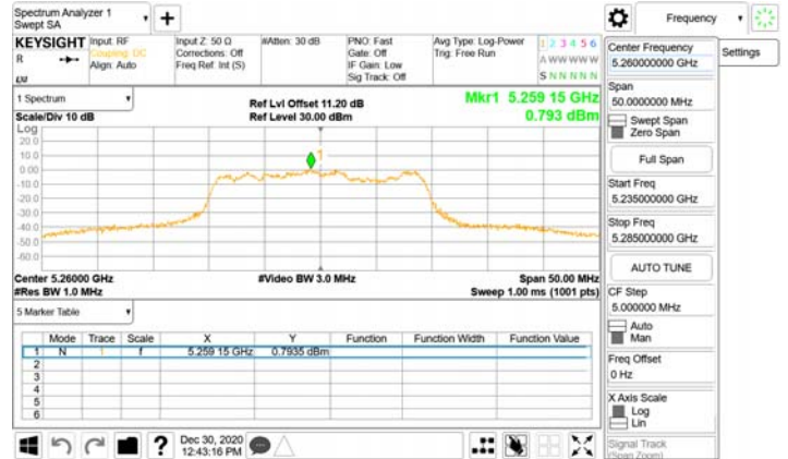
802.11n_20MHz_Chain1_5260MHz
