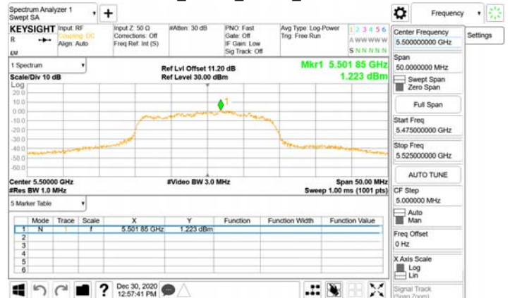
802.11n_20MHz_Chain0_5500MHz
