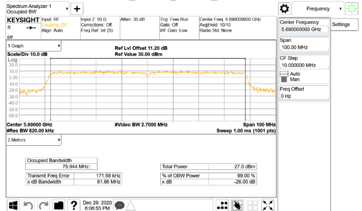
802.11ac_80MHz_Chain2_5690MHz
