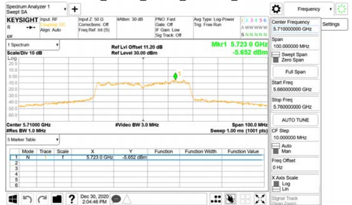
802.11n_40MHz_Chain1_5710MHz_UNII 3
