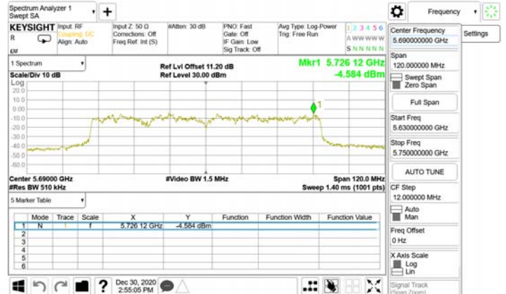
802.11ac_80MHz_Chain3_5690MHz_UNII 3
