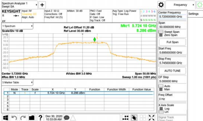
802.11a_20MHz_Chain1_5720MHz_UNII 3
