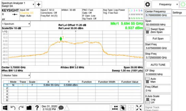
802.11n_20MHz_Chain0_5700MHz
