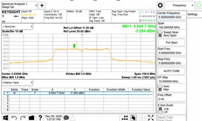
802.11n_40MHz_Chain1_5550MHz
