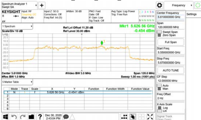
802.11ac_80MHz_Chain2_5610MHz
