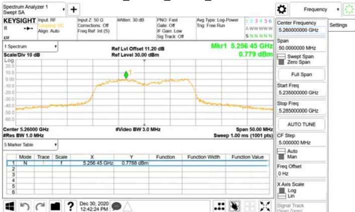
802.11n_20MHz_Chain0_5260MHz
