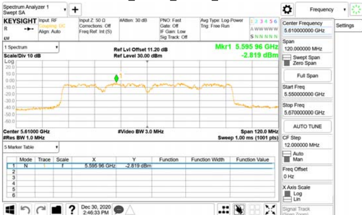
802.11ac_80MHz_Chain3_5610MHz
