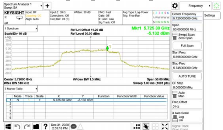
802.11n_20MHz_Chain1_5720MHz_UNII 3
