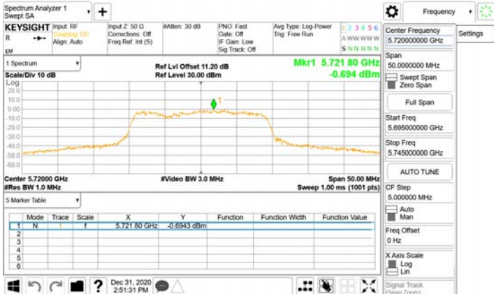
802.11n_20MHz_Chain0_5720MHz_UNII 2C
