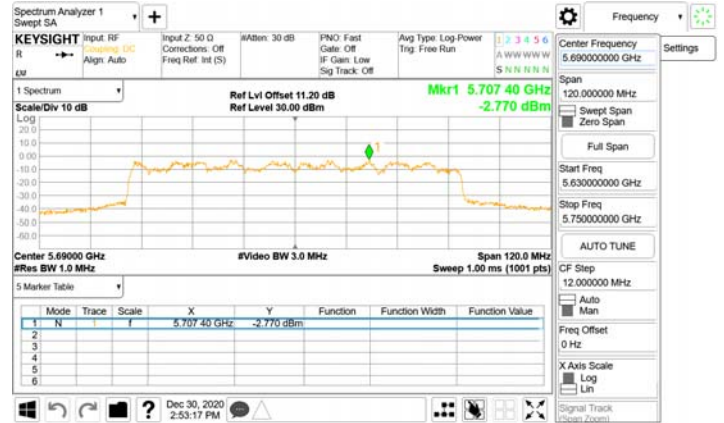
802.11ac_80MHz_Chain2_5690MHz_UNII 3
