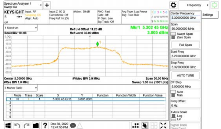
802.11n_20MHz_Chain1_5300MHz
