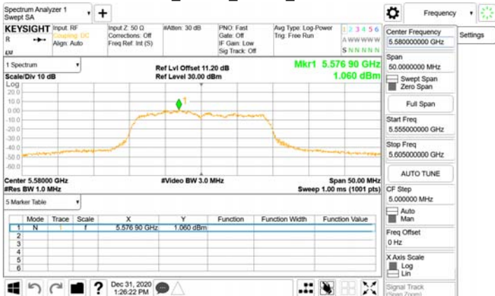
802.11n_20MHz_Chain1_5580MHz
