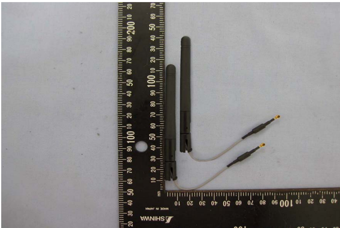
Dipole Antenna / 6602113051-090
