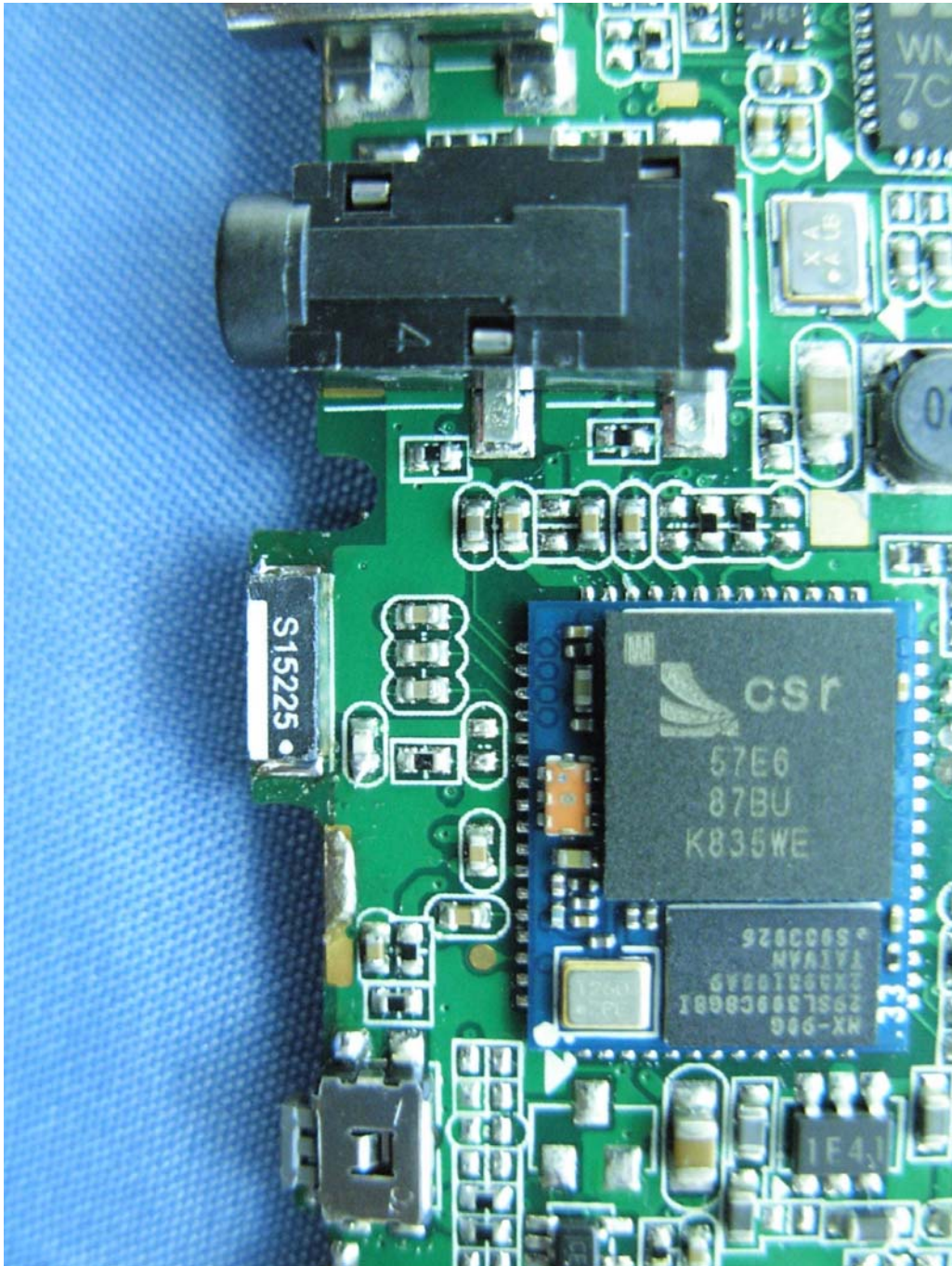
(18) EUT Photo
