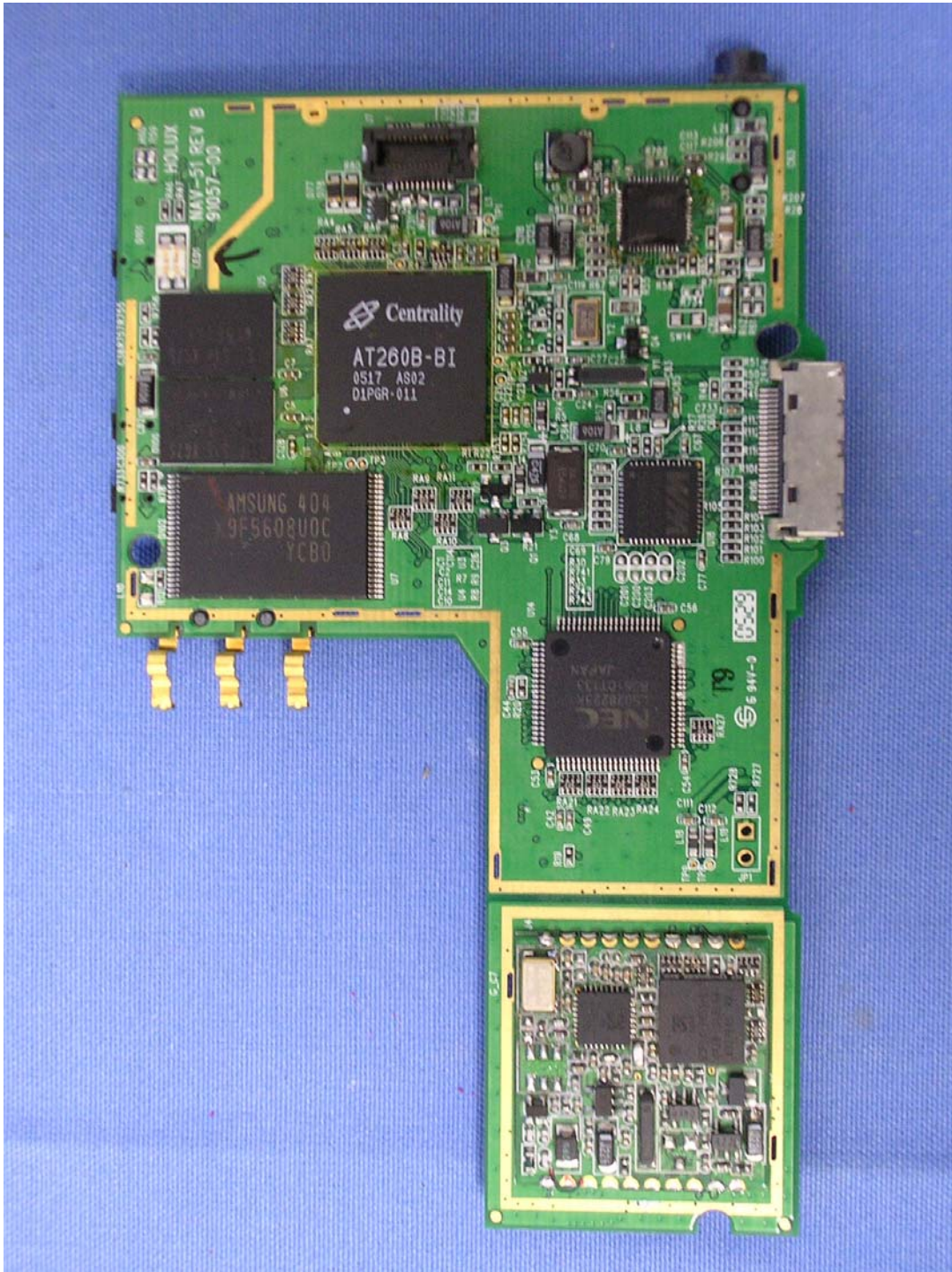
(6) EUT Photo
