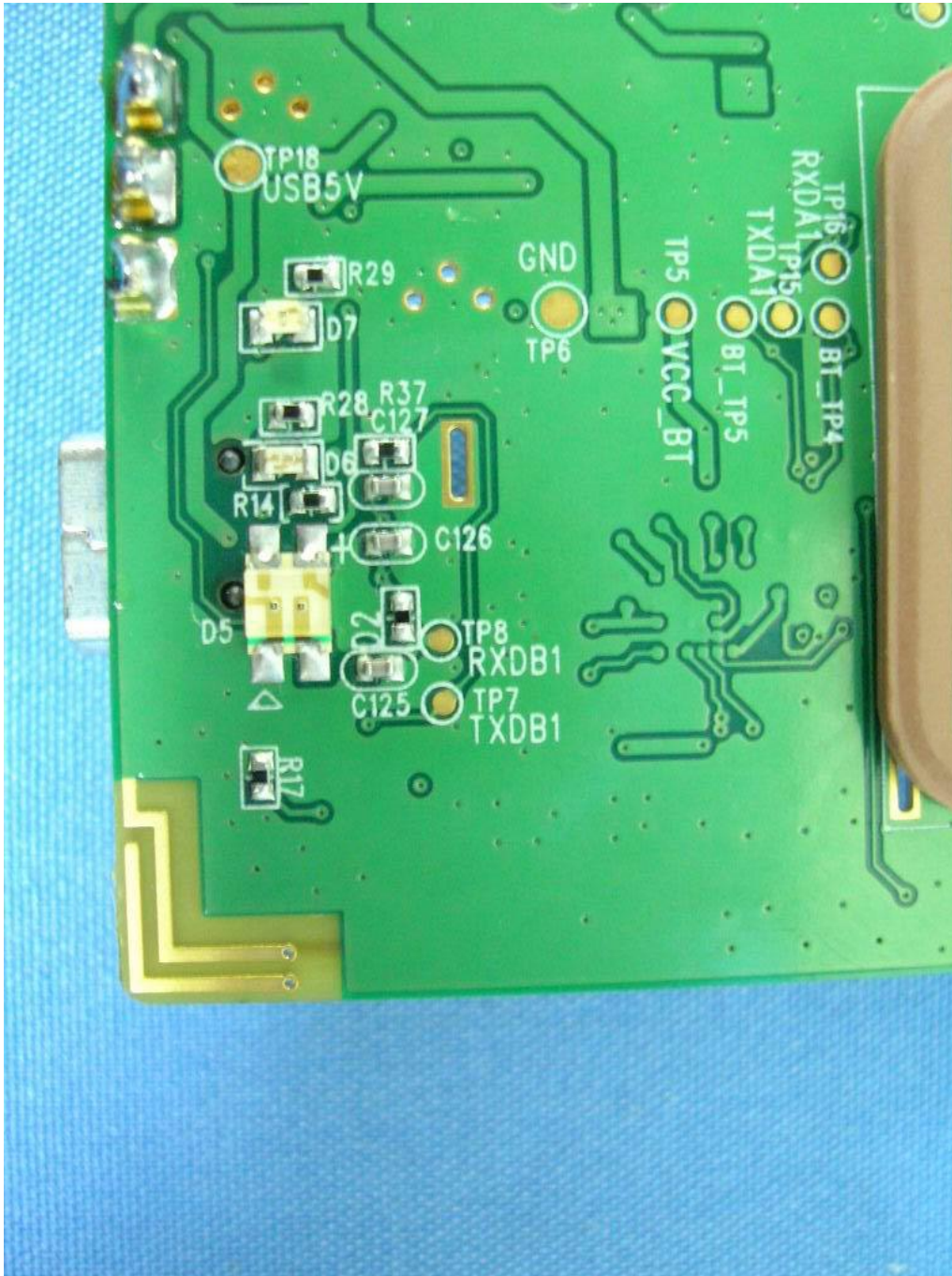
(16) EUT Photo
