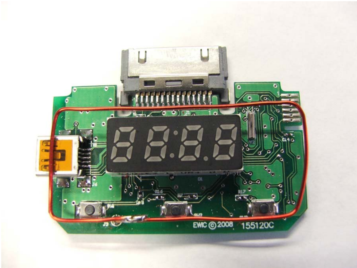
FCC ID: 178065-00 PCB TOP
