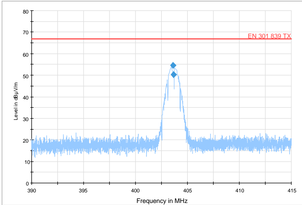
EN 301 839 TX Power
