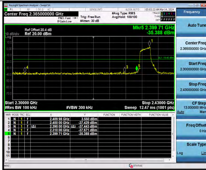
11AX20MIMO Ant1 Low 2412 242Tone RU61
