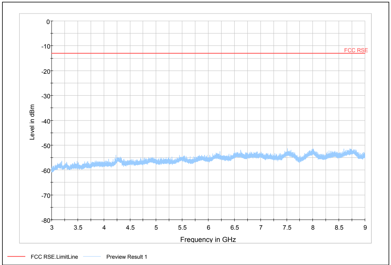
GSM 850 128 Channel 3GHz~9GHz
