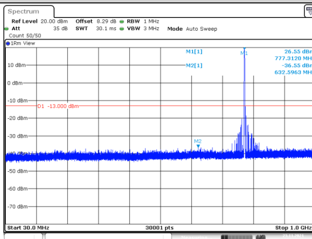
Band13-5MHz-QPSK-23205-1-0-Low-30-1000--36.55-PASS
