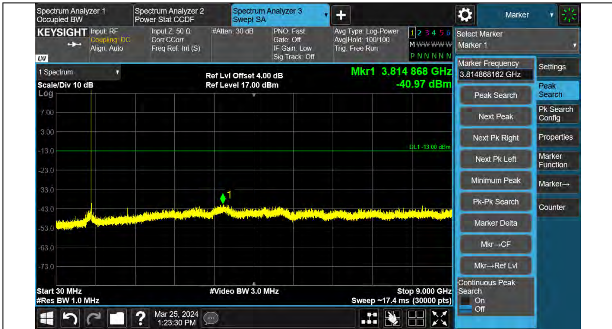
Band26-QPSK-15KHz-26692-1RB#0
