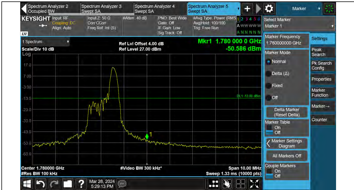
Band66-20MHz-QPSK-132572-6RB#0
