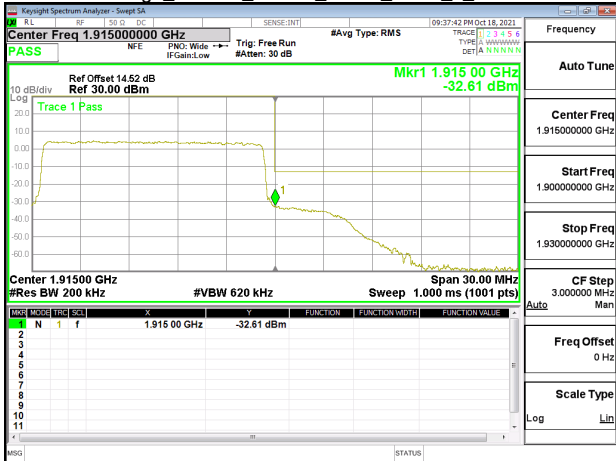
Band Edge_Band25_20MHz_QPSK_RB1_0_CH26140
