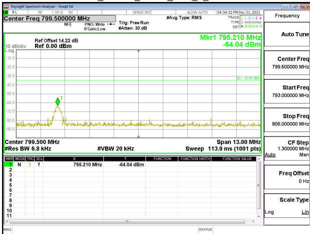
Band13_10MHz_QPSK_RB1_49_CH23230
