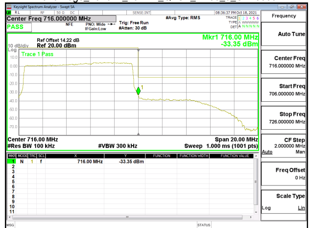
Band Edge_Band17_10MHz_QPSK_RB50_0_CH23800
