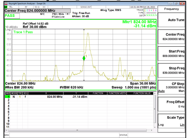
Band Edge_Band26_15MHz_QPSK_RB1_74_CH26965
