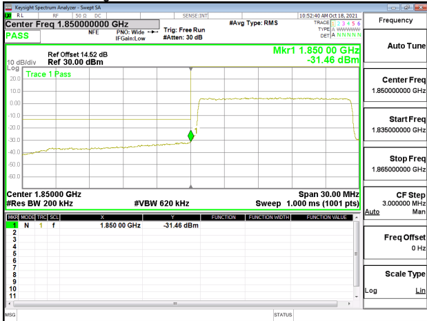
Band Edge_Band2_15MHz_QPSK_RB75_0_CH19125
