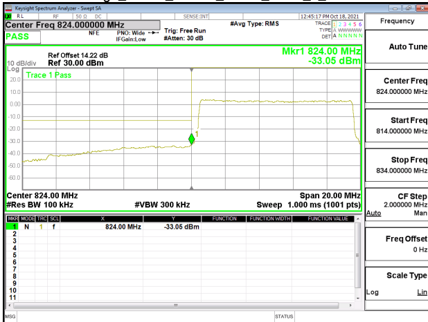
Band Edge_Band5_10MHz_QPSK_RB50_0_CH20450
