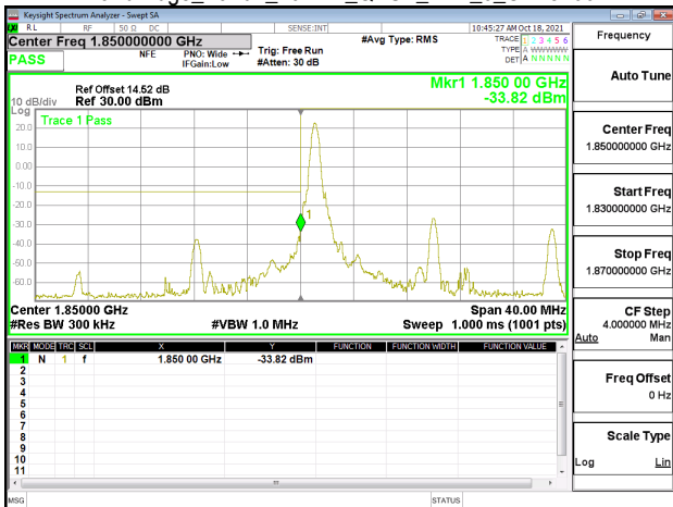
Band Edge_Band2_20MHz_QPSK_RB1_0_CH18700
