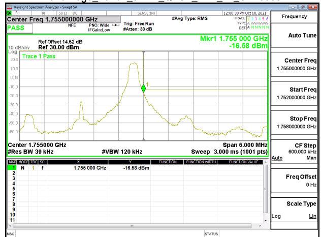
Band Edge_Band4_3MHz_QPSK_RB1_14_CH20385
