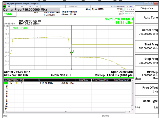
Band Edge_Band12_10MHz_QPSK_RB50_0_CH23130
