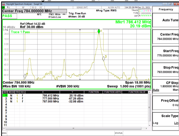
Band Edge_Band13_10MHz_QPSK_RB50_0_CH23230
