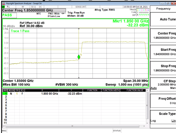
Band Edge_Band2_10MHz_QPSK_RB50_0_CH18650
