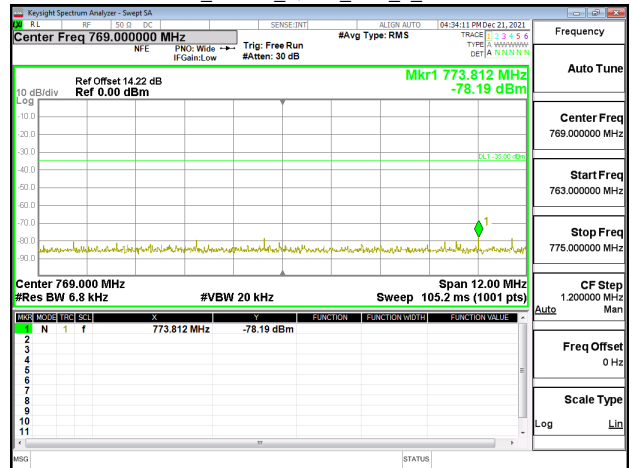
Band13_10MHz_QPSK_RB1_49_CH23230
