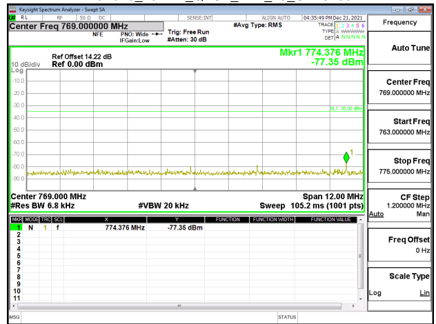
Band13_10MHz_QPSK_RB50_0_CH23230
