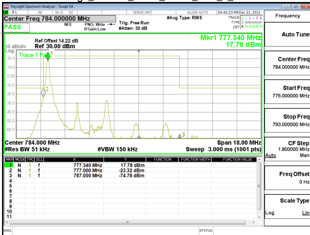
Band Edge_Band13_5MHz_QPSK_RB1_24_CH23255
