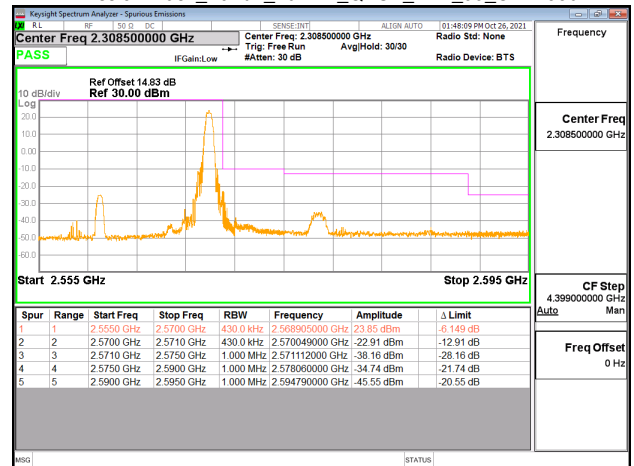
Emission Mask_Band7_20MHz_QPSK_RB1_99_CH21350
