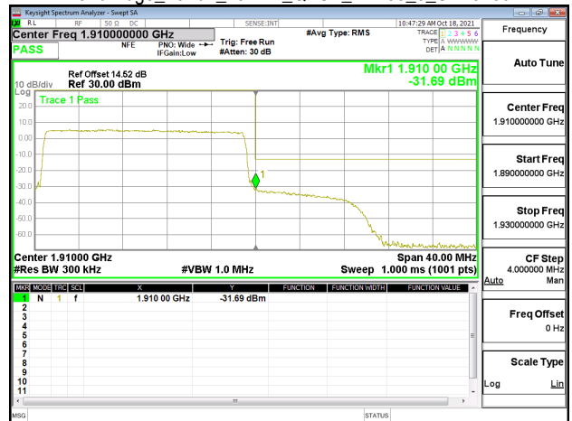
Band Edge_Band2_20MHz_QPSK_RB100_0_CH19100
