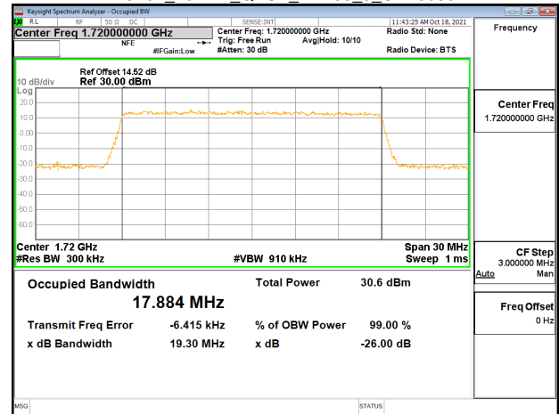
Band4_20MHz_QPSK_RB100_0_CH20175
