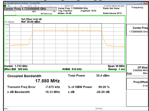
Band4_20MHz_QPSK_RB100_0_CH20300
