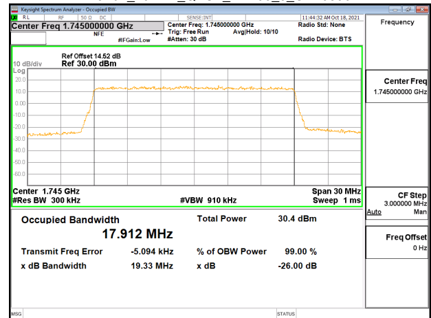
Band4_20MHz_QPSK_RB100_0_CH20300
