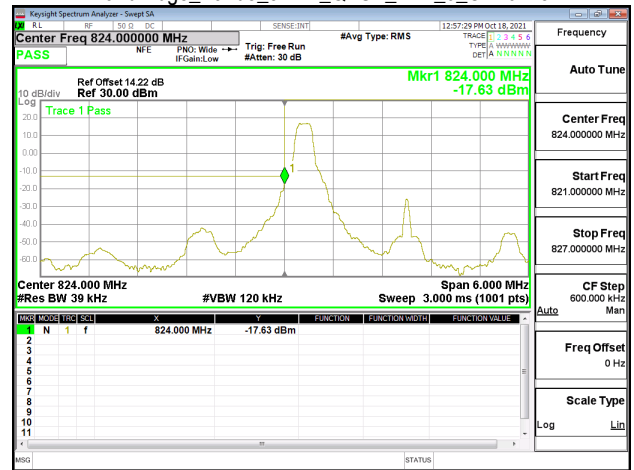
Band Edge_Band5_3MHz_QPSK_RB1_14_CH20635
