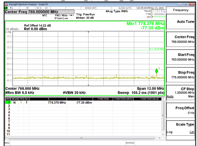
Band13_10MHz_QPSK_RB50_0_CH23230
