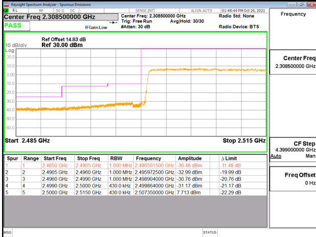
Emission Mask_Band7_20MHz_QPSK_RB100_0_CH21350
