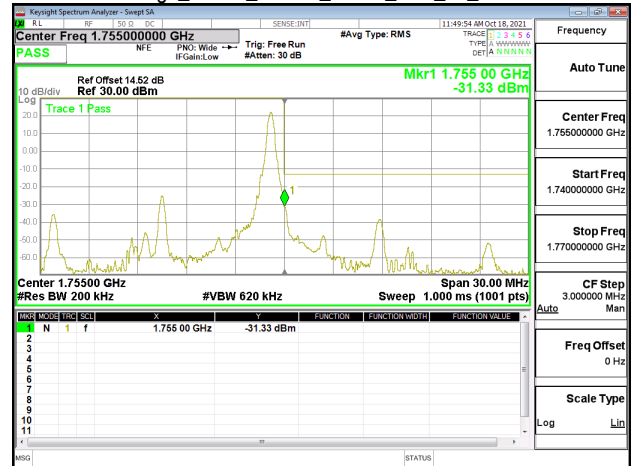
Band Edge_Band4_15MHz_QPSK_RB1_74_CH20325
