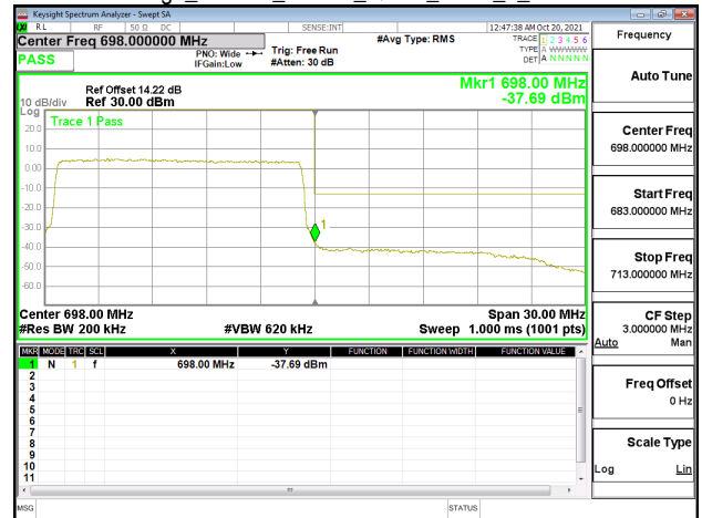
Band Edge_Band71_20MHz_QPSK_RB1_0_CH133222
