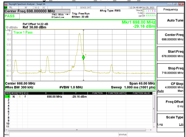
Band Edge_Band71_20MHz_QPSK_RB1_99_CH133372
