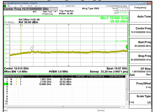
Band2_20MHz_QPSK_RB1_0_CH18900
