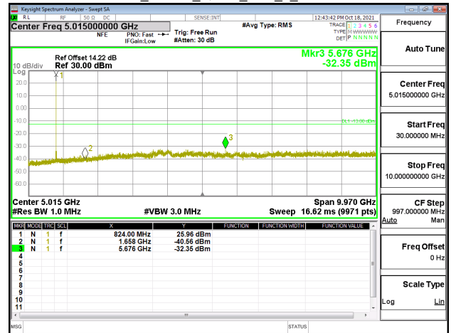
Band5_10MHz_QPSK_RB1_0_CH20525
