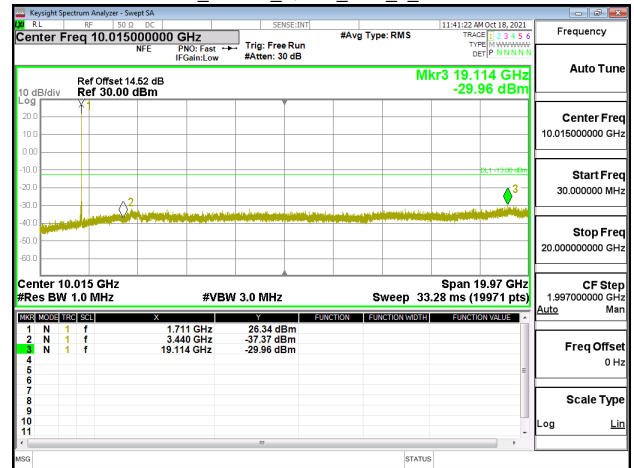
Band4_20MHz_QPSK_RB1_0_CH20175
