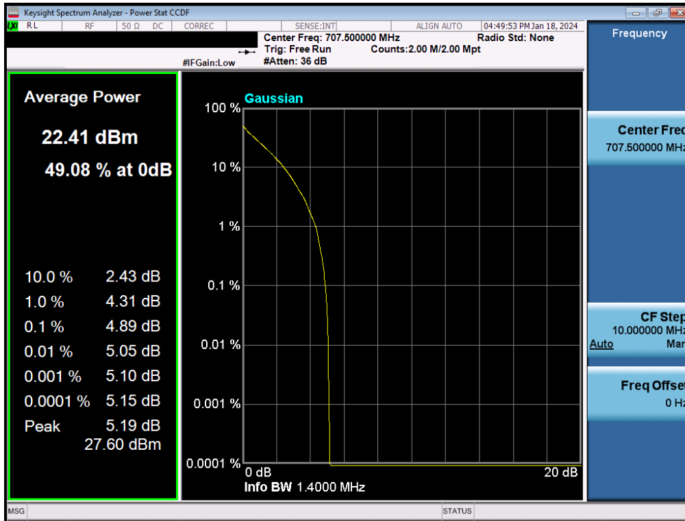
Plot 7-104. PAR Plot (LTE Band 12 - 1.4MHz QPSK - Full RB)
