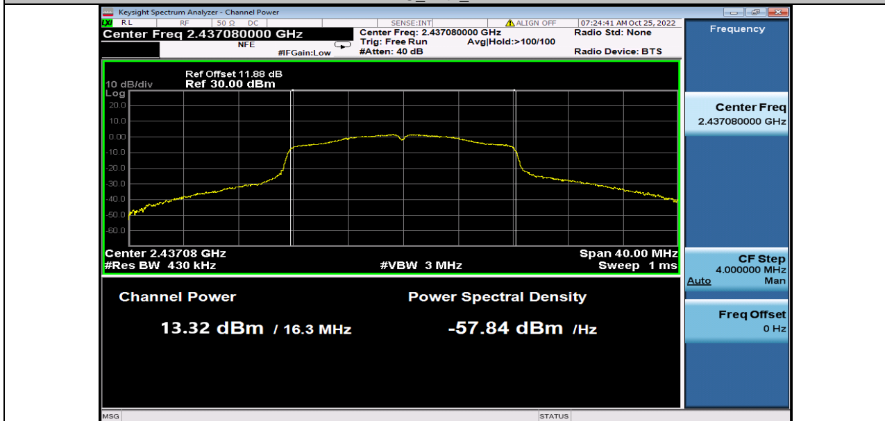
11G_Ant1_2437
