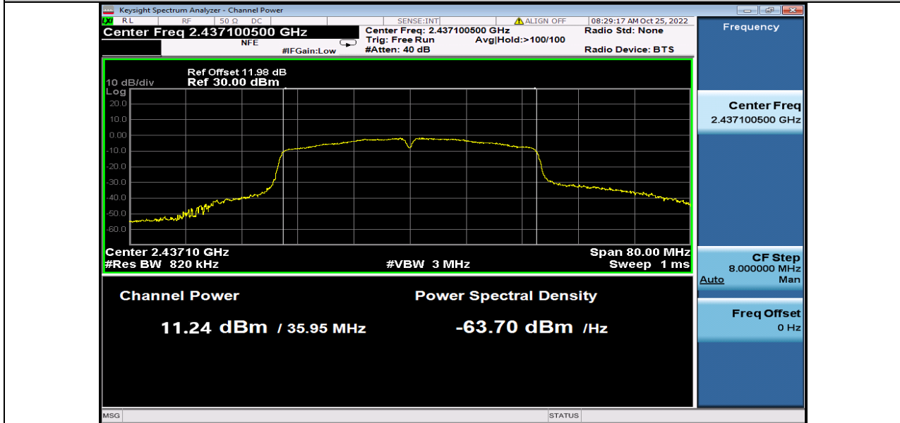
11N40SISO_Ant1_2437
