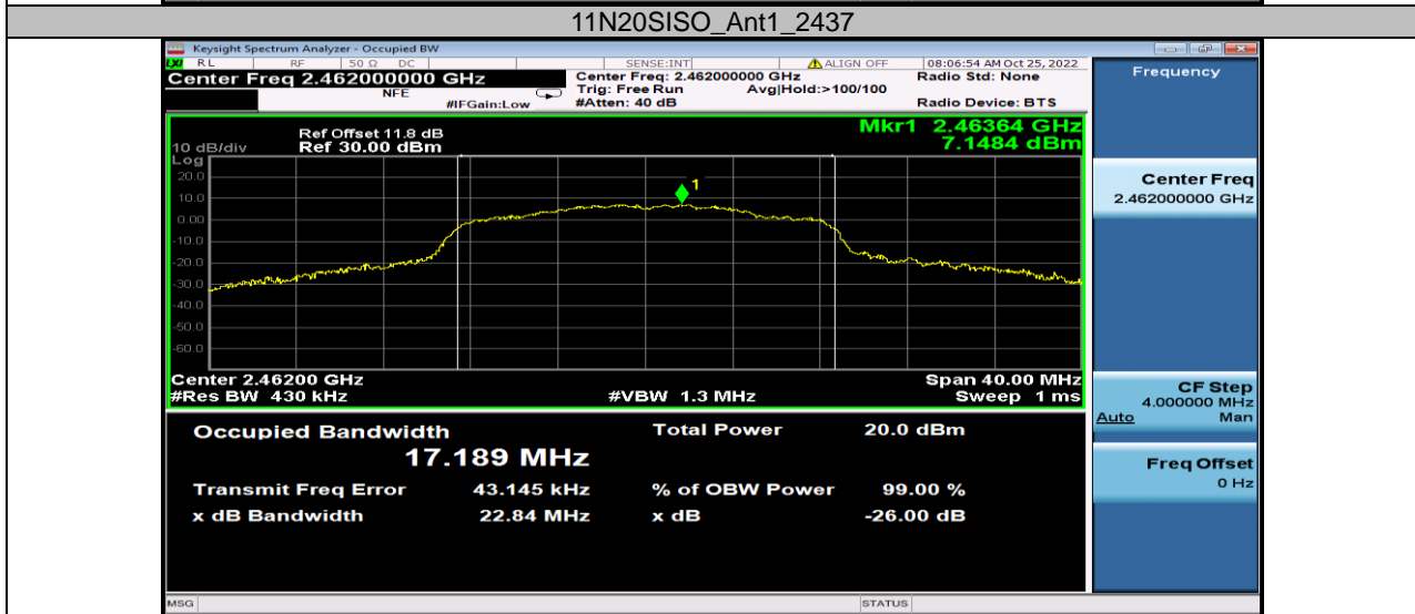
11N20SISO_Ant1_2462
