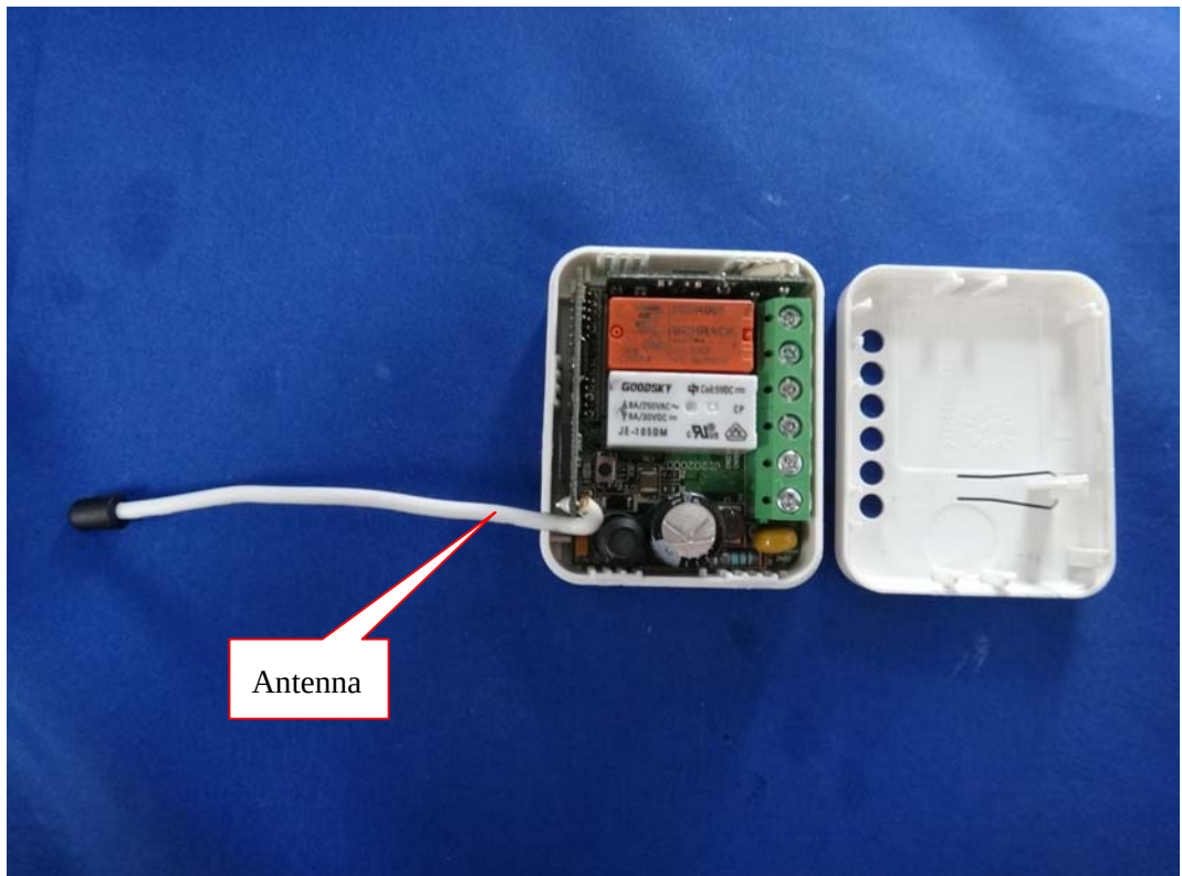
(4) EUT Photo
