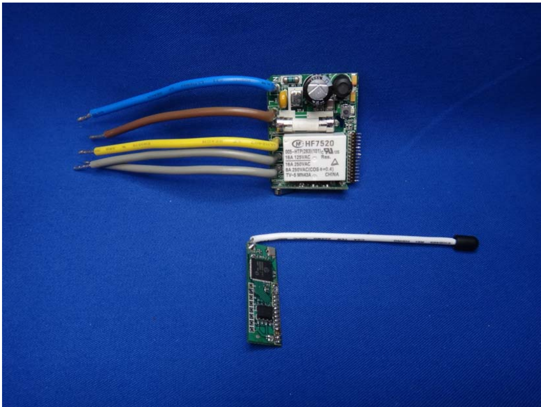
(8) EUT Photo (Z-Wave Module)
